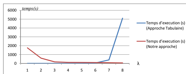
FIGURE 3.6 – Temps d'exécution des algorithmes en fonction du poids de pondération \lambda
