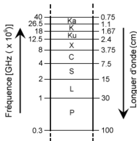
Figure 1-1 : Bandes de fréquence utilisées en télédétection (source : Centre canadien de télédétection).
