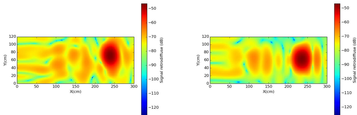
Figure 4-11 : Reconstruction d'image radar entre 1 et 2 GHz à partir de l'algorithme présenté chapitre 2. À gauche, image sur le bac de sable après un déversement de 40L de diesel. À droite, image sur le bac de terre après un déversement de 10L de diesel. La tache rouge situé à 2.5m sur les deux images correspond au trièdre.
