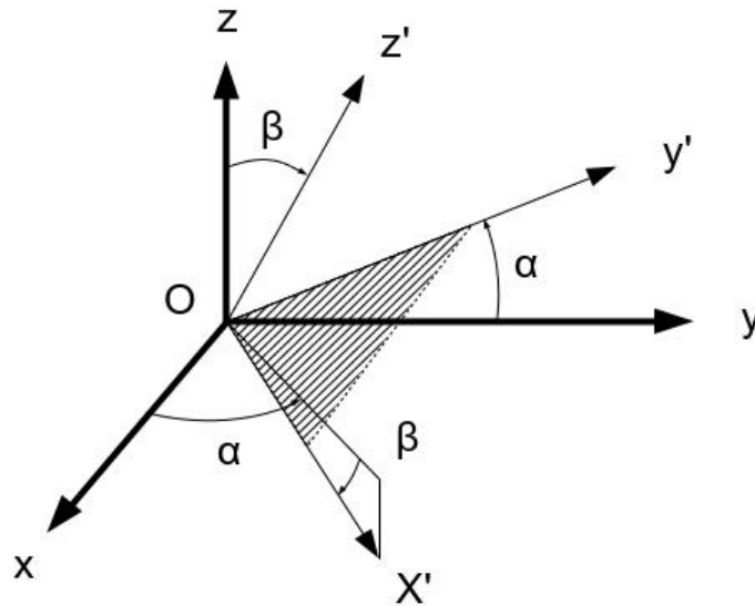
Figure 2-7 : Repère global (O, \vec{x}, \vec{y}, \vec{z}) et repère local du triangle (O', \vec{x}', \vec{y}', \vec{z}') . Le repère du triangle est orienté par l'angle polaire \beta et l'angle azimutal \alpha par rapport au repère de référence.
