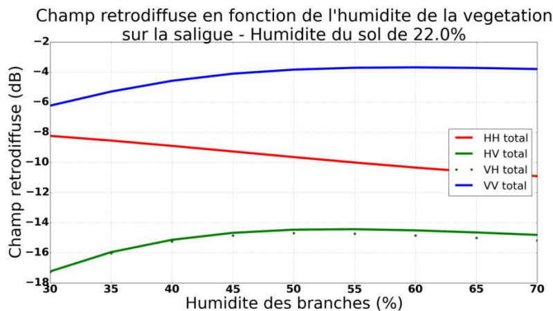
Figure 4-27 : Évolution de la rétrodiffusion en fonction de l'humidité de la végétation sur la saligue. L'humidité du sol reste constante. Simulation du mois de juin.
