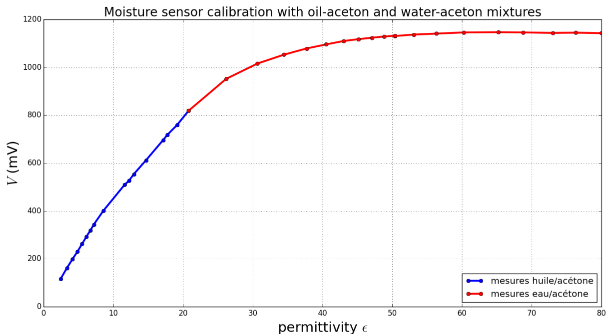
Figure 2-35 : Calibration de la sonde d'humidité : relation entre la tension lue sur la sonde et la permittivité du mélange. On note le bon raccordement entre les séries de mesures huile/acétone et eau/acétone qui conforte nos mesures.
