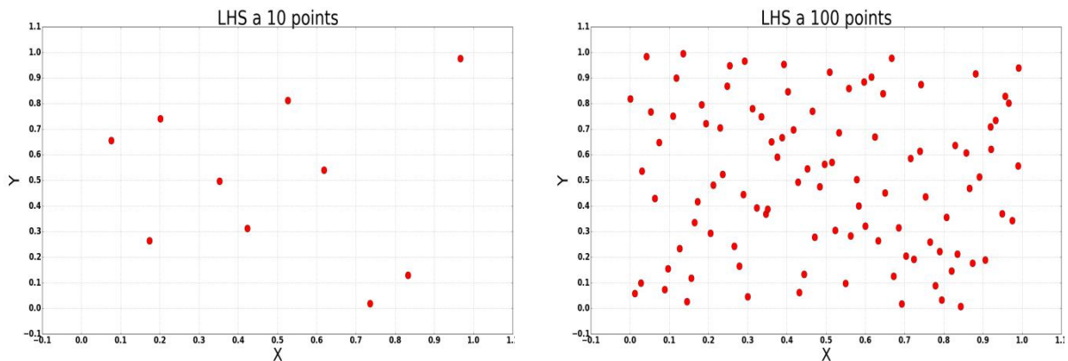
Figure 5-4 : LHS dans \mathbb{R}^2 à 10 points (à gauche) et 100 points (à droite).
