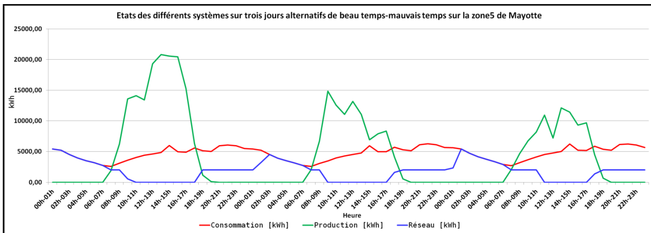
Figure 4.53 : États des différents systèmes sur 3 jours sur la zone 5 [Limite haute = 30 000 kWh]
