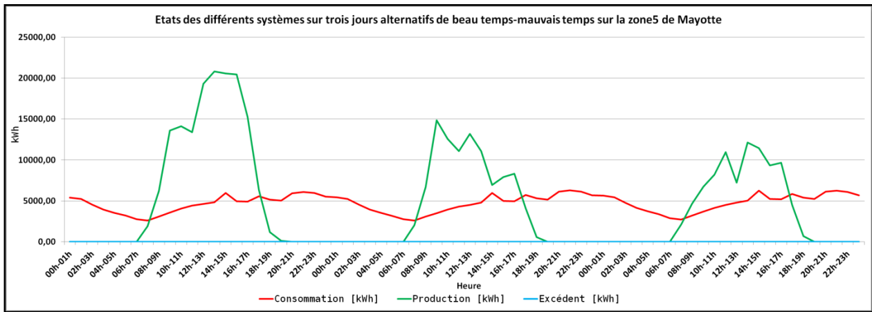
Figure 4.51 : États des différents systèmes sur 3 jours alternatifs de beau-temps et mauvais-temps sur la zone 5 avec une capacité de stockage de 113 660 kWh [kWh]
