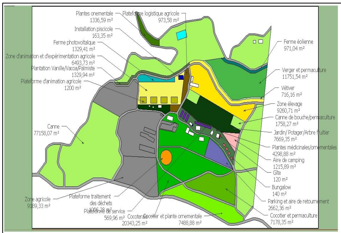
Figure 3.9 : Schéma directeur Eco Ferme de Vincendo avec ces différents espaces Auteur : C.Hoarau
