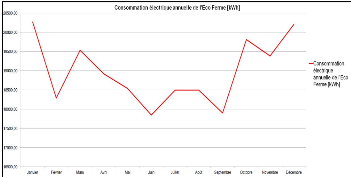
Figure 3.28 : Résultat de la consommation électrique annuelle de l'Eco Ferme [kWh]
