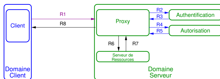
FIGURE 5.6 – Modèle d'une architecture basée sur OSCORE.
