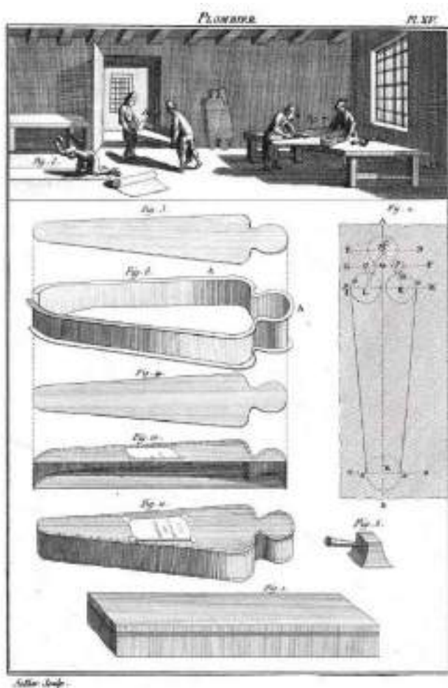
Figure 87 : Mode opératoire de la fabrication des cercueils en plomb au XVIII e siècle (Bertrand 1780, pl. XV)
