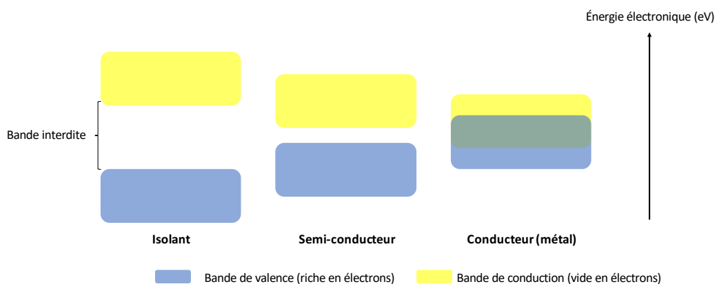
Figure 3. Représentation schématique illustrant la théorie des bandes pour des matériaux isolants, semi-conducteurs et conducteurs.
