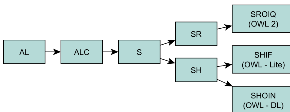
FIGURE 2.4 – Familles de logiques descriptives
