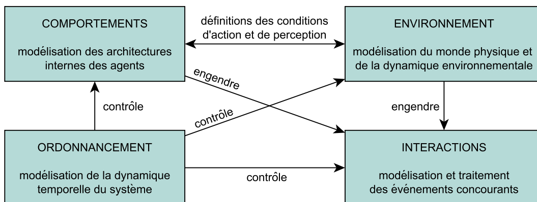
FIGURE 2.1 – Les quatre aspects d'un modèle de simulation multi-agents Michel [2004]
