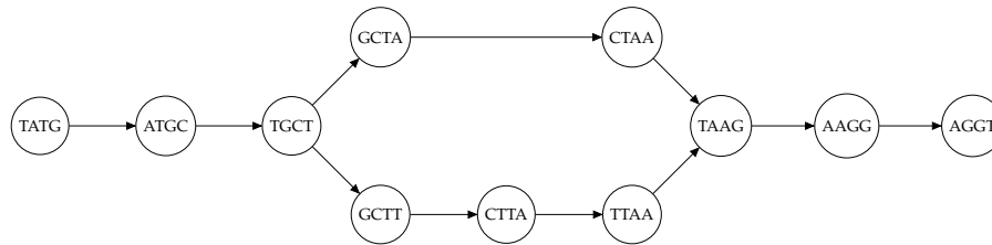
FIGURE 2.17 – Graph de de Bruijn d'ordre 4 de l'ensemble de séquences S = \{\text{TATGCT}, \text{TGCTAA}, \text{GCTTAA}, \text{TAAGGT}\} . Afin de simplifier le graphe, les séquences complémentaires inverses des k -mers ne sont pas considérées ici.
