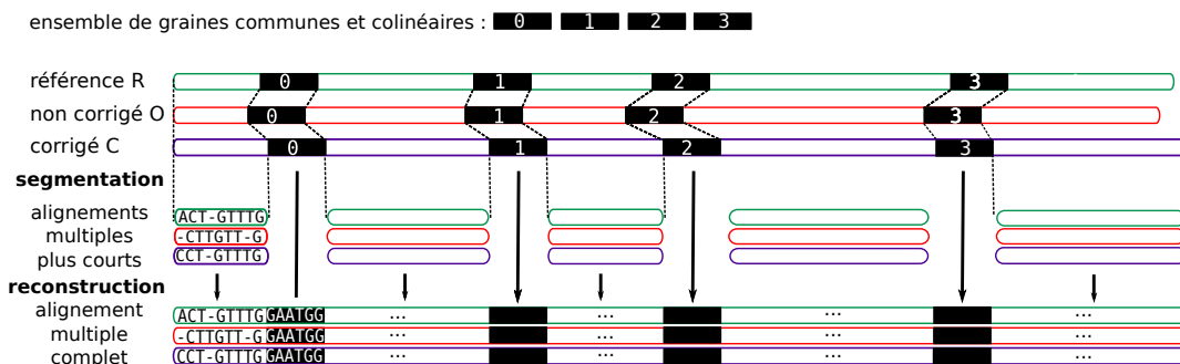
FIGURE 4.4 – Stratégie de segmentation pour l’alignement multiple d’un triplet représentant la version de référence, la version non corrigée, et la version corrigée d’un même read. Plutôt que de calculer un alignement multiple sur toute la longueur des trois séquences, le problème est divisé en de plus petits alignements multiples indépendants. Puisque chaque version du read est différente, des k -mers communs (en noir) aux trois séquences, et définissant des matches exacts locaux, sont utilisés comme graines afin de déterminer la façon dont l’alignement multiple peut être divisé. Des alignements multiples locaux et indépendants sont alors calculés pour les facteurs des séquences bordés par des graines, ainsi que pour leurs préfixes et pour leurs suffixes. Les alignements multiples des fenêtres ainsi définies, et les k -mers ayant servi de graines, sont ensuite concaténés, afin d’obtenir un alignement multiple unique, sur toute la longueur des séquences.
