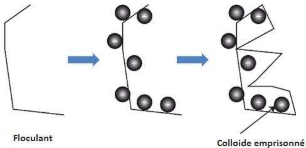
Figure 6 : Flocculation par emprisonnement (balayage ou sweep) (Tardat et al., 2000)
