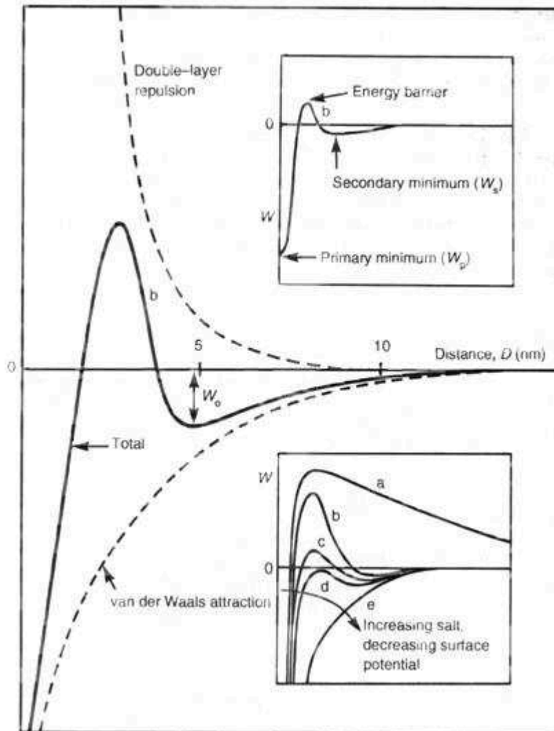
Figure 2 : Energie d'interaction entre les particules en fonction de la distance interparticulaire (Israelachvili 2011).
