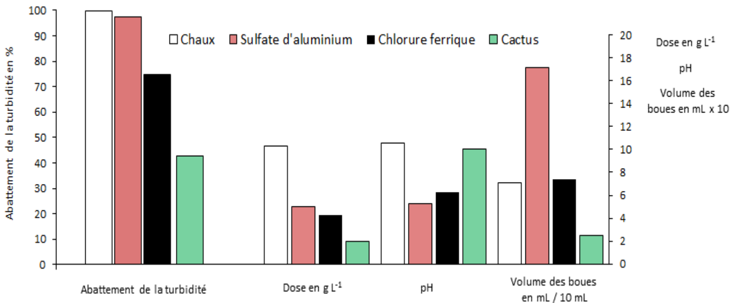
Figure 23 : Comparaison de l'efficacité de traitement en fonction du type de coagulant
