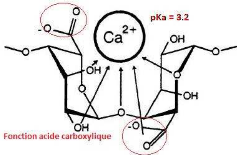
Figure 11 : Structure chimique d'un gel formé par l'alginate de sodium et les ions de calcium (Huang et al., 1999)
