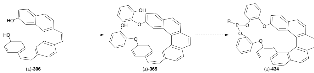
Schéma 123 : Structure hélicoïdale cyclique envisagée
