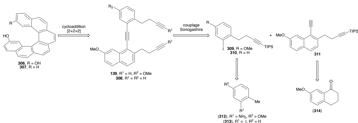
Figure 19 : Analyse rétrosynthétique
