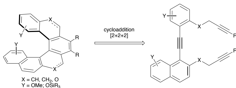
Figure 18 : Voie de synthèse par [2+2+2]
