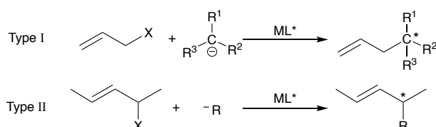
Figure 42 : Les deux types d'alkylation allylique asymétrique
