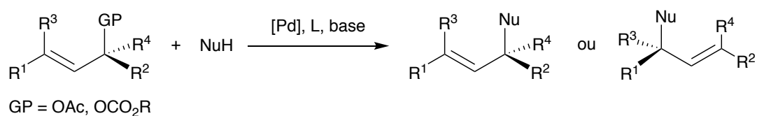
Schéma 110 : Bilan de l'alkylation allylique catalysée au palladium
