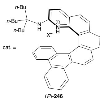
Schéma 66 : Réaction de Diels-Alder énantiosélective
