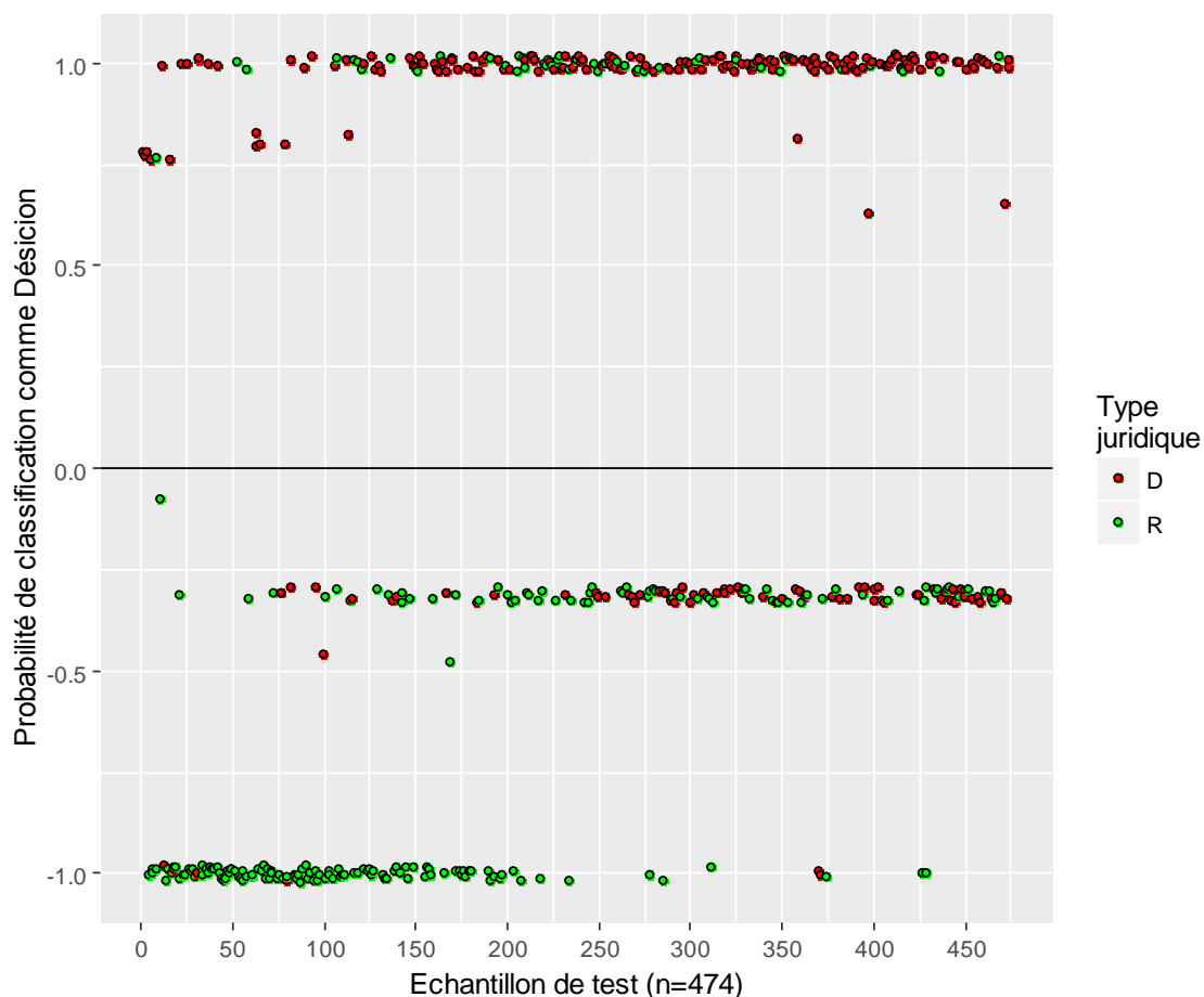
Figure 68 : probabilités du modèle RF basé sur l'existence des mots étiquette
