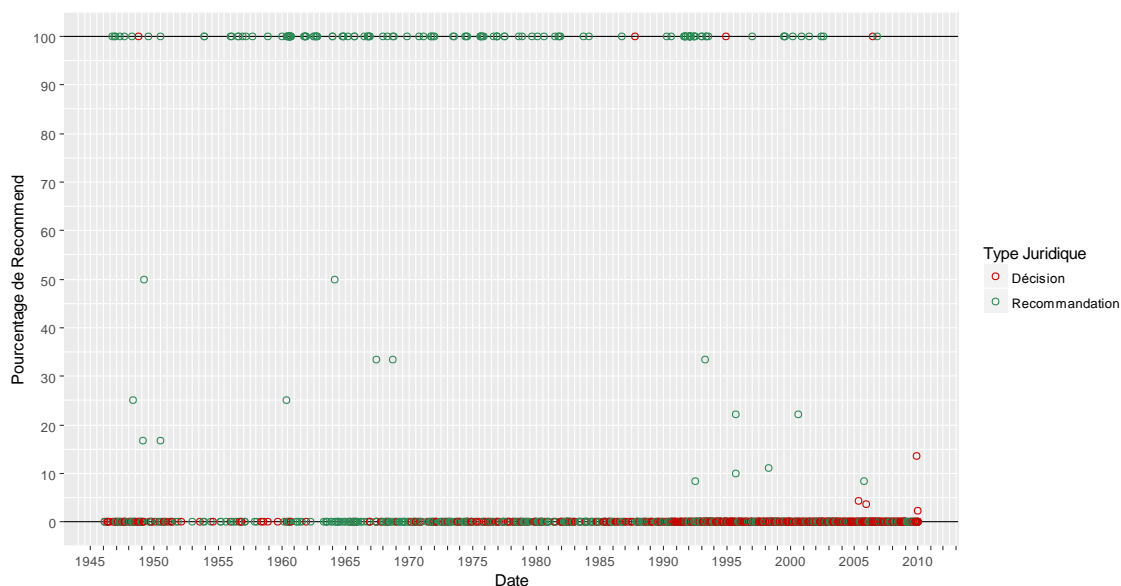
Figure 63 : pourcentage de Recommend jusqu'à la resolution 1907 (2009) par type juridique
