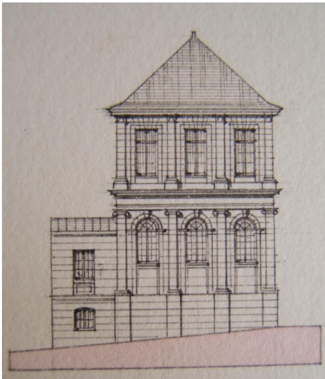
Façade latérale et plan de coupe du pavillon central du palais universitaire
