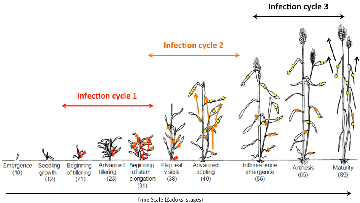
Figure 6 : schéma simplifié du déroulement d'épidémies polycycliques de Rouille du blé
