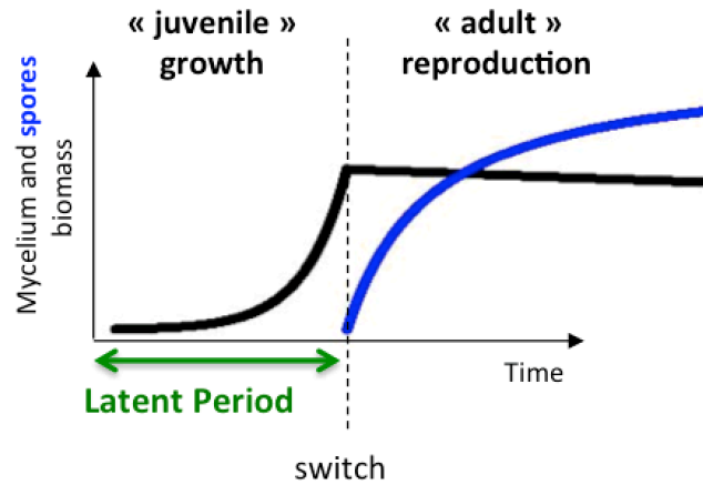
Figure 5 : simplification du cycle infectieux de la rouille du blé telle qu'utilisée dans nos modèles.
