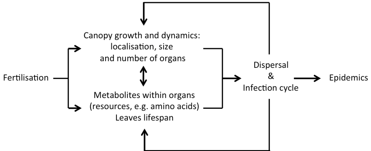
Figure 7 : résultat de notre synthèse bibliographique sur l'impact de la fertilisation sur le pathosystème.
