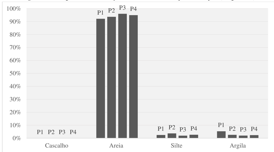
Figura 18: Histograma da Distribuição Granulométrica - Frequência Simples (Alegrete/RS)
