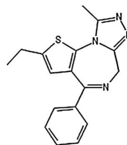
Figure 14. Structure chimique du deschloroétizolam
