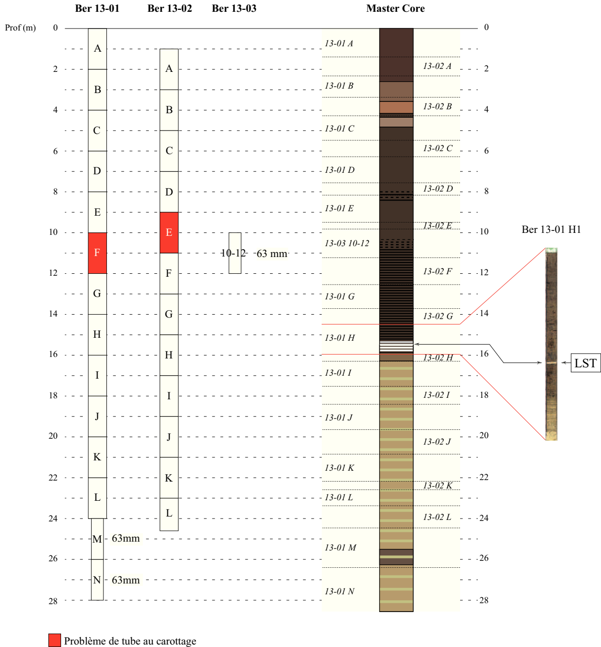
FIGURE 2.5 – Représentations schématiques du carottage du Bergsee (2013) et de la stratigraphie (explication des dessins en figure suivante) de la séquence composite finale. La section BER 13-01 H1 est ajoutée, le téphra du Laasher See - LST - indiqué.
