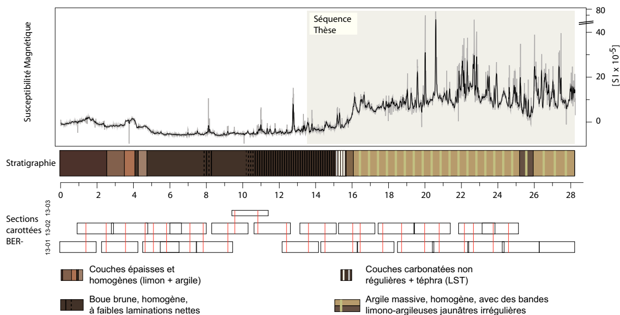
FIGURE 2.7 – Evolution de la susceptibilité magnétique - SM - et stratigraphie de la séquence composite (i.e. Master Core). Bas : schéma de la compilation des différentes sections pour la construction de la Master Core. La séquence utilisée dans cette thèse est indiquée par un encadré gris.
