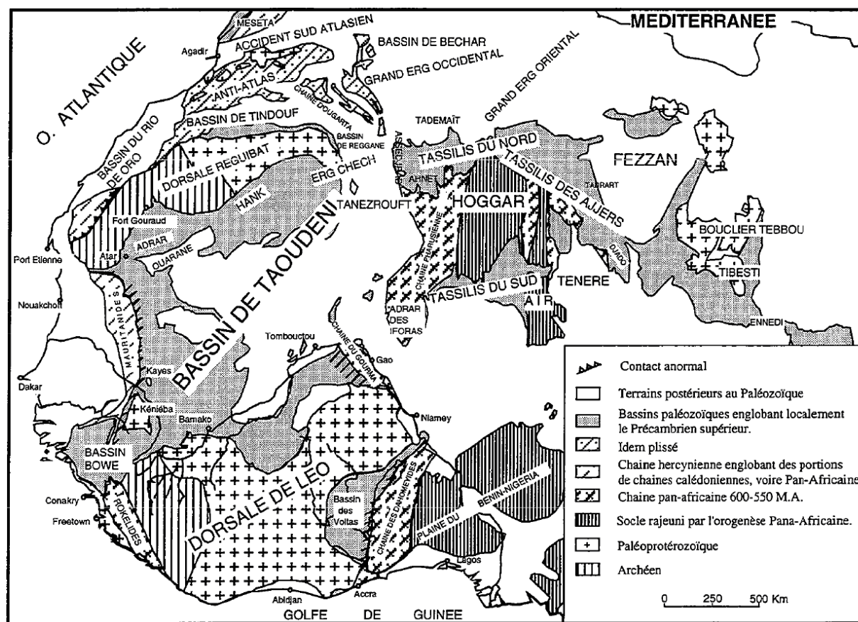
FIGURE 3.1 : Carte géologique de l'Afrique de l'Ouest. D'après Trompette (1973).
