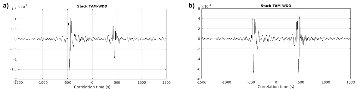
FIGURE 4.4 : Inter-corrélations de la paire de station TAM-WDD : a) corrélation sommée sur l'année 2011 et b) corrélation sommée de 2003 à 2014. On voit que les amplitudes des formes d'ondes sont plus stables et avec une meilleure symétrie dans les corrélations sur une longue période des temps.
