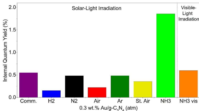
Figure 4. Rendement quantique interne (IQY,%) des composites tels que préparés sous irradiation solaire et visible.
