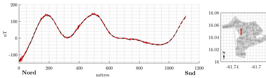
FIGURE 4.38 – Comparaison d'un profil extrait de la grille calculée par l'algorithme gridfit et du profil correspondant de l'anomalie magnétique. La localisation du profil en question au sein des routes du drone est donnée par la figure sur la droite.
