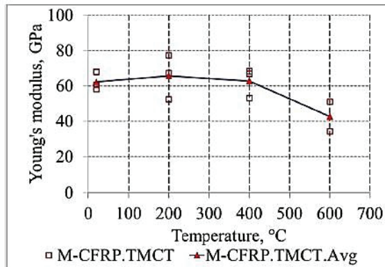
(c) Evolution du module d'Young ultime en fonction de la température
