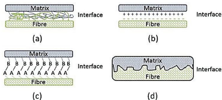
Figure 1. 3 : Mécanisme d'adhérence entre fibre et matrice à l'interface : (a) par enchevêtrement moléculaire ; (b) par attraction électrostatique ; (c) par réaction chimique ; (d) par inter-diffusion d'éléments
