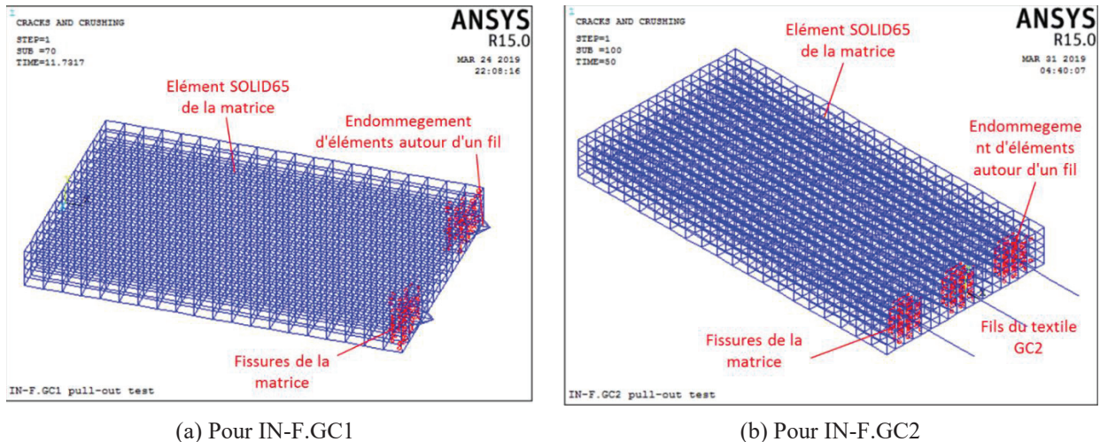
Figure 4. 20 : Mode de rupture des éprouvettes d'arrachement dans le modèle numérique
