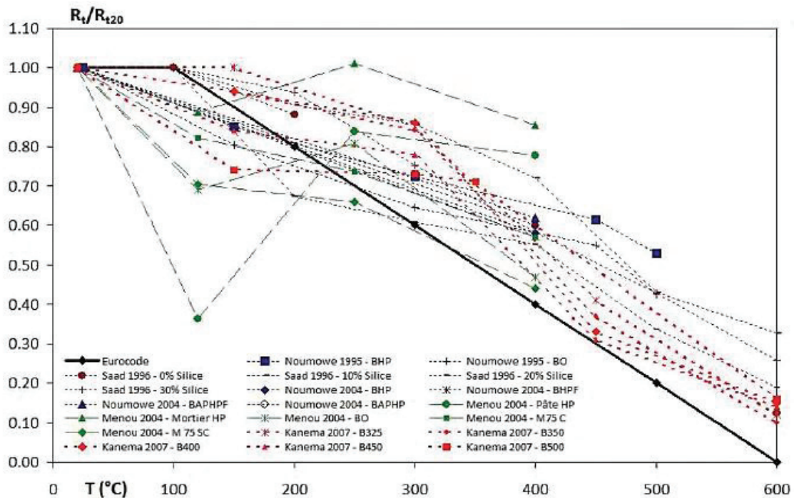
Figure 1. 21: Différents résultats concernant l'évolution de la résistance de matrice de béton en traction en fonction de la température, reportés par Fares [55]
