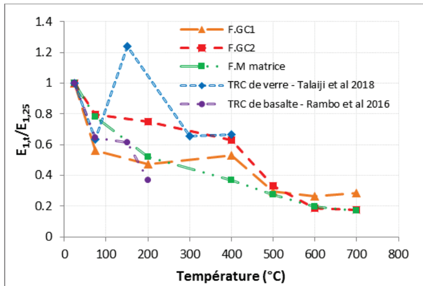
Figure 3. 16: Evolution du module d'Young normalisé à la première phase dépendant de la température, en comparant avec les résultats expérimentaux sur le TRC de basalte obtenu par Rambo et al [32] et le TRC de verre obtenu par Talaji et al [35]
