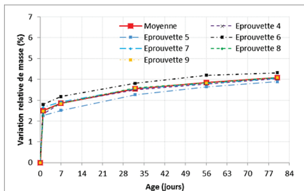
Figure 2. 8 : Cinétique de saturation dans l'eau de l'éprouvette de matrice réfractaire
