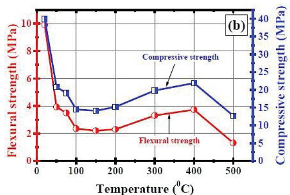
Figure 1. 23 : Evolution de la résistance ultime (en flexion et compression) du béton en fonction de la température [70]
