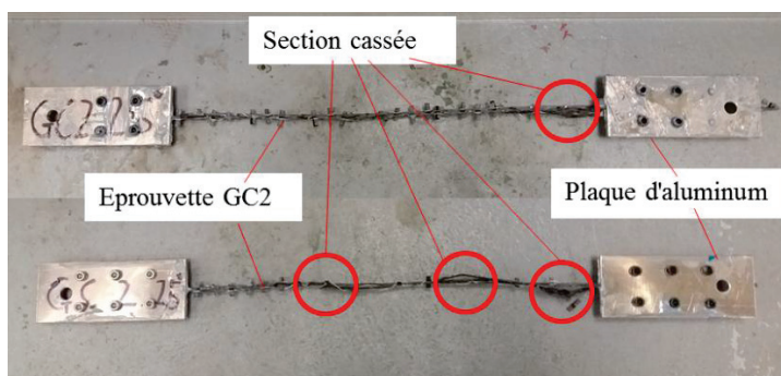
GC2: Mode de rupture à température ambiante
