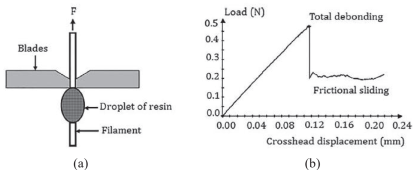
Figure 1. 28 : Schéma de principe du test des microgouttelettes (a), courbe « force – déplacement » typique (b), Selon Baley et al [85]
