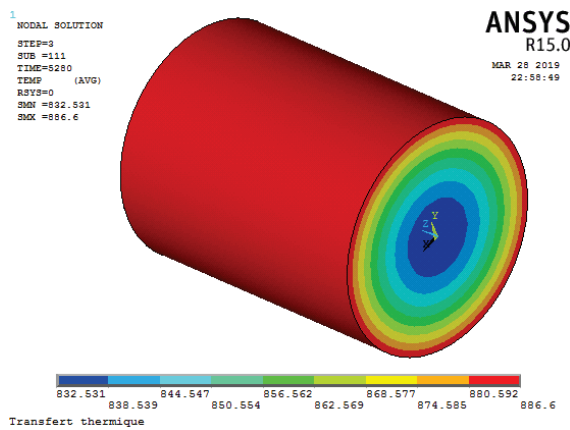
(a) Température sur l'éprouvette après 40 minutes de calcul
