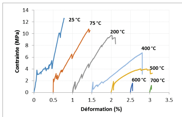
Figure 3. 10: Comportement thermomécanique du composite F.GC1 à différentes température
