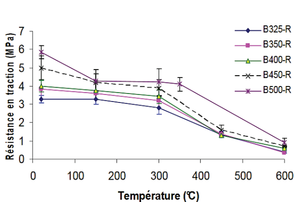
Figure 1. 22 : Evolution de la résistance résiduelle en traction en fonction de la température [58]
