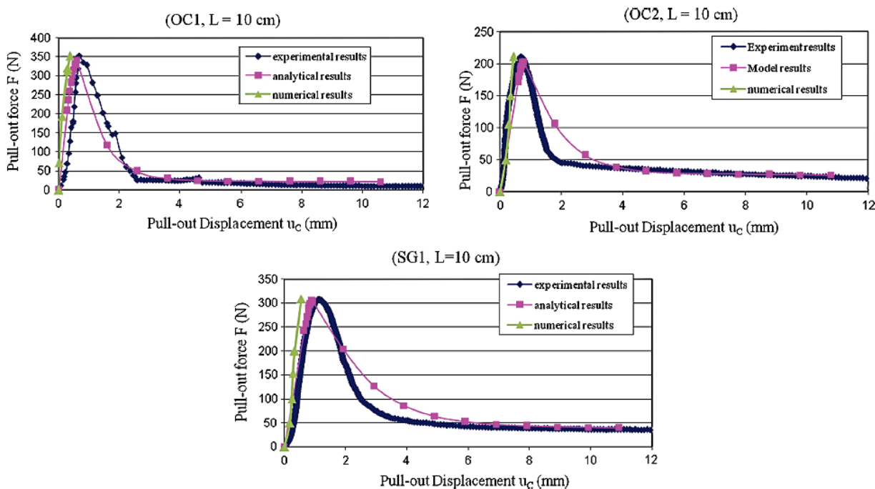
Figure 1. 69 : Comparaison des résultats expérimental, analytique et numérique, selon Zhang et al 2013 [86]
