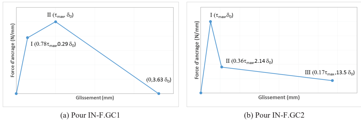
Figure 4. 13 : Relation « force – glissement » d'élément COMBIN 39 pour la liaison « fil – matrice » dans le modèle numérique
