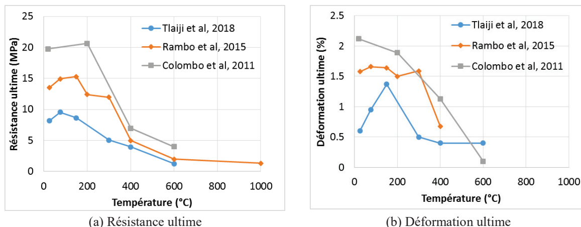
Figure 1. 48 : Evolution des propriétés résiduelles du composite en fonction de la température, (a) résistance ultime, (b) déformation ultime
