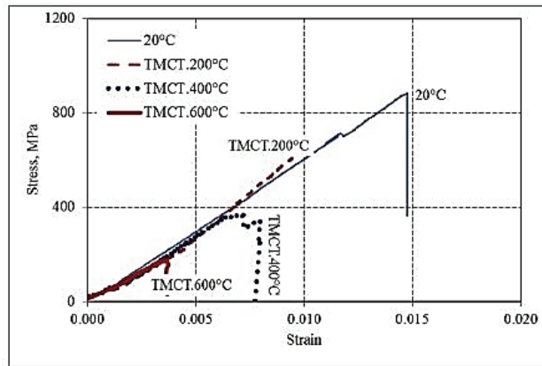
(a) Courbes « contrainte – déformation » à différentes températures
