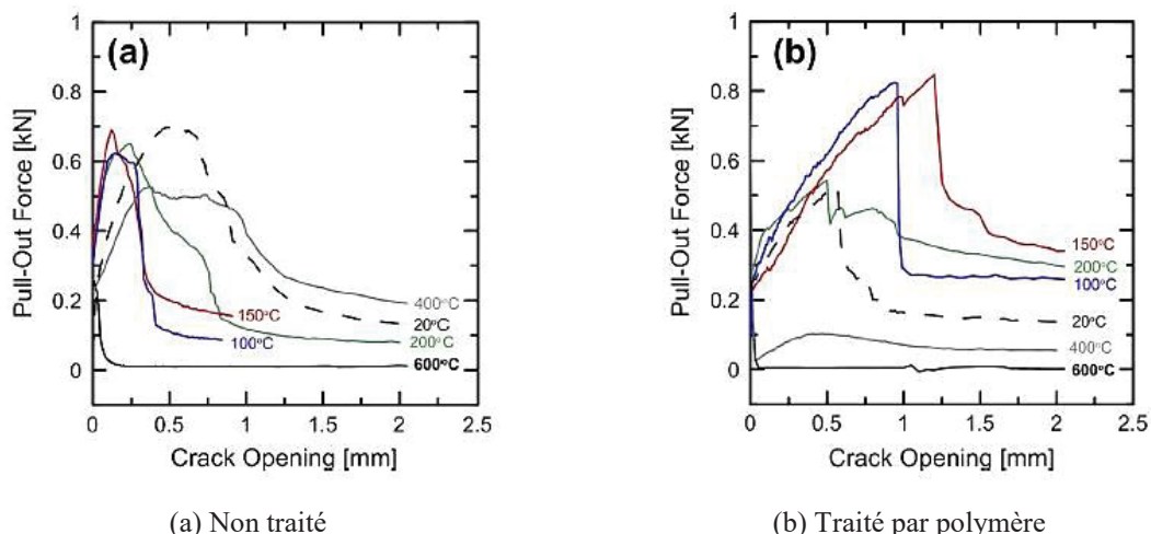
Figure 1. 31 : Influence du traitement de fibre sur le comportement de l'interface ; non traité (a) et traité par polymère, Selon Silva et al [43]
