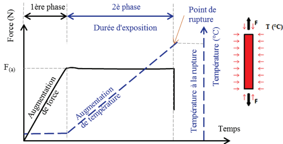
Figure 3. 4: Schéma de chargement des essais thermomécaniques au régime TMFC
