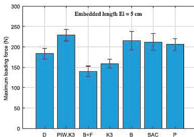
Figure 1. 39 : Evolution de la force maximale en fonction des configurations étudiées (avec la longueur d'ancrage 5 cm), selon Homoro et al [89]
