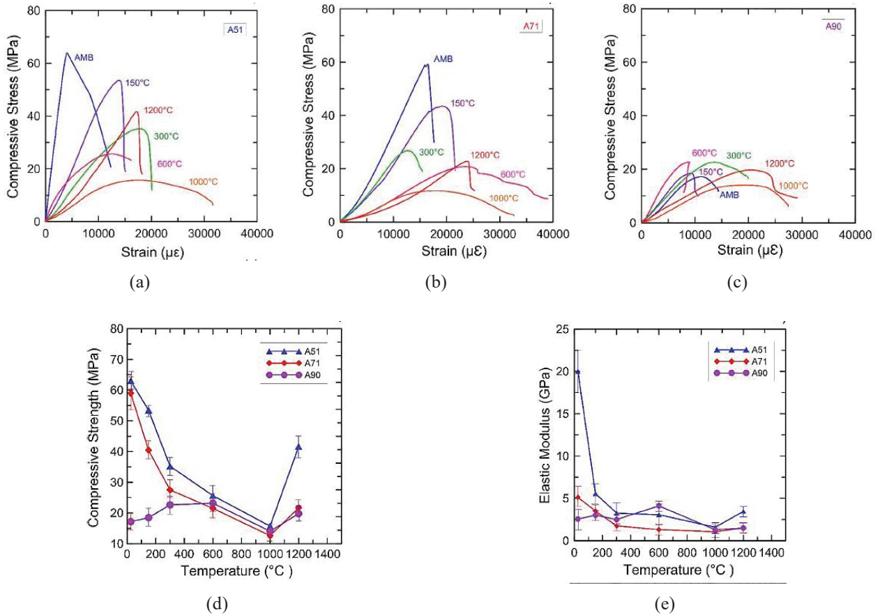
Figure 1. 24: Résultats résiduelles sur les éprouvettes du béton réfractaire à hautes température ; (a)(b)(c) Comportement en compression pour trois niveaux de teneur en alumine ; Evolution des propriétés en compression avec la température : (d)résistance ultime, (e) module d'Young. [23]
