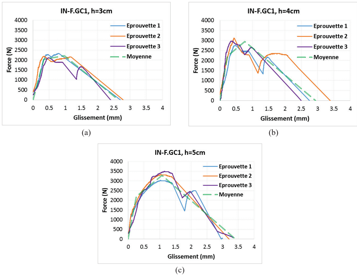
Figure 2. 36 : Courbes « force – glissement » de l'interface textile GC1/matrice cimentaire avec différentes longueurs d'ancrage
