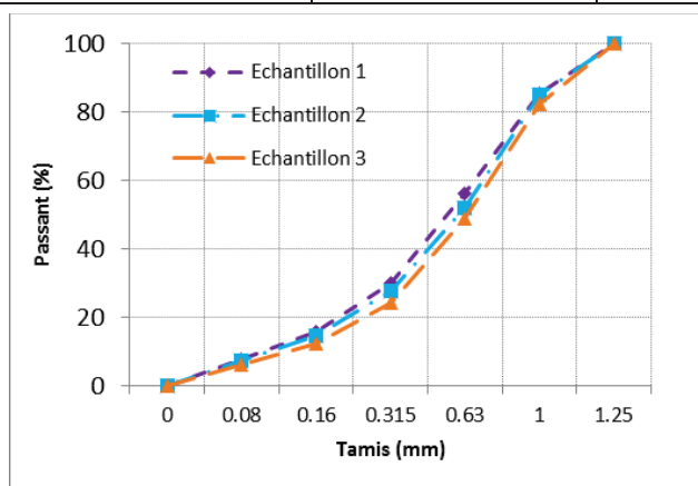
Figure 2. 4 : Courbes granulométriques d'agrégats synthétiques silico-alumineux-calciques
