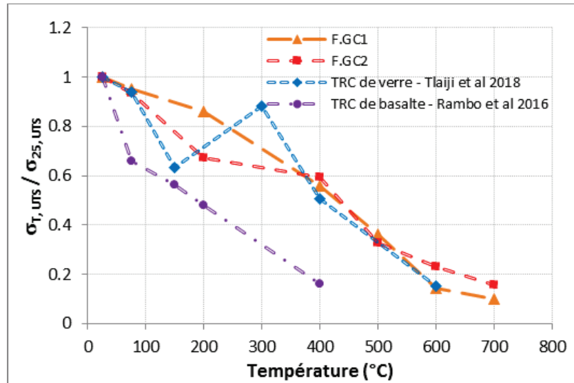
Figure 3. 14: Évolution de la contrainte ultime normalisée obtenue pour les composites F.GC1 et F.GC2, en comparant avec les résultats expérimentaux sur le TRC de basalte obtenus par Rambo et al [32] et sur le TRC de verre obtenu par Tlaji et al [35]
