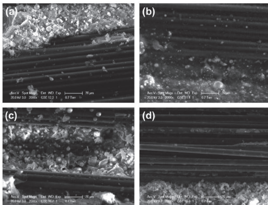
Figure 1. 34 : Interface matrice-fibre de carbone revêtue: (a) dans son état naturel et (b) après exposition à des températures de (b) 150 °C, (c) de 200 °C et (d) de 400 °C, Selon Silva et al [43]
