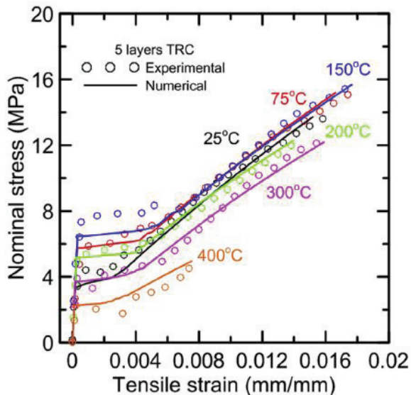
(a) Comportement de TRC à différentes températures
