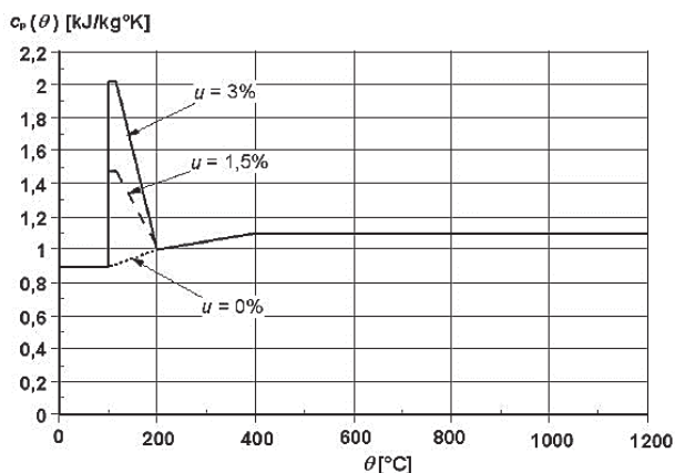
(a) Chaleur spécifique, C_p(\theta) , en fonction de la température pour 3 teneurs en eau différentes ( u ): 0 %, 1,5 % et 3 % du poids de béton
