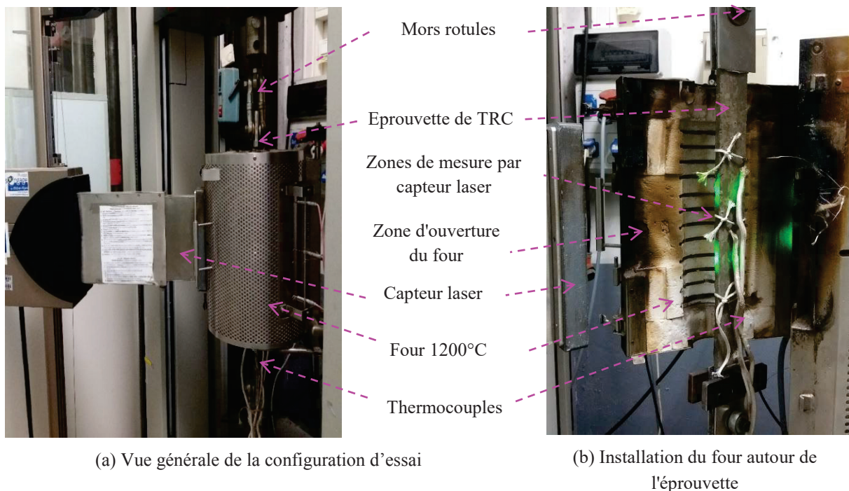
Figure 3. 1: Configuration d'essai thermomécanique sur l'éprouvette de TRC
