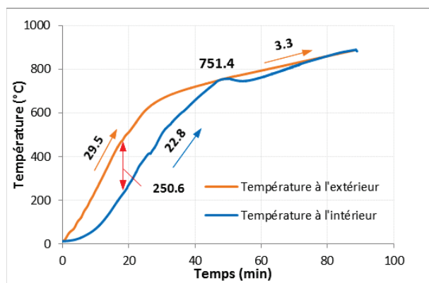
Figure 2. 32 : Augmentation de la température à l'extérieur et à l'intérieur de l'éprouvette cylindrique
