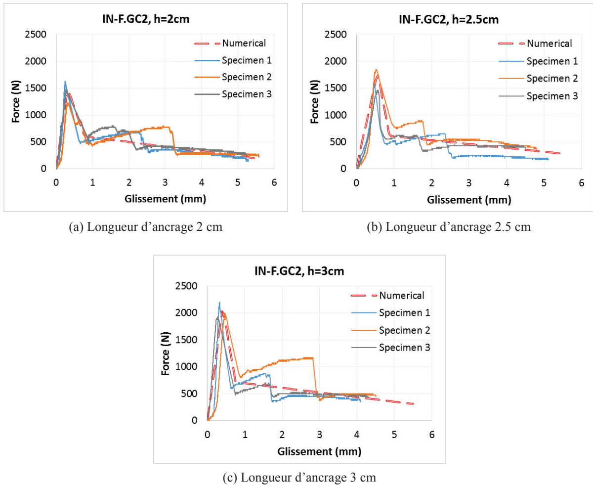
Figure 4. 19 : Comparaison des résultats expérimentaux et numériques sur le comportement d'arrachement des éprouvettes d'IN-F.GC2
