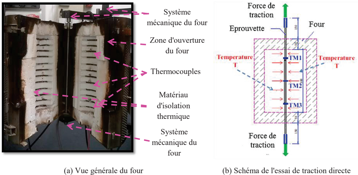
Figure 2. 10: Détail du four pour l'essai thermomécanique sur TRC
