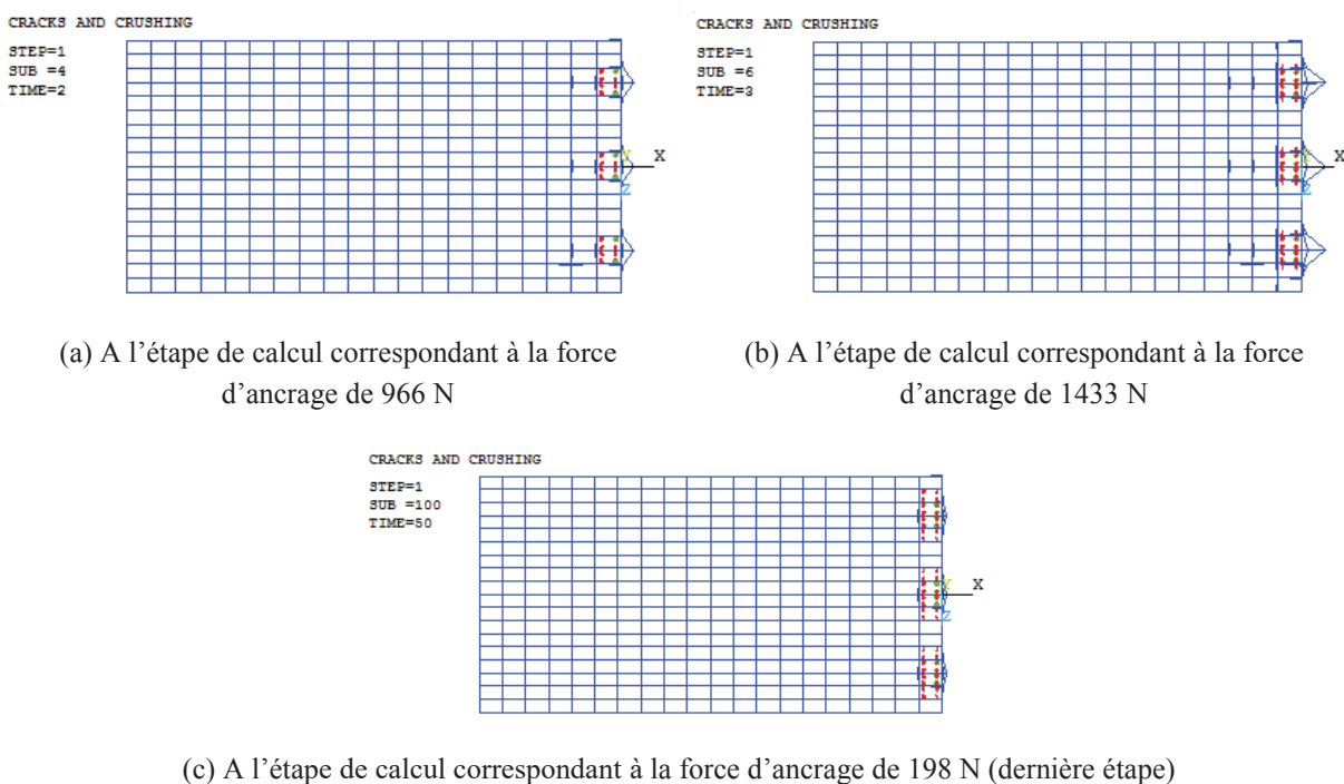
Figure 4. 23 : Elargissement des fissures avec l'augmentation de la force d'ancrage pour IN-F.GC2-2cm
