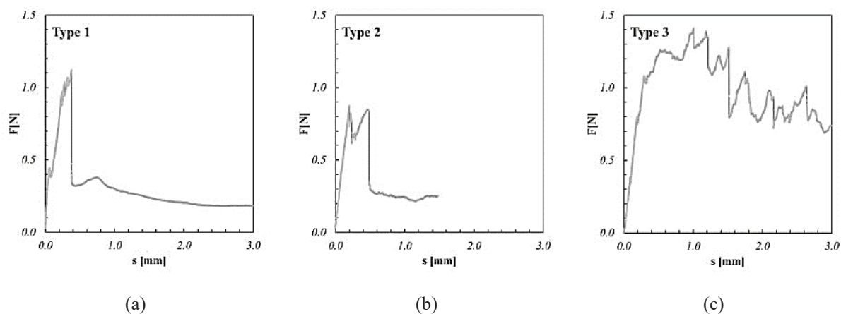
Figure 1. 30 : Trois types de réponses de l'interface entre fibre de jute et matrice cimentaire ; Selon Ferreira et al [88]
