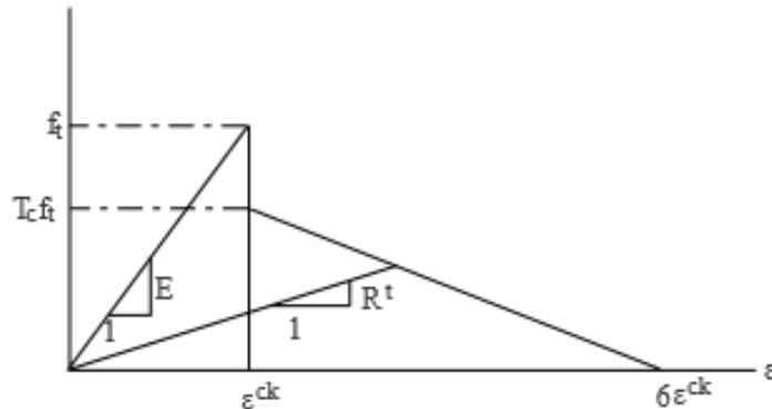
Figure 4. 8: Loi du comportement mécanique de la matrice
