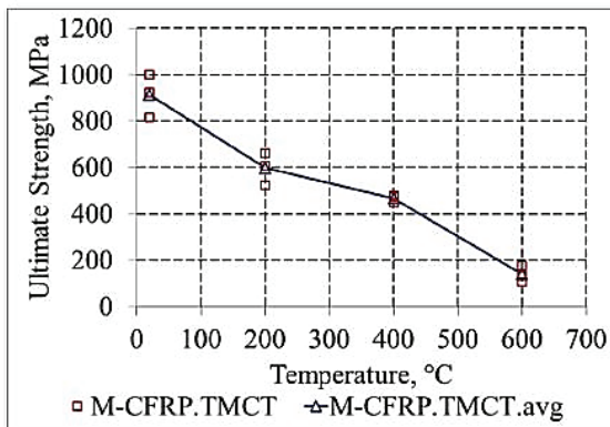
(b) Evolution de la résistance ultime en fonction de la température
