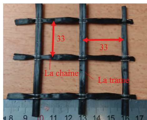
(b) Géométrie du textile GC3
