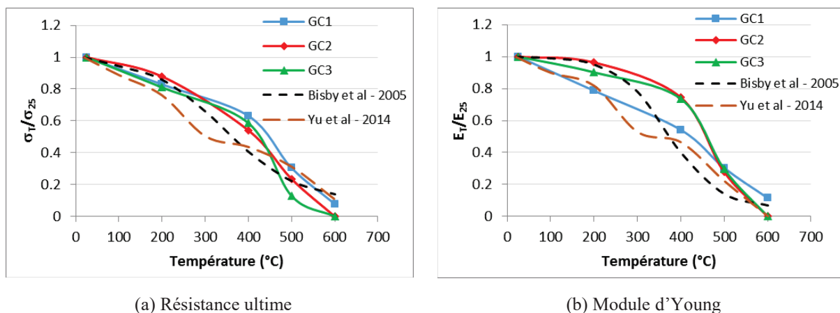
Figure 2. 20: Evolution des propriétés thermomécaniques normalisées obtenues pour les textiles de carbone étudiés en comparant avec les résultats expérimentaux sur les matériaux composites CFRP obtenus par Bisby et al. 2005 [47], par Yu et al [150]
