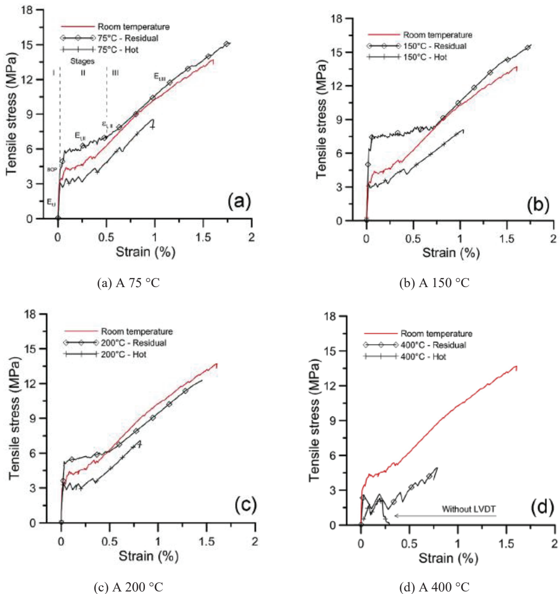
Figure 1.52 : Comparaison des comportements résiduel et thermomécanique du composite TRC de basalte à différentes températures, Rambo et al [32]
