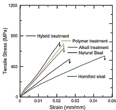
(a) fibre de sisal avec différents traitements, Ferreira et al [39]
