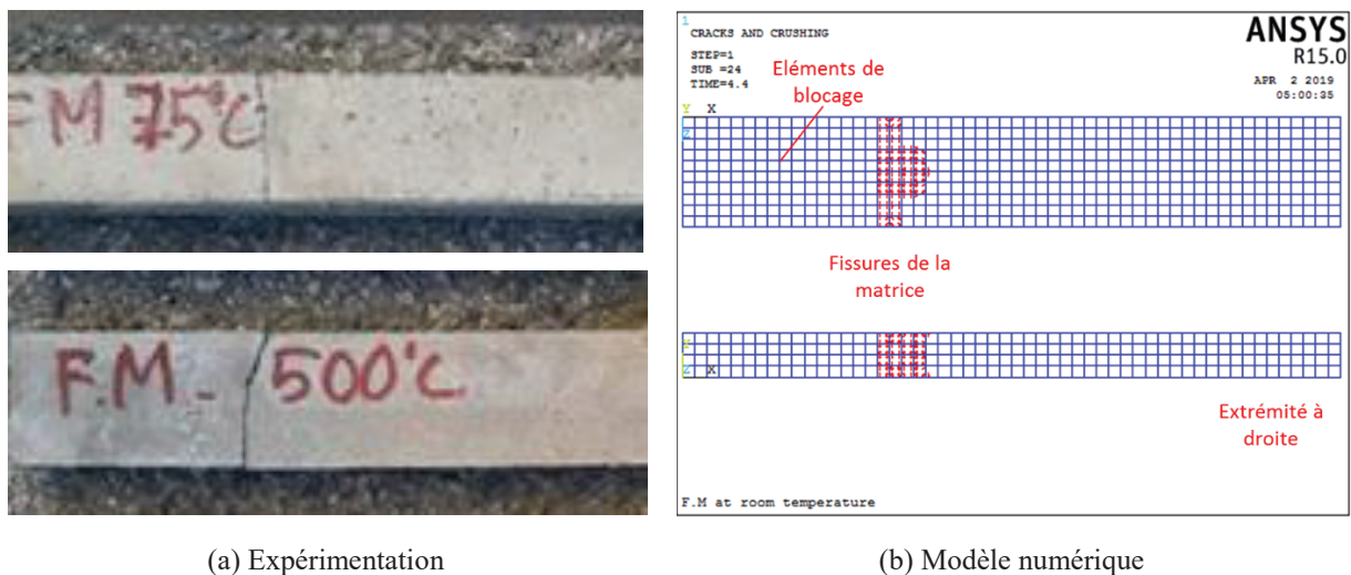
Figure 4. 11 : Fissuration sur l'éprouvette dans l'expérimentation et le modèle numérique 3D pour la matrice cimentaire
