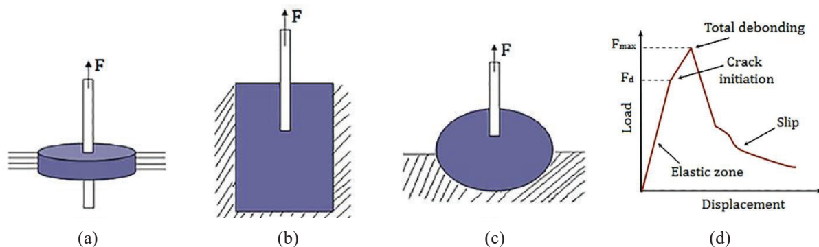
Figure 1. 27 : Différentes configurations de test d'arrachement: (a) Selon Favre [81] (b) Selon Piggott et al [80] (c) Selon Pitkethly et al [82]; (d) Courbe typique du comportement de l'interface selon Zhandarov et al [84]
