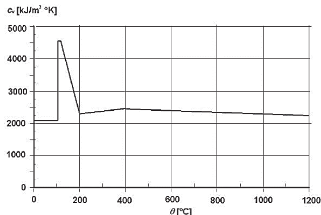
(b) Chaleur spécifique volumique, C_v(\theta) , en fonction de la température pour une teneur en eau, u de 3 % du poids et une masse volumique de 2300 \text{ kg/m}^3 du béton.
