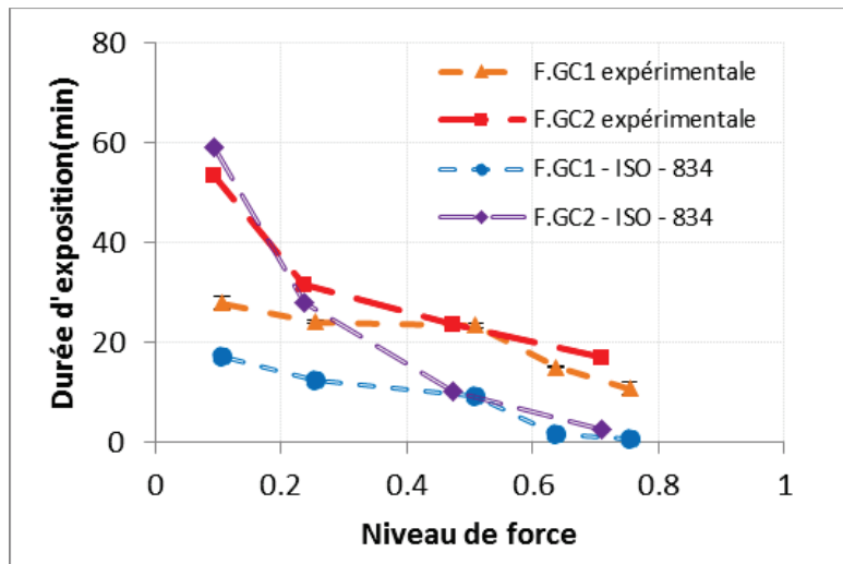
Figure 3. 24: Evolution de la durée d'exposition à température élevée des TRC de carbone en fonction du niveau de force appliqué.
