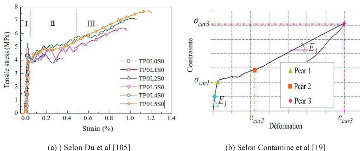
Figure 1. 42: Loi du comportement « contrainte – déformation » du composite TRC
