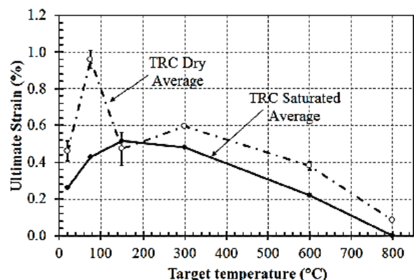
(b) TRC saturé
