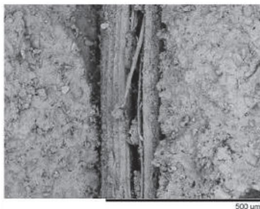
(c) Fibre incorporée dans une matrice à base de ciment
