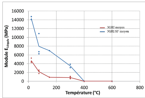
(b) Module d'Young à la première phase
