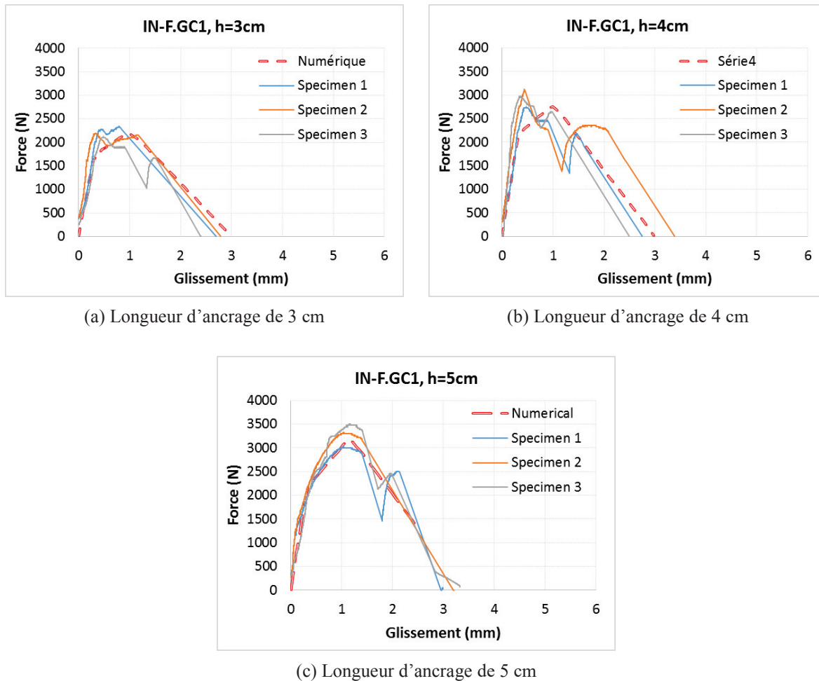
Figure 4. 18 : Comparaison des résultats expérimental et numérique sur le comportement d'arrachement des éprouvettes d'IN-F.GC1
