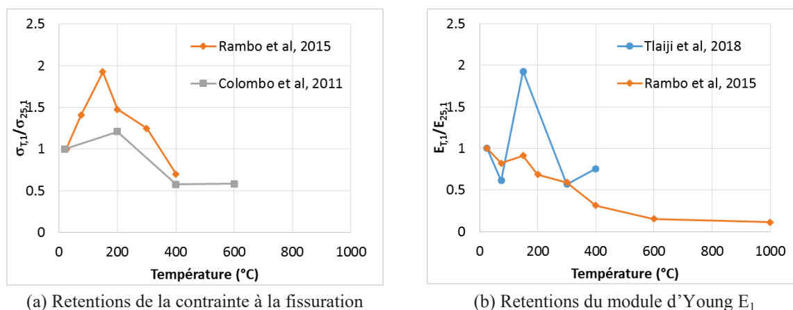
Figure 1. 49 : Evolution des propriétés résiduelles à la première phase en fonction de la température
