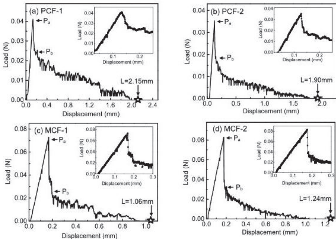
Figure 1. 36 : Courbes « force – déplacement » des fibres de carbone non traité (a,b) et traité par \text{SiO}_2 avec deux différentes méthode (c,d), Selon Lu et al [75]
