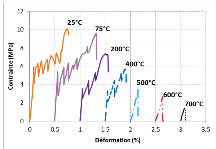
Figure 3. 11 : Comportement thermomécanique des éprouvettes F.GC2: relation contrainte-déformation à différentes températures
