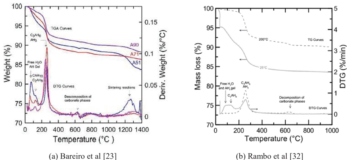
Figure 1. 14 : Résultats des analyses thermogravimétriques et thermogravimétries dérivées pour perte de masse des bétons réfractaires
