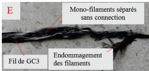
(b) GC3: Zoom de la partie endommagée E
