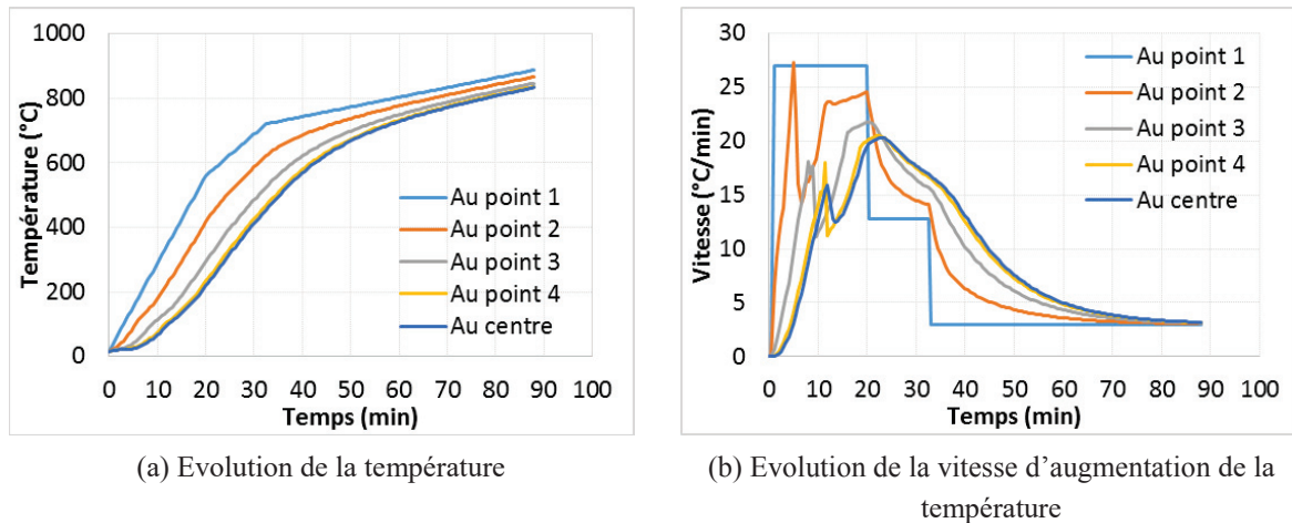
Figure 4. 28 : Evolution de la température et de la vitesse d'augmentation en fonction du temps aux plusieurs points d'éprouvette cylindrique
