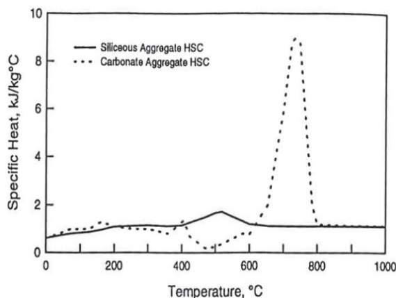
Figure 1. 18 : Influence des granulats sur la chaleur spécifique de béton à température élevée
