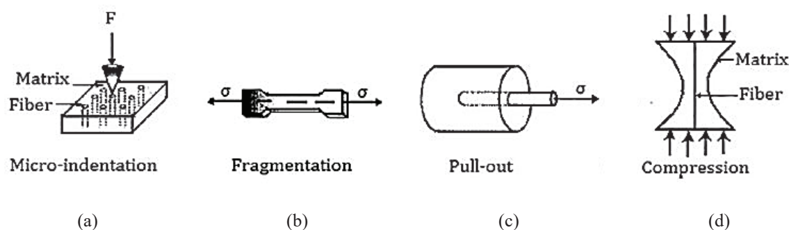
Figure 1. 26 : Certains tests micromécaniques utilisés pour caractériser le comportement de l'interface fibre / matrice ; (a) Micro-indentation ; (b) Fragmentation ; (c) Arrachement ; (d) Compression [Selon Teklal et al [76]]
