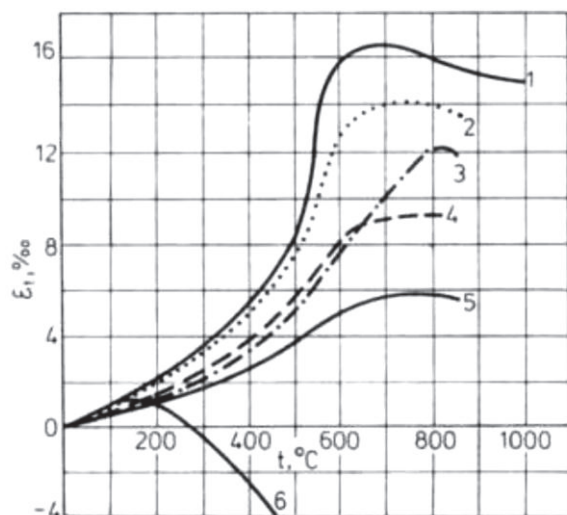
(a) Selon Piasta, reporté par Hager [54] ; 1. siliceux, 2. grès, 3. calcaire, 4. basaltes, 5. argiles expansées, 6. pâte du ciment
