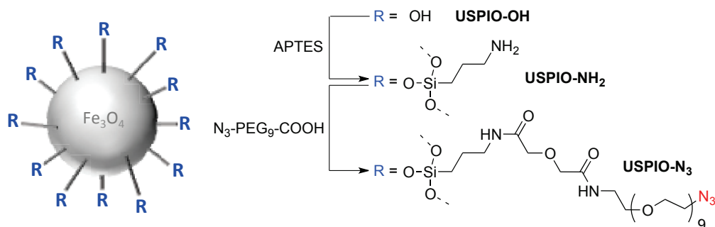
Schéma 75 : Fonctionnalisation multi-étapes de l'USPIO nu pour introduire une fonction azoture
