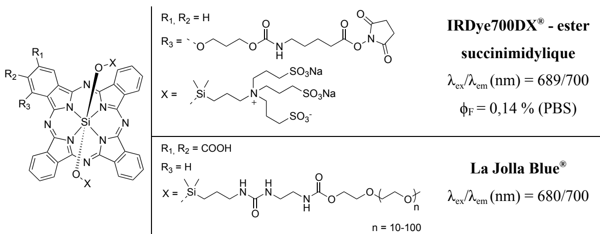
Figure 32 : Structures et propriétés de l'ester activé de l'IRDye700DX ® et de La Jolla Blue ®
