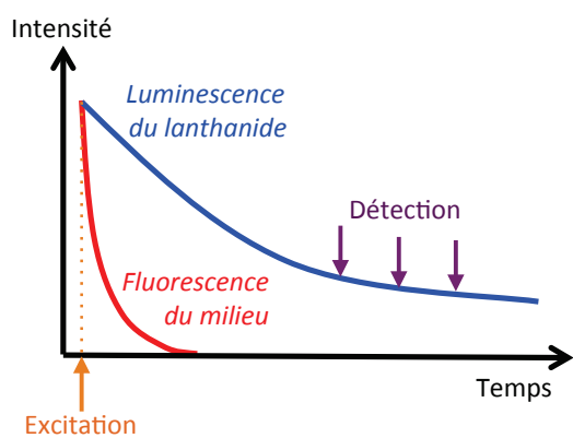
Figure 24 : Détection en temps résolu dans le cas des lanthanides luminescents
