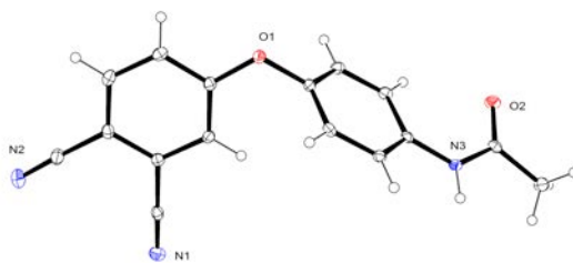
Figure 92 : Structure cristallographique du composé 57
