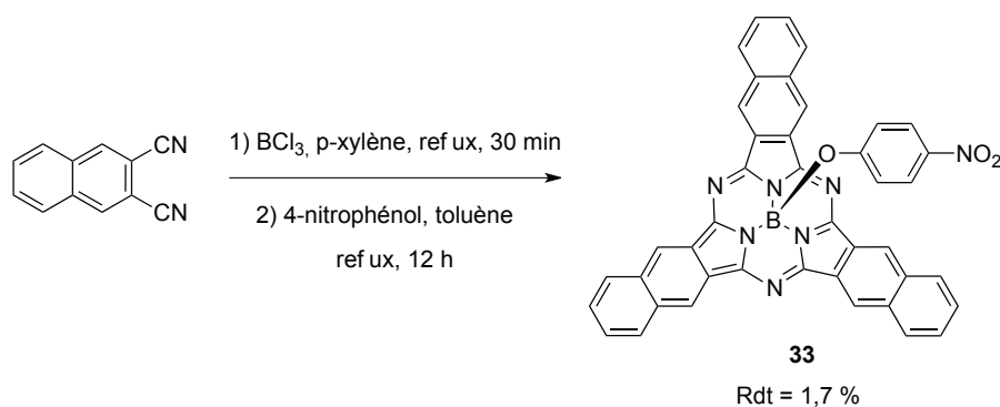
Schéma 32 : Synthèse de la SubNc-NO 2 33
