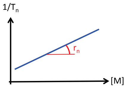
Figure 3 : Vitesse de relaxation en fonction de la concentration métallique
