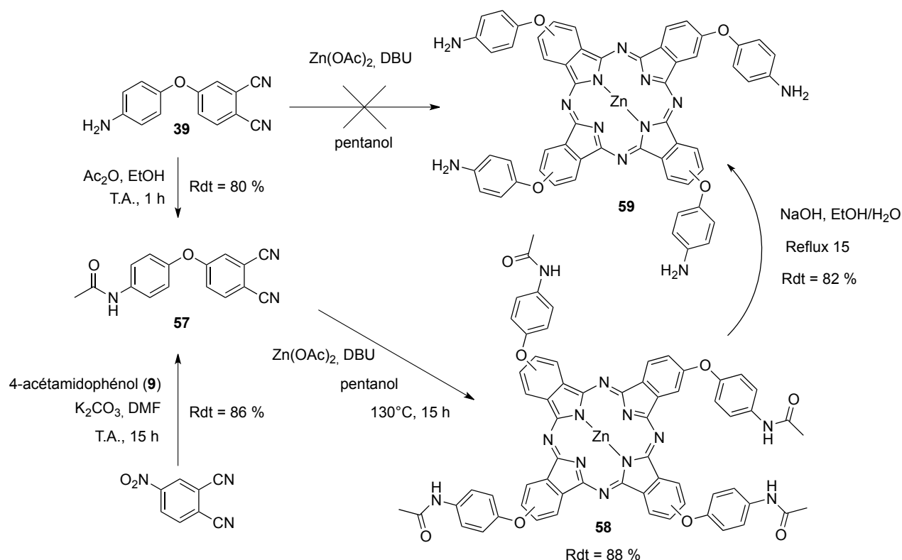
Schéma 47 : Essais de synthèse directe de la phtalocyanine 59 et chemin de synthèse alternatif par protection du précurseur
