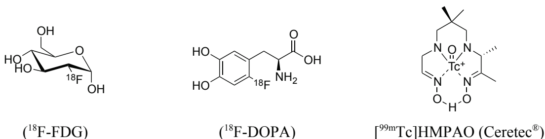
Figure 22 : Structures du ^{18}\text{F} -FDG, du ^{18}\text{F} -DOPA et du Ceretek ®
