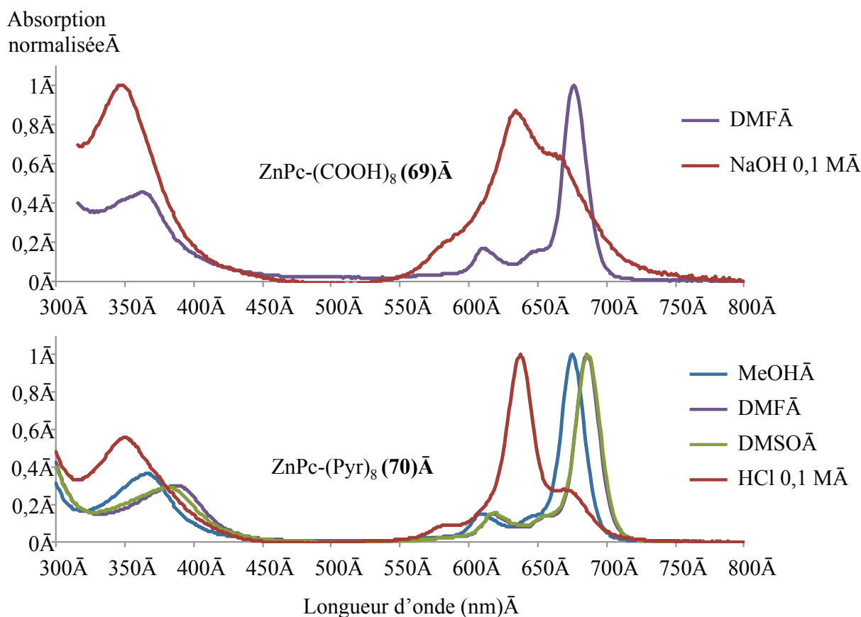
Figure 94 : Superposition des spectres d'absorption du composé 69 dans le DMF et dans la soude 0,1 M et du composé 70 dans le MeOH, le DMF, le DMSO et \text{H}_2\text{O}
