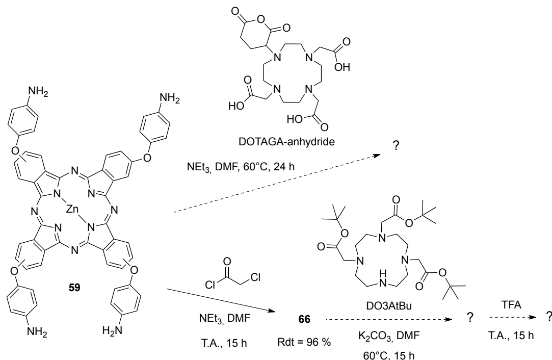
Schéma 51 : Essais d'introduction de quatre agents chélatants à partir de la phtalocyanine 59
