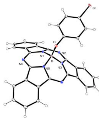
Figure 60 : Vue ORTEP du composé 7
