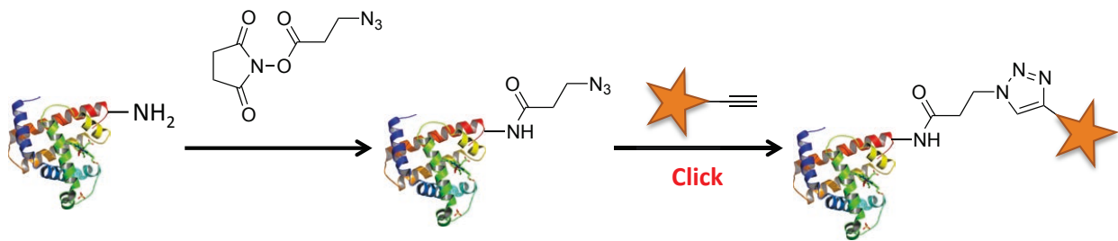
Schéma 3 : Exemple de méthode de biovectorisation en deux temps par chimie click
