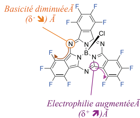
Figure 80 : Conséquences de la présence de substituants périphériques attracteurs
