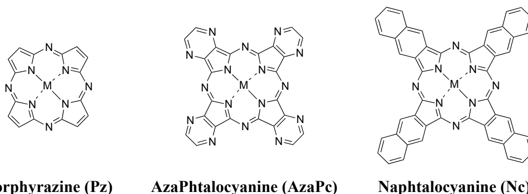
Figure 53 : Structures d'une naphthalocyanine, d'une porphyrazine et d'une azaphtalocyanine
