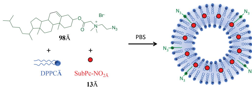
Schéma 73 : Préparation du liposome fonctionnalisé en surface par des groupes azotures
