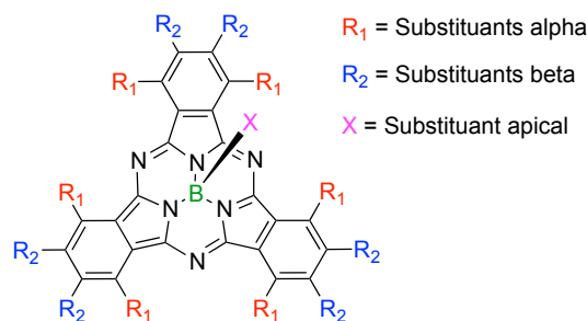
Figure 54 : Structure générale d'une subphtalocyanine et positions de substitution
