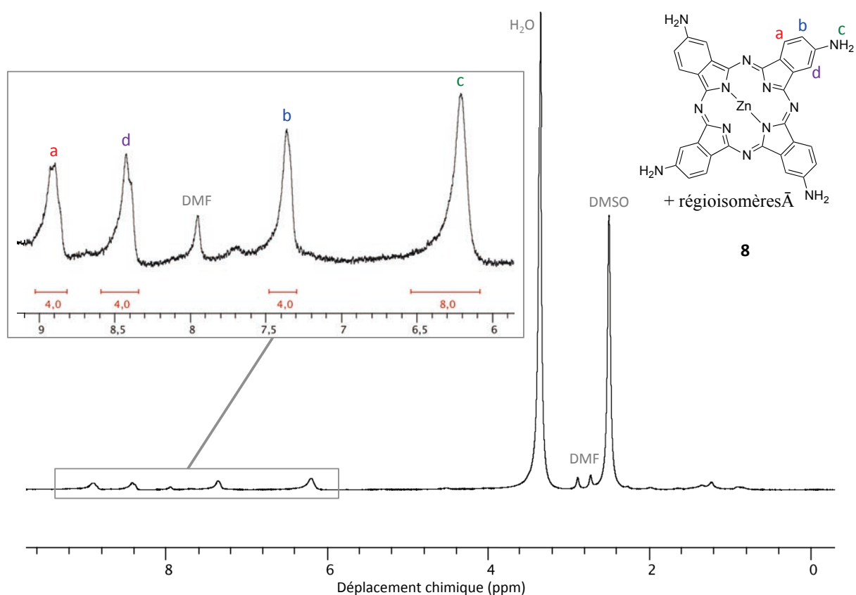
Figure 91 : Spectre de RMN ^1\text{H} de la ZnTAPc 64 et zoom sur la zone des aromatiques
