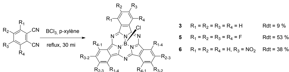
Schéma 14 : Synthèse des subphthalocyanines de départ 3 , 5 et 6
