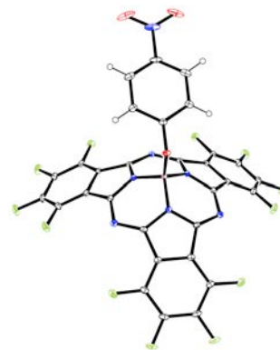
Figure 76 : Vue ORTEP du composé 34
