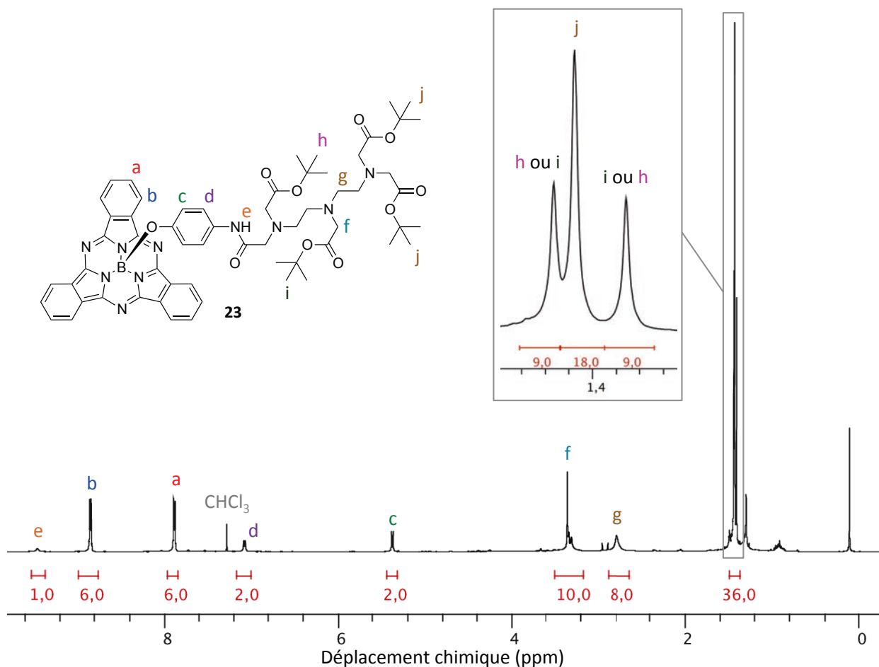
Figure 71 : Spectre de RMN ^1\text{H} du composé 23 ( \text{CDCl}_3 , 500 MHz, 300 K)
