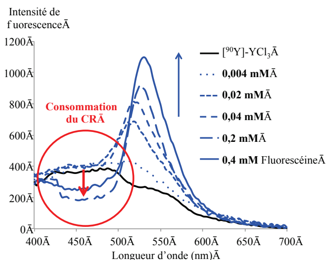
Figure 146 : Reproduction de la figure 143 pour montrer la consommation du signal Cherenkov (CR)
