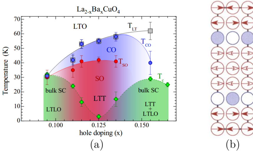
FIGURE 2.2 – (a) Diagramme des phases expérimental du composé \text{La}_{2-x}\text{Ba}_x\text{CuO}_4 dans le plan température - dopage en trous (reproduit de la référence Hücker et al. [184]). Les mesures ont été réalisées par diffraction de rayons X et diffraction des neutrons et ont permis d'obtenir les T_c de la supraconductivité dans le matériau massif, T_{co} de l'ordre de charge et T_{so} de l'ordre de spin. A basse température, la supraconductivité et les ordres de charge et de spin coexistent pour 0.095 \leq x \leq 0.135 . (b) Illustration des rayures antiferromagnétiques de période 4a détectées dans certains cuprates où a est le pas du réseau (reproduit de la référence Tranquada et al. [94]).
