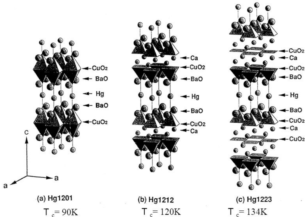
FIGURE 1.6 – Structures cristallines des composés cuprates à base de mercure dont les structures multi-couches (de une à trois, de gauche à droite, respectivement) par maille élémentaire sont tétragonales simples. Figure reproduite de la référence L. Chapman [85].
