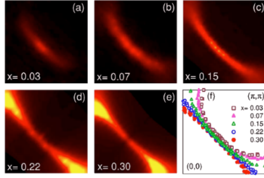
FIGURE 1.16 – Surfaces de Fermi 2D mesurées par ARPES sur des cristaux de LSCO pour différentes valeurs du dopage en trous. Figure reproduite de la référence Yoshida et al. [144].
