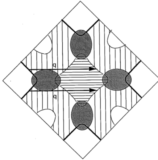
FIGURE 4.1 – Surface de Fermi du chrome projetée dans le plan (1,0,0) . Le vecteur d'onde \mathbf{q} correspond au vecteur de nesting : la poche de trous translattée de ce vecteur devient tangente à la poche d'électrons. La figure est reproduite de la référence M. Héritier [267].
