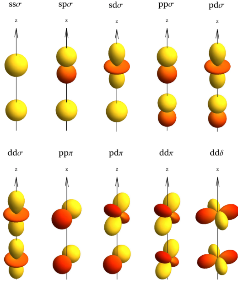
FIGURE 2.7 – Intégrales de saut de Slater-Koster (figure reproduite de la référence G. Autès [214]).
