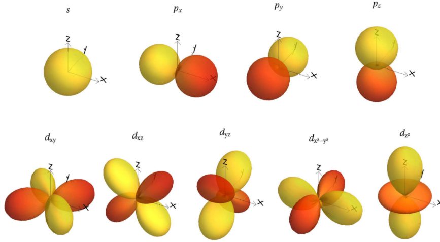
FIGURE 2.6 – La base des orbitales atomiques s, p et d (figure reproduite de la référence G. Autès [214]).
