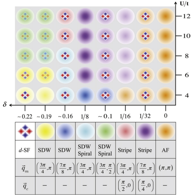
FIGURE 2.1 – Diagramme des phases du modèle de Hubbard bidimensionnel t-U sur réseau carré (cellule de taille 16 \times 4 ) obtenu par la méthode SEMF et qui a permis de capturer quelques aspects du diagramme des phases expérimental des cuprates supraconducteurs (reproduit de la référence Leprévost et al. [21, 22]). En particulier, un ordre à longue portée antiferromagnétique est détecté au demi-remplissage. Des corrélations de paires en onde- d à longue portée entrelacées avec des ondes de densité de spin sont détectées pour certaines valeurs du dopage en trous. Cependant, la présence d’une phase superfluide est non-systématique sur la gamme de dopage en trous \delta \simeq 0 - 0.22 . Une stripe magnétique (régions antiferromagnétiques de phases opposées séparées périodiquement par des rivières de trous) est, par ailleurs, détectée au dopage \delta = 0.125 comme expérimentalement pour certains cuprates mais dont la longueur d’onde de l’ordre de charge est de 8a où a est le pas du réseau.
