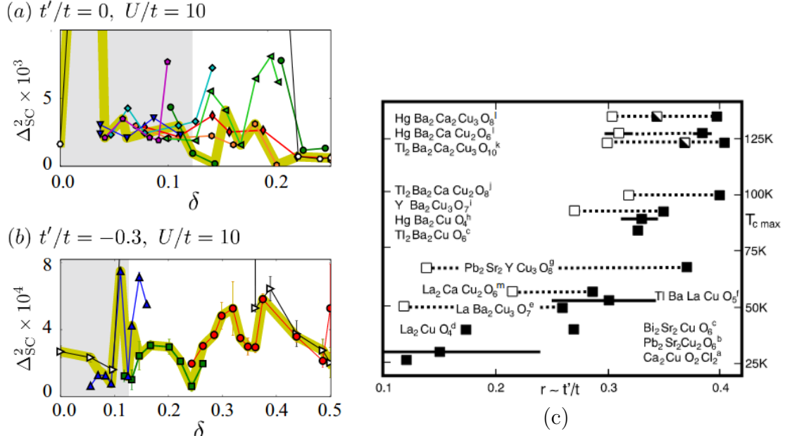
FIGURE 2.4 – (a) et (b) (reproduites de la référence Ido et al. [55]) : paramètre d'ordre supraconducteur en onde-d en fonction du dopage en trous \delta calculé pour le modèle t-t'-U et U/t = 10 . La supraconductivité est évanescente et déjà peu marquée dans le cas où t' = 0 mais celle-ci est considérablement réduite en incluant t' . (c) : figure reproduite de la référence Pavarini et al. [59] montrant une corrélation entre t'/t et T_c^{max} .
