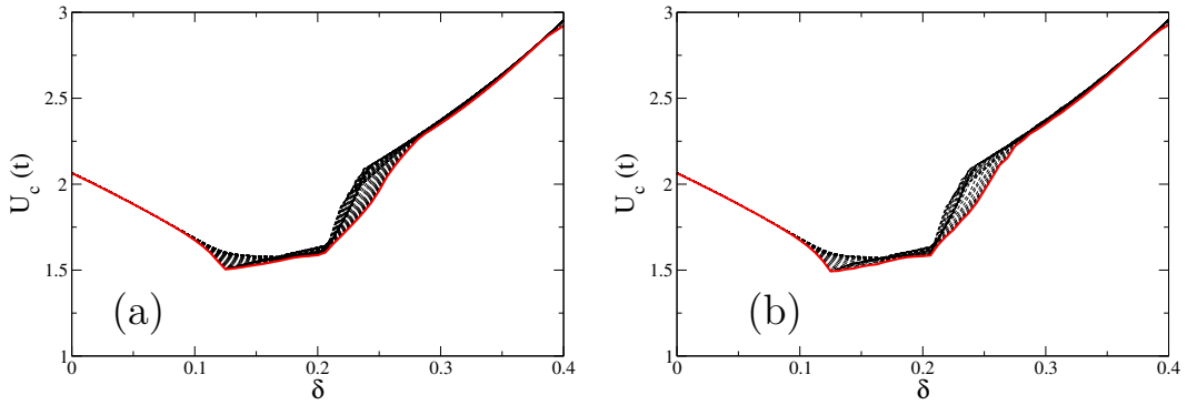
FIGURE 4.14 – (a) U critique (ligne rouge pleine) du modèle 3D calculé sur une cellule de taille 1500 \times 1500 \times 100 à T = t/1000 . (b) U critique (ligne rouge pleine) du modèle 3D calculé sur une cellule de taille 600 \times 600 \times 600 à T = t/1000 . Les lignes tirées noires correspondent au calcul de U_c mais pour chaque q_z variant de 0 à 2\pi/c .
