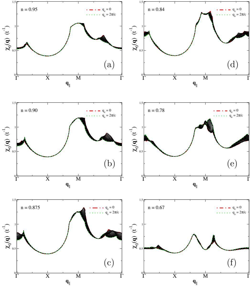
FIGURE 4.3 – Susceptibilités sans interaction \chi_0(\mathbf{q}) en unité de |t|^{-1} calculées pour diverses densités d'électrons et un grand nombre de valeurs de q_z variant de 0 (ligne rouge en traits tirés-pointillés) à 2\pi/c (ligne verte en traits pointillés). (a) n = 0.95 (sous-dopé), (b) n = 0.90 (sous-dopé), (c) n = 0.875 (sous-dopé), (d) n = 0.84 (optimal), (e) n = 0.78 (sur-dopé), (f) n = 0.67 (sur-dopé). Le calcul est réalisé sur une cellule de taille 1500 \times 1500 \times 100 à la température T = t/1000 pour le modèle de liaisons fortes effectif déterminé dans le chapitre 3 en utilisant les amplitudes de saut données par les Eqs. (3.39, 3.40).
