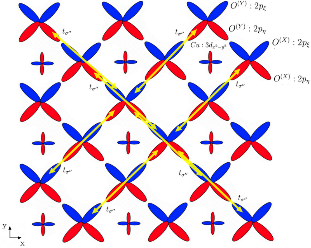
FIGURE 3.4 – Illustration des couplages de type \sigma entre les orbitales 2p_{\xi,\eta}^{(X,Y)} des ions oxygène du plan \text{CuO}_2 troisième plus proches voisins.
