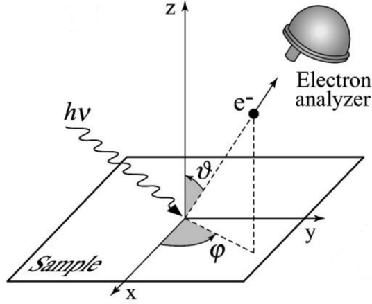
FIGURE 1.15 – Illustration de la géométrie d’une expérience ARPES dans laquelle la direction d’émission du photoélectron est paramétrée par les angles polaire ( \theta ) et azimutal ( \phi ). La figure est reproduite de la référence Damascelli et al. [26].
