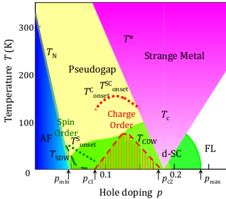
FIGURE 1.9 – Diagramme des phases générique pour les cuprates dopés en trous (figure reproduite de la référence Keimer et al. [99]).
