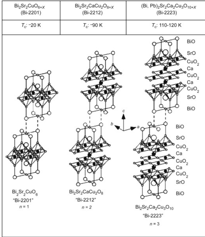
FIGURE 1.4 – Structures cristallines tétragonales centrées des composés cuprates à base de bismuth constitués de un à trois plans par maille élémentaire (Bi-2201, Bi-2212, Bi-2223, de gauche à droite, respectivement). Dans la direction perpendiculaire aux plans \text{CuO}_2 , les mailles élémentaires se trouvent décalées de (a/2, a/2, 0) . Figure reproduite de la référence J.-I. Shimoyama [78].
