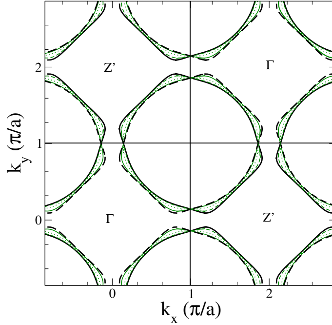
FIGURE 3.24 – Projection des surfaces de Fermi sur le plan de base pour plusieurs valeurs représentatives de k_z au dopage \delta = 1/8 = 1 - n pour le modèle effectif à une bande impliquant t, t', t'', t''', \theta, et \theta'' (voir Eqs. (3.39, 3.40)). Paramètres : k_z = 0 (ligne noire pleine), k_z = \pi/2c (ligne verte en traits tirés), k_z = \pi/c (ligne verte en traits pointillés), k_z = 3\pi/2c (ligne verte pleine) et k_z = 2\pi/c (ligne noire en traits tirés). Les paramètres de liaisons fortes utilisés sont donnés dans le Tableau 3.1.
