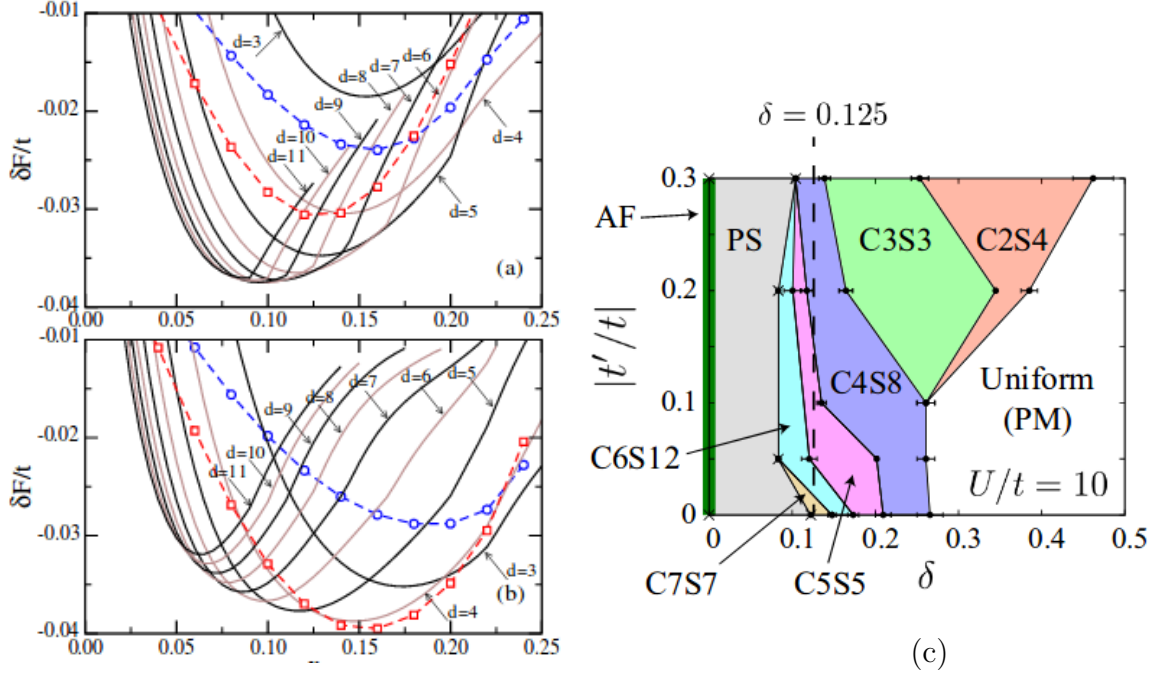
FIGURE 2.3 – (a) et (b) (reproduites de la référence Raczkowski et al. [182]) : gain d'énergie libre \delta F de la phase rayure magnétique par rapport à la phase antiferromagnétique en fonction du dopage en trous x pour le modèle de Hubbard t - t' - U avec U = 12t pour t' = 0 (a) et t' = -0.15 (b). Les parois de domaine sont séparées par 3,...,11 pas du réseau. On constate que t' favorise énergétiquement l'émergence de la stripe de période 4a au dopage 1/8 . (c) Figure du diagramme des phases magnétiques dans le plan |t'/t| - \delta obtenu récemment par Ido et al. [55] montrant que le t' \simeq -0.1t usuel pour les cuprates monocouches au lanthane corrige la période de la stripe magnétique par rapport au modèle t - U .
