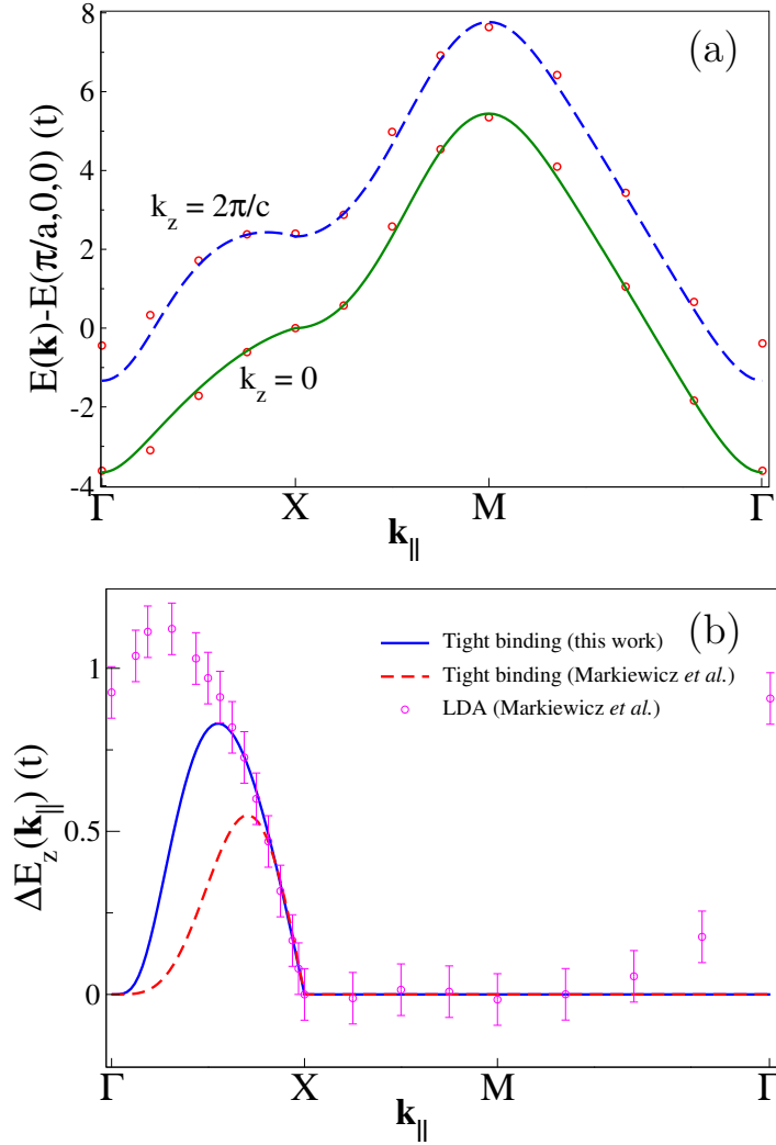
FIGURE 3.9 – (a) Comparaison de la dispersion de la bande de conduction obtenue par les calculs de DFT par Markiewicz et al. [61] (cercles) à celle obtenue dans notre modèle de liaisons fortes. Ici, E(\pi/a, 0, 0) définit le zéro d'énergie et la ligne en traits tirés décrivant la bande pour k_z = 2\pi/c est décalée de 1 eV, afin d'apporter une meilleure visibilité. (b) Différence en énergie \Delta E_z(\mathbf{k}_{\parallel}) Eq. (3.24) en fonction de \mathbf{k}_{\parallel} . Les paramètres de liaisons fortes utilisés sont donnés dans le Tableau 3.1 et t/t_{pd} = 0.283 .
