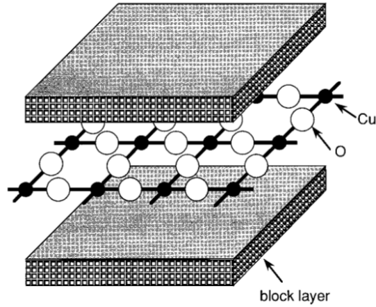
FIGURE 4 – Représentation des plans de conduction \text{CuO}_2 intercalés entre les couches atomiques “réservoirs de charges” (figure reproduite de la référence Imada et al. [60]).
