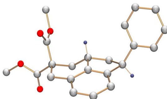
Figure 2. Cliché de diffraction des rayons X de B6a (les hydrogènes sont omis pour plus de clarté)
