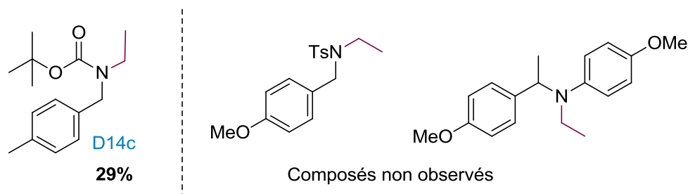
Schéma 237. Imines possédant un groupement protecteur et cétimine éthylées
