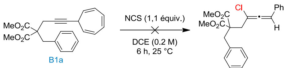
Schéma 149. Absence de réactivité de B1a en présence de NCS
