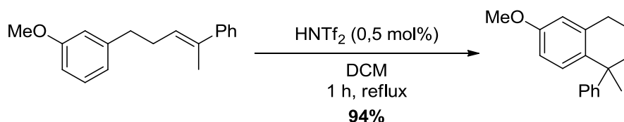
Schéma 92. Hydroarylation d'arénènes catalysée par \text{HNTf}_2
