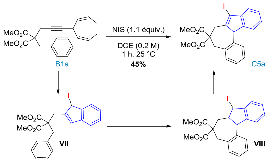
Schéma 150. Réactivité de B1a en présence de NIS
