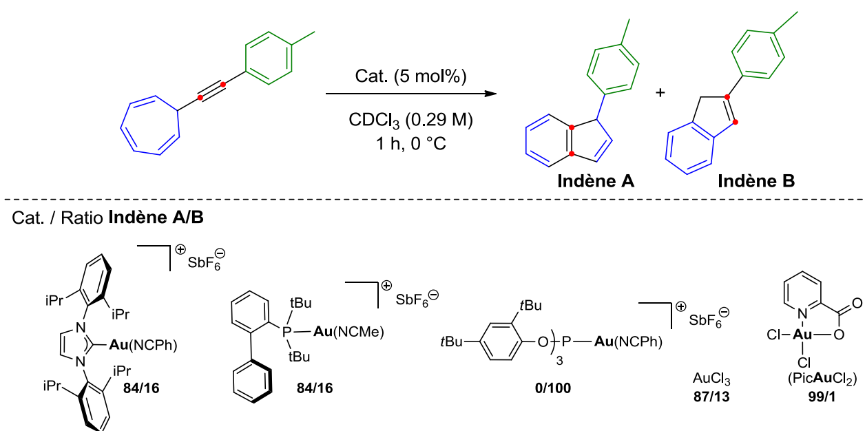
Schéma 98. Traitement d'un 7-alcynylcycloheptatriène avec divers catalyseurs d'or
