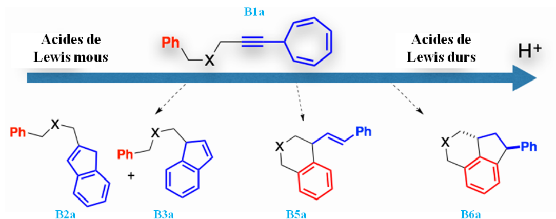
Figure 5. Structure des différents composés obtenus en fonction de l'acidité de Lewis \pi du catalyseur
