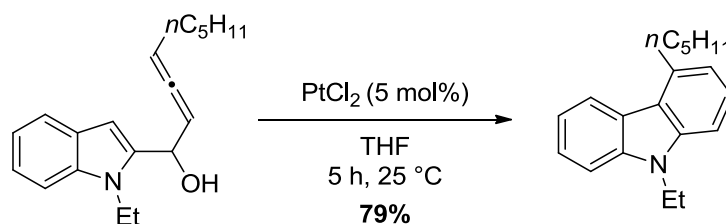
Schéma 79. Synthèse de carbazoles par réaction tandem d'hydroarylation/hydroxylation
