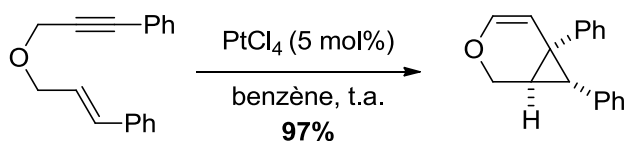
Schéma 64. Formation d'oxabicyclo[4.1.0]heptène catalysée par \text{PtCl}_4
