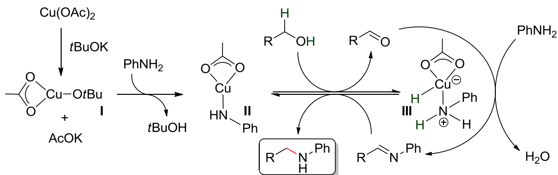
Schéma 210. Mécanisme proposé pour la N-alkylation d'amines avec des alcools catalysée par \text{Cu(OAc)}_2
