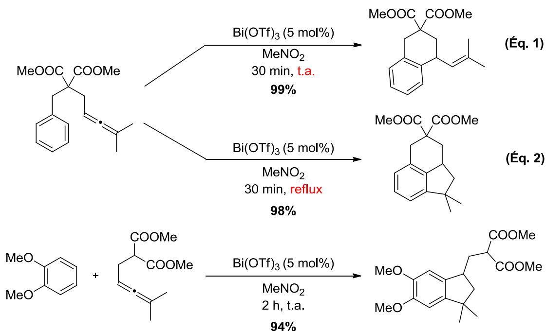
Schéma 26. Hydroarylation d'allènes catalysée par \text{Bi}(\text{OTf})_3
