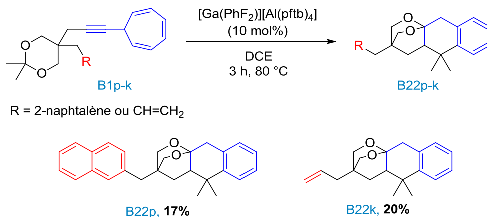
Schéma 123. Exemplification de la réaction en présence de [\text{Ga}(\text{PhF}_2)][\text{Al}(\text{pftb})_4]
