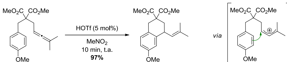
Schéma 90. Hydroarylation d'un arylallène catalysée par \text{HOTf}
