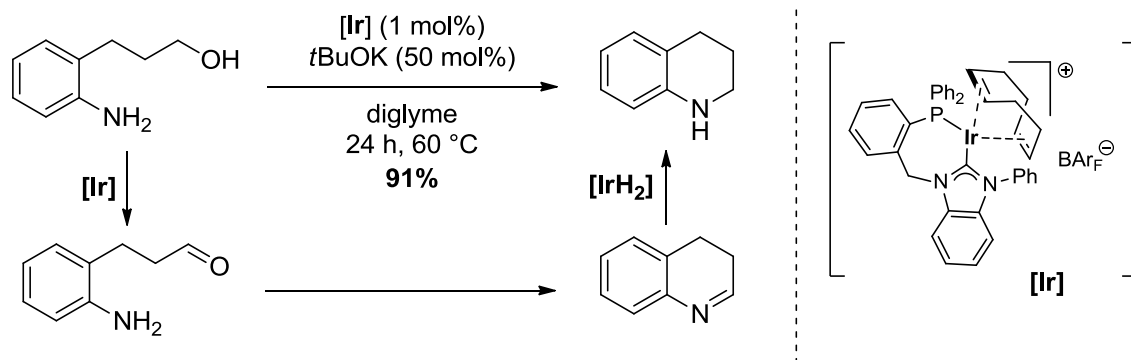
Schéma 204. Réaction d'amination d'alcools intramoléculaire
