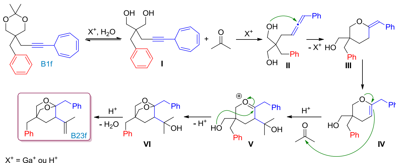
Schéma 120. Mécanisme proposé pour la formation du composé B23f
