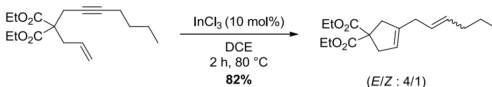
Schéma 71. Cycloisomérisation d'énynes-1,6 avec un alcyne disubstitué catalysée par \text{InCl}_3
