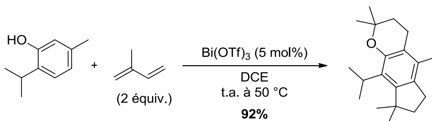
Schéma 24. Double réaction tandem entre le thymol et l'isoprène
