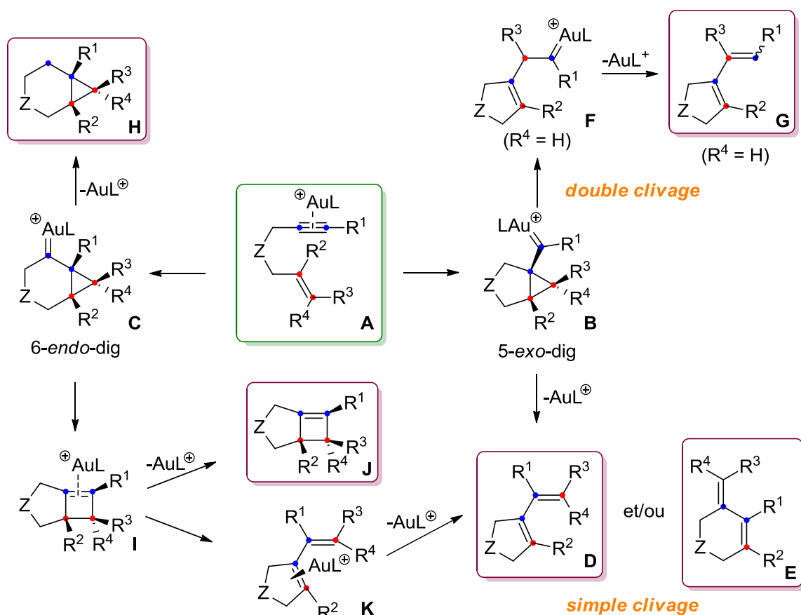
Schéma 57. Mécanisme général pour les cycloisomérisations d'ényne-1,6
