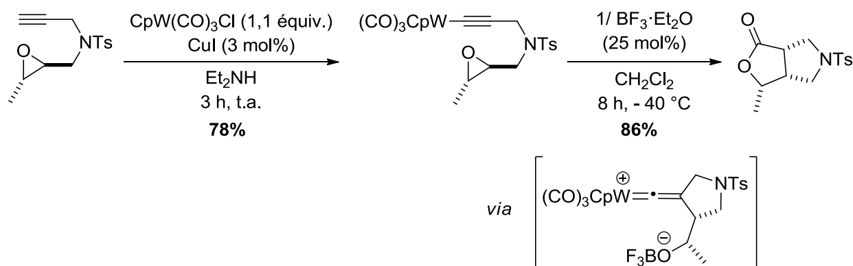
Schéma 12. Cycloaddition [3+2] d'un alcynyltungstène avec un époxyde
