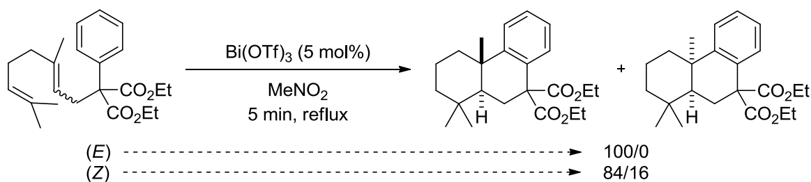
Schéma 28. Cyclisation d'un aryldiène en présence de \text{Bi}(\text{OTf})_3
