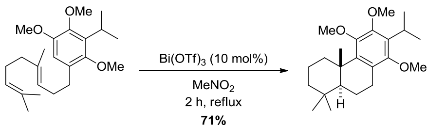
Schéma 29. Synthèse d'un composé tricyclic catalysé par \text{Bi}(\text{OTf})_3
