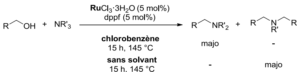
Schéma 200. Alkylation d'amines tertiaires par des alcools
