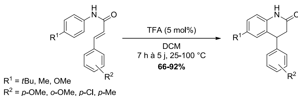
Schéma 91. Hydroarylation d'aryl-cinnamides catalysée par le \text{TFA}
