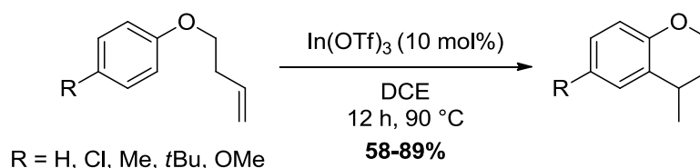
Schéma 87. Synthèse de dérivés du chromane catalysée par \text{In}(\text{OTf})_3
