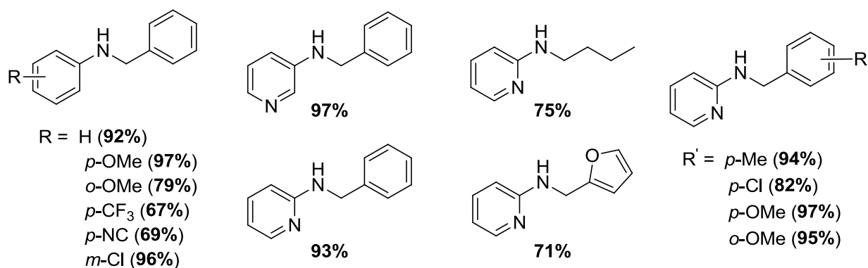
Schéma 206. Sélection de composés synthétisés par amination directe d'alcools
