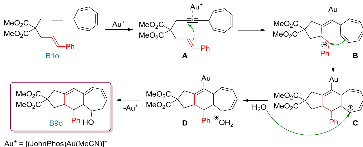
Schéma 111. Mécanisme proposé pour la formation du composé B9o
