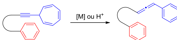
Schéma 49. 7-Alcynylcycloheptatriène arylé et sa forme isomérisée en phényllallène
