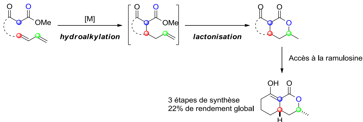
Schéma 44. Réaction tandem d'hydroalkylation/lactonisation sur des \beta -cétoesters 1,3-diénoïques
