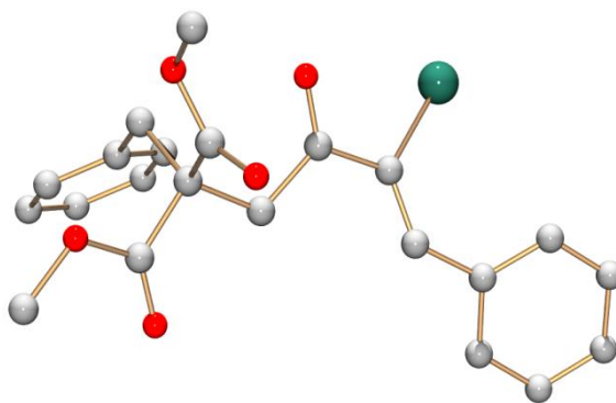
Figure 6. Structure de la bromoénone C2 déterminée par diffraction RX (les hydrogènes sont omis pour plus de clarté)
