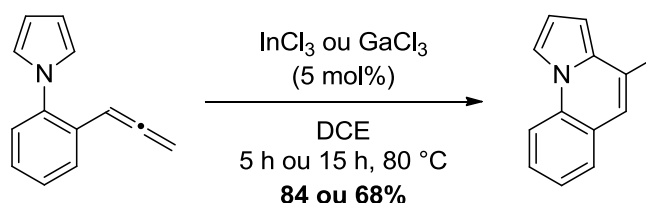
Schéma 84. Hydroarylation d'un allène catalysée par \text{InCl}_3 et \text{GaCl}_3
