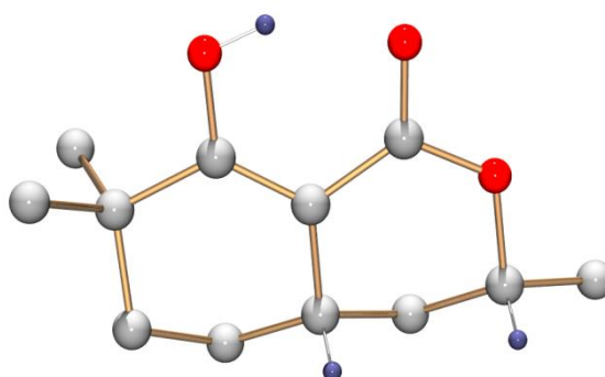
Figure 1. Structure de la bicyclolactone A3a obtenue par diffraction des rayons X (les hydrogènes sont omis pour plus de clarté)
