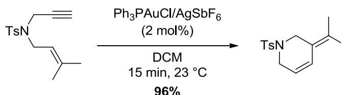
Schéma 59. Réarrangement d'énynes 1,6 par cyclisation 6- endo -dig et simple clivage
