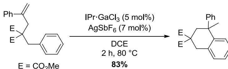
Schéma 86. Cyclisation d'un arénène
