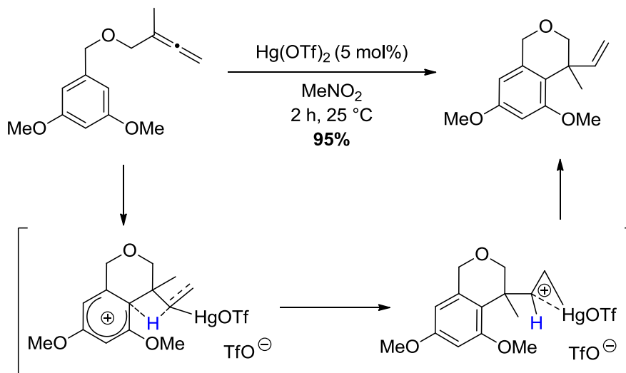
Schéma 83. Hydroarylation d'aryllallènes catalysée par \text{Hg}(\text{OTf})_2
