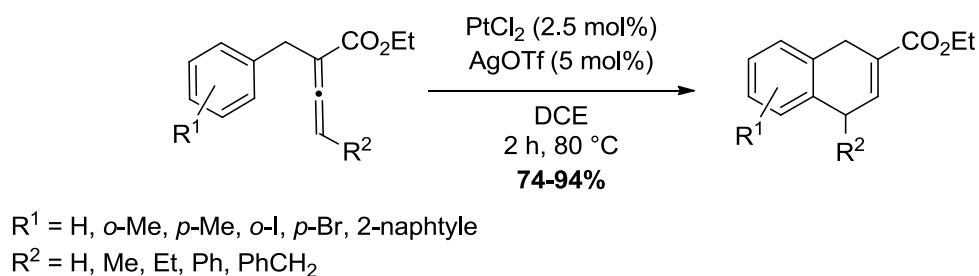
Schéma 81. Synthèse de 1,4-dihydronaphtalènes catalysée par un complexe de platine
