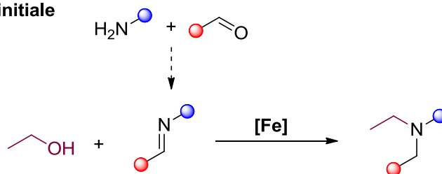
Schéma 191. Stratégie envisagée pour la synthèse d'amines tertiaires dissymétriques
