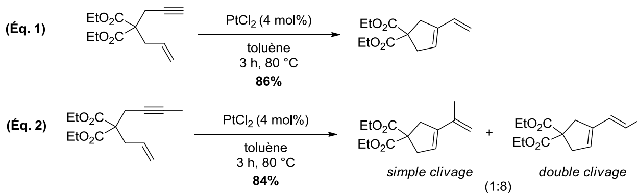
Schéma 62. Cycloisomérisation d'énynes-1,6 catalysée par \text{PtCl}_2
