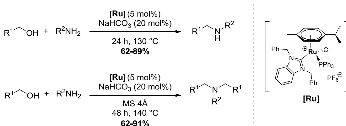
Schéma 198. Monoalkylation et dialkylation d'amines primaires par l'équipe de Huynh
