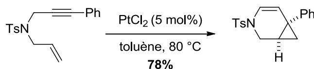
Schéma 65. Formation d'azabicyclo[4.1.0]heptène catalysée par \text{PtCl}_2
