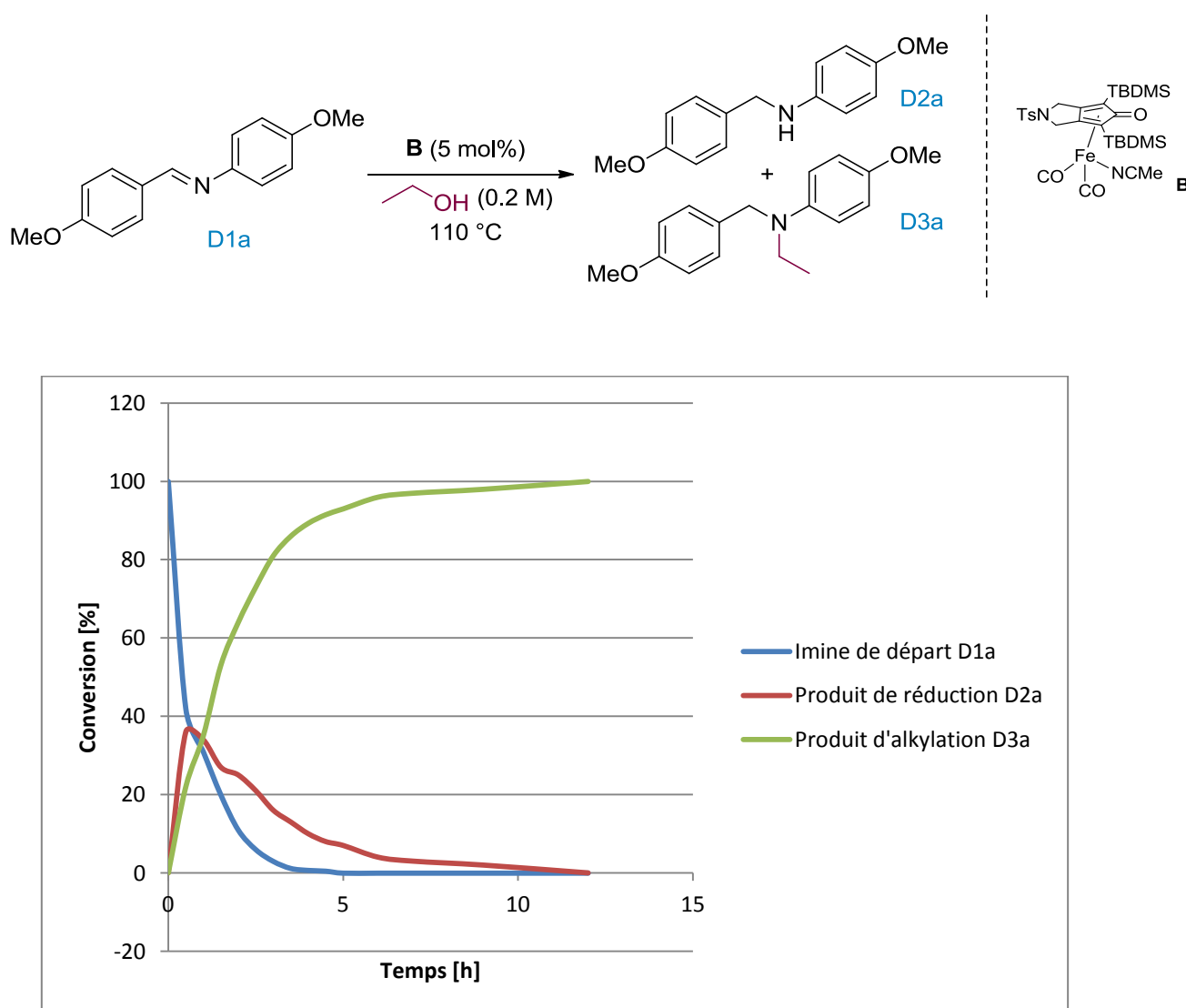
Figure 7. Suivi cinétique par GC de la réaction de N-éthylation d'imine avec l'éthanol
