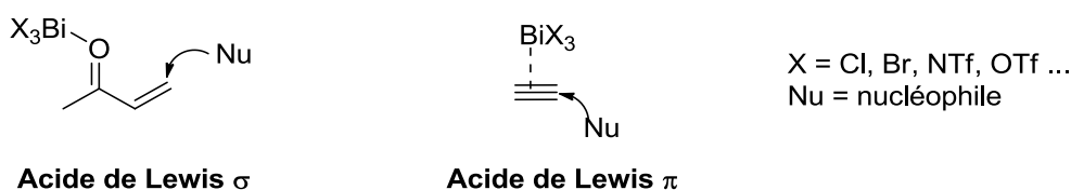
Schéma 19. Acidités de Lewis \sigma et \pi des sels de Bi(III)
