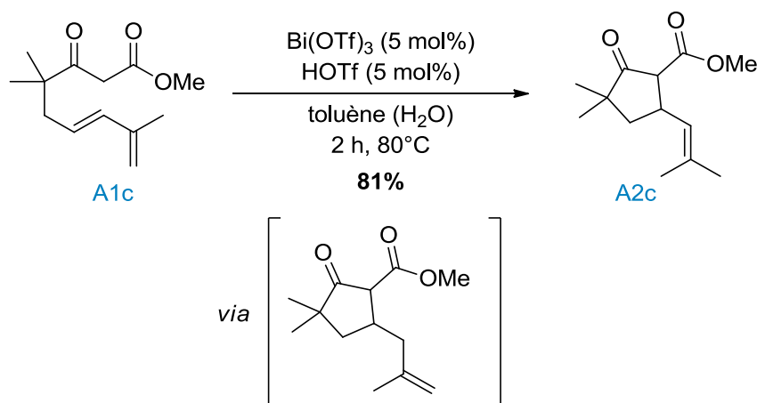
Schéma 35. Cyclisation du \beta -cétoester A1c
