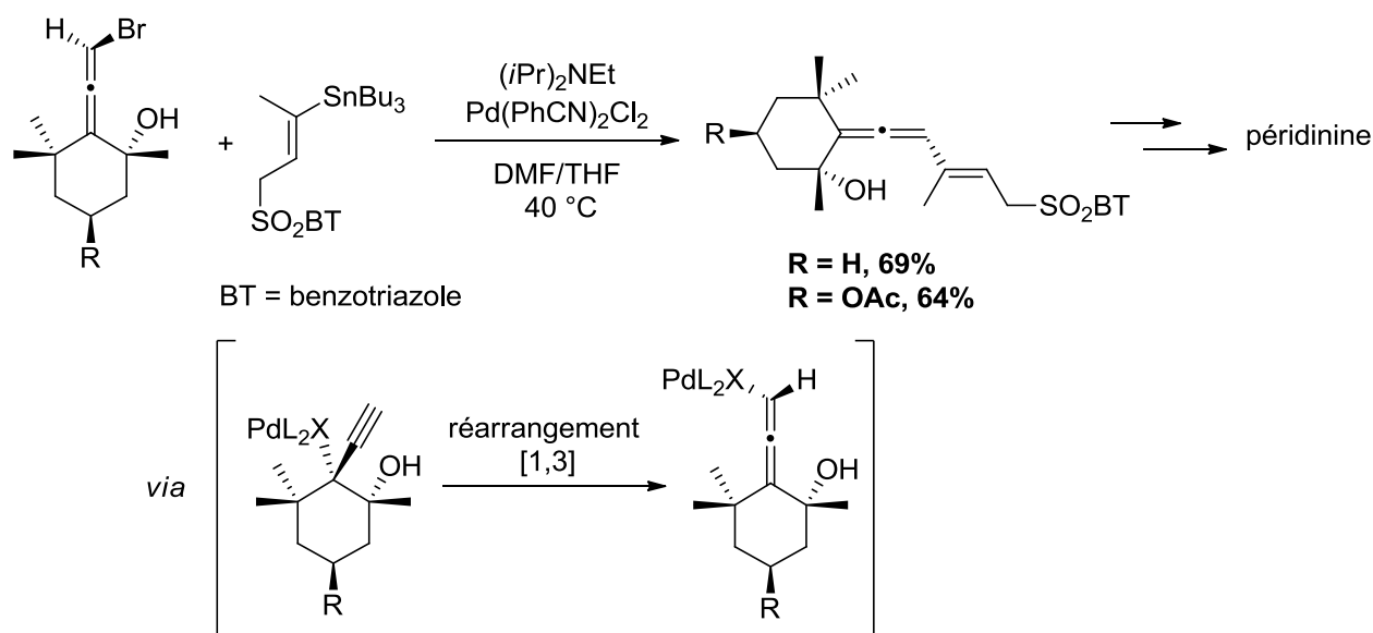
Schéma 161. Formation d'un intermédiaire à la synthèse totale de la péricidine
