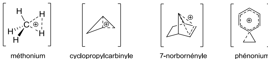
Schéma 53. Exemples de carbocations non classiques
