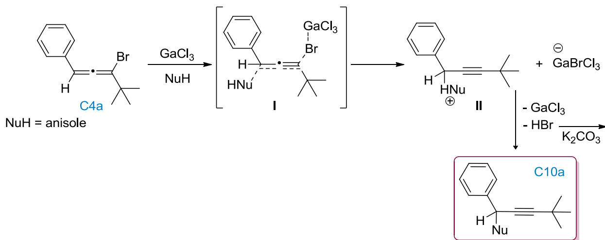
Schéma 174. Mécanisme proposé pour la formation de C10a
