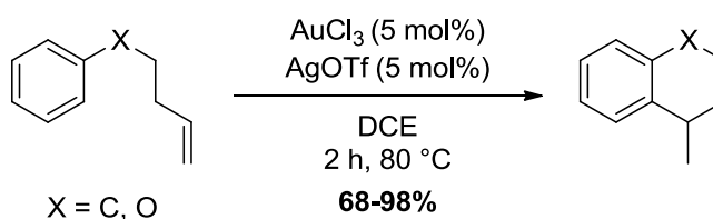
Schéma 78. Hydroarylation intramoléculaire d'alcènes non activés
