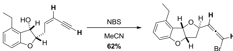
Schéma 136. Réaction de bromoéthérification pour accéder au (±)-panacène
