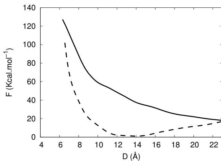
Figure 7.14 – Profil d'énergie libre pour le PAAm (ligne pleine) et le PDMA (ligne pointillée) dans un solvant explicite.
