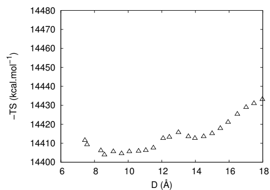
(d) Entropy (-TS) of PDMA.
