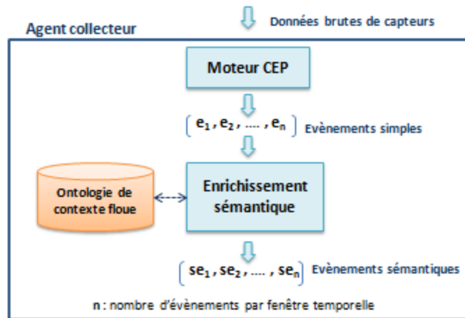
FIGURE 2.5. Processus d'enrichissement sémantique des événements
