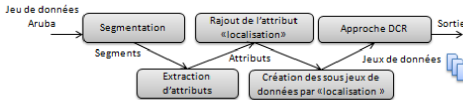
FIGURE 5.2. Pré-traitement du jeu de données Aruba pour simuler l'approche DCR
