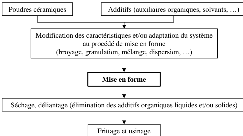
Figure I-16 : Procédé d'élaboration général d'une pièce céramique.
