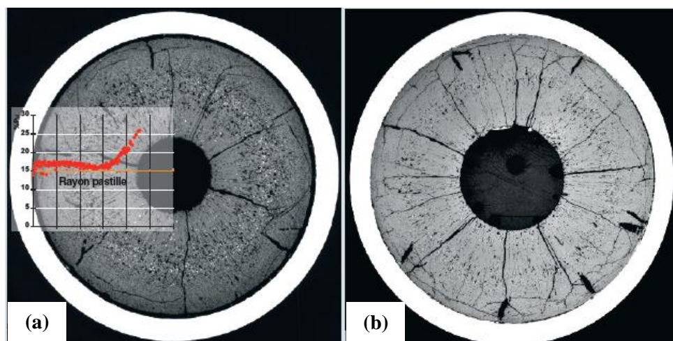
Figure I-13 : Vue transversale d'un combustible Phénix initialement plein avec le profil de concentration en plutonium le long du rayon de la pastille (graphique) (a) et d'un combustible Superphénix initialement annulaire (b) [23].
