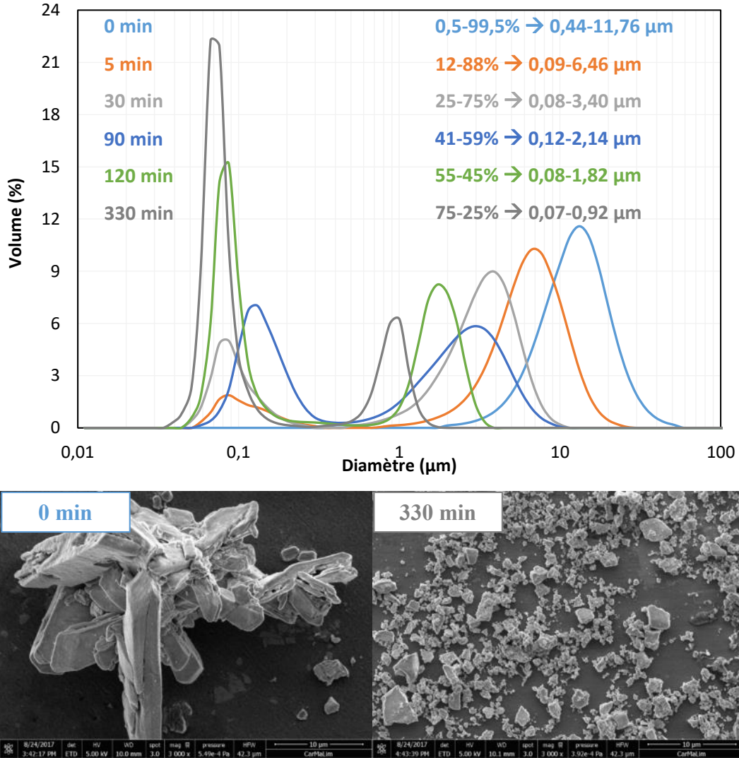
Figure IV-10 : Suivi granulométrique d'une suspension aqueuse de CeO_2 ex-oxalate (20% en volume) calcinée à 800^\circ C placée dans un Turbula® en présence de billes de 2 mm de diamètre et clichés MEB-FEG de la poudre avant et après désagglomération.
