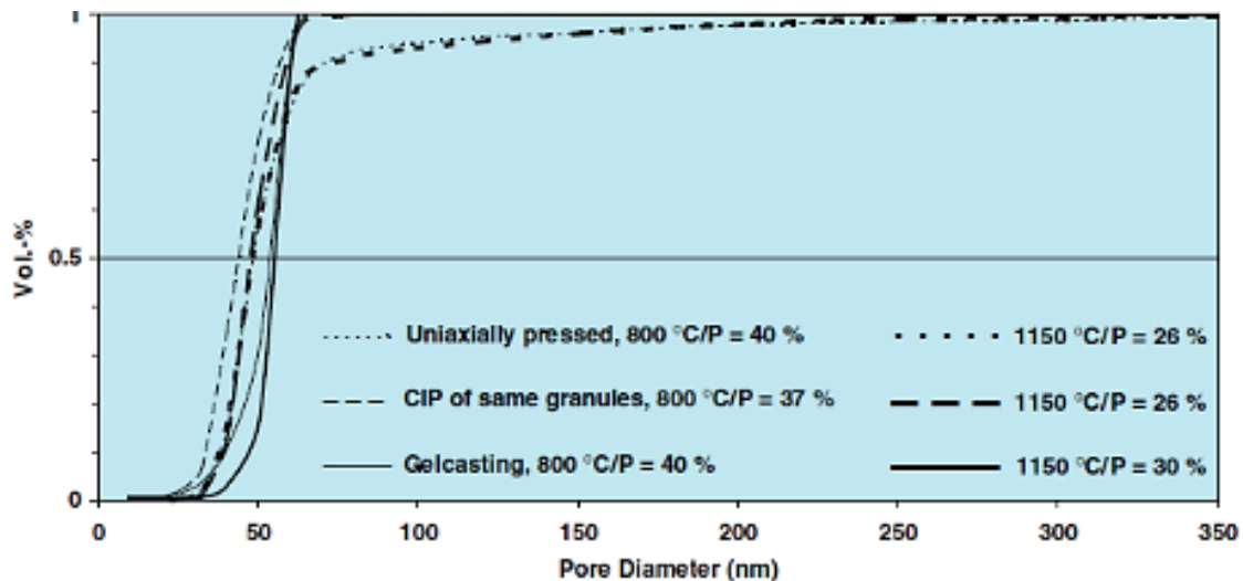
Figure I-23 : Distribution en taille de pores d'échantillons d' \text{Al}_2\text{O}_3 élaborés par pressage uniaxial, pressage isostatique à froid et coulage-gélification [96].
