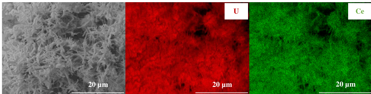
Figure IV-22 : Analyse EDXS couplée au MEB de la poudre (\text{U,Ce})\text{O}_2
