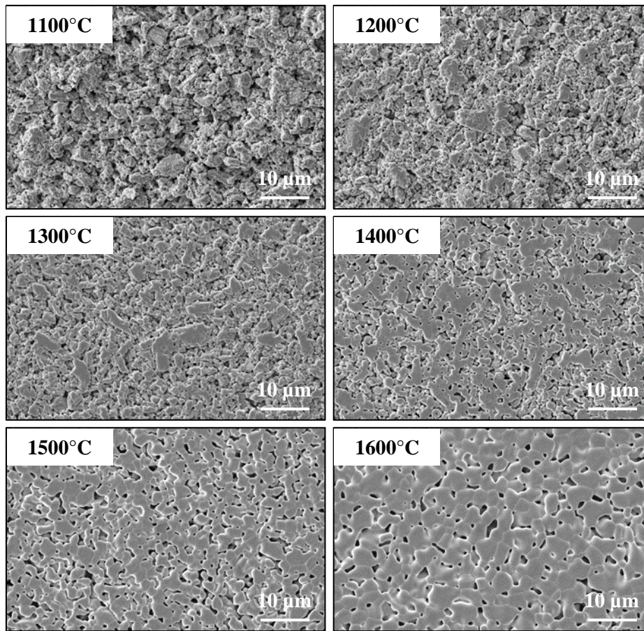
Figure IV-18 : Microstructures de faces polies de pastilles de \text{CeO}_2 ex-oxalate (800-1) élaborées par coulage-gélification (F1-44% en volume) et frittées à différentes températures.
