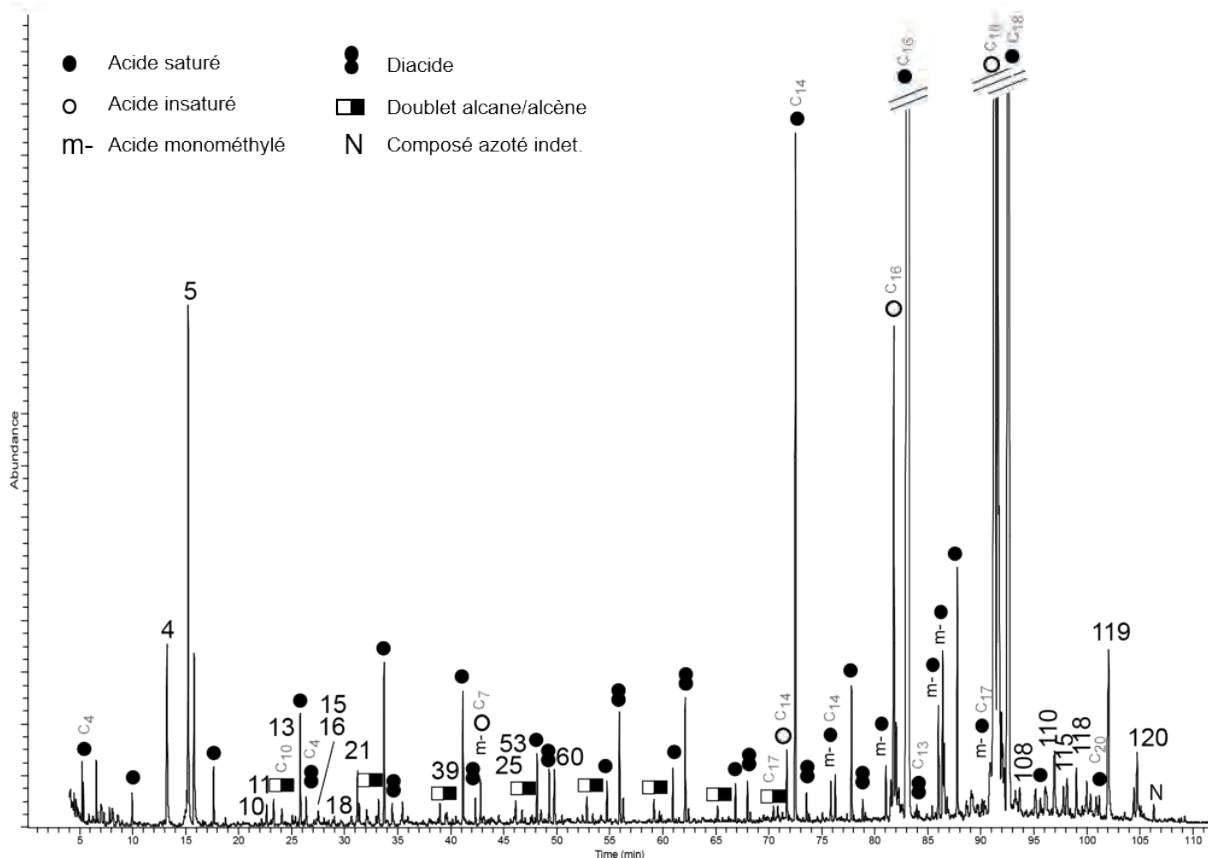
Figure IV.107: Pyrochromatogramme de l'échantillon 2014 Ib (les numéros renvoient au Tabl. Ann. G.1 ; p, dérivés de plastique et polluants, c, colonne, tmah : dérivés du TMAH ; C x indique le nombre de carbonnes sur la chaîne linéaire pour les composés les plus courts, les plus longs et les principaux contributeurs de chaque série).
