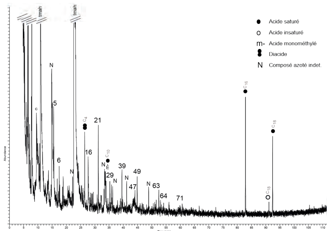
Figure IV.106: Pyrochromatogramme de l'échantillon 2014 Ia (les numéros renvoient au Tabl. Ann. G.1 ; p, dérivés de plastique et polluants, c, colonne, tmah : dérivés du TMAH ; C x indique le nombre de carbonnes sur la chaîne linéaire pour les composés les plus courts, les plus longs et les principaux contributeurs de chaque série).
