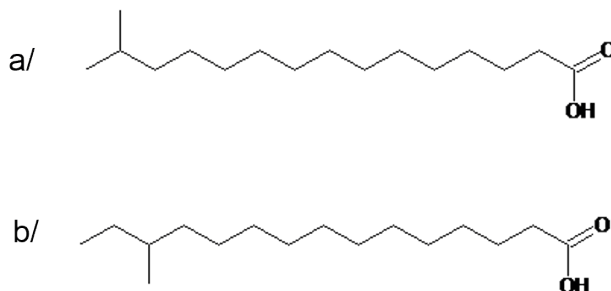
Figure III.10: Acides méthylés C 15:0 . a/ iso-C 15:0 b/ anteiso-C 15:0
