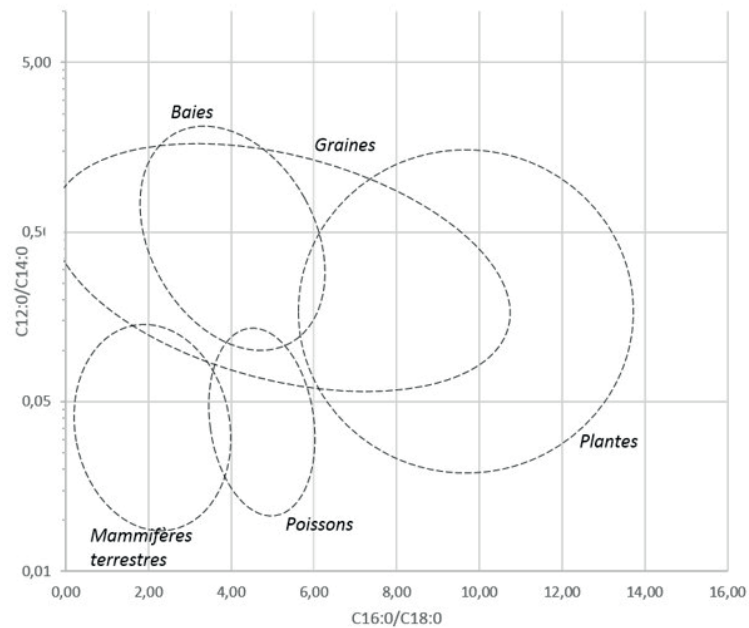
Figure III.36: Biplot des ratios C_{16:0}/C_{18:0} et C_{12:0}/C_{14:0} . Les ellipses ne sont pas statistiques (d'après Eerkens, 2005).
