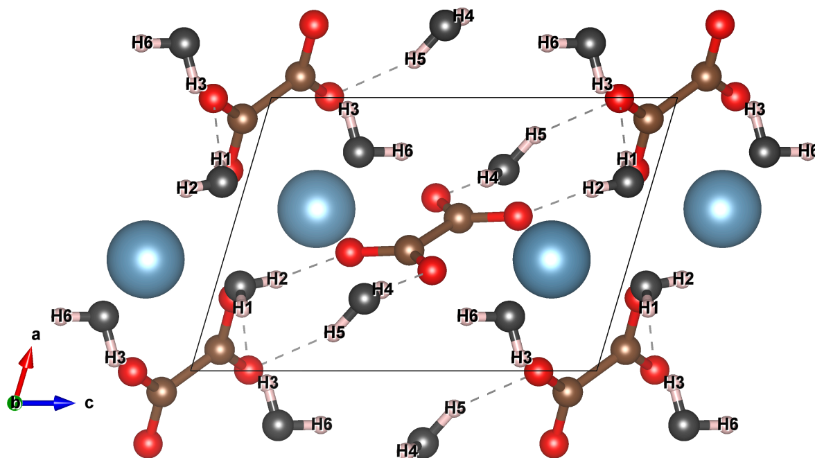
FIGURE 3.5 : Structure de la COT, en bleu Ca, en marron C, en rouge O des oxalates, en noir O de \text{H}_2\text{O} et en blanc H.
