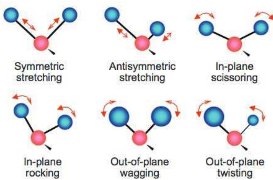
FIGURE 2.3 : Les différents modes vibrationnels [61].
