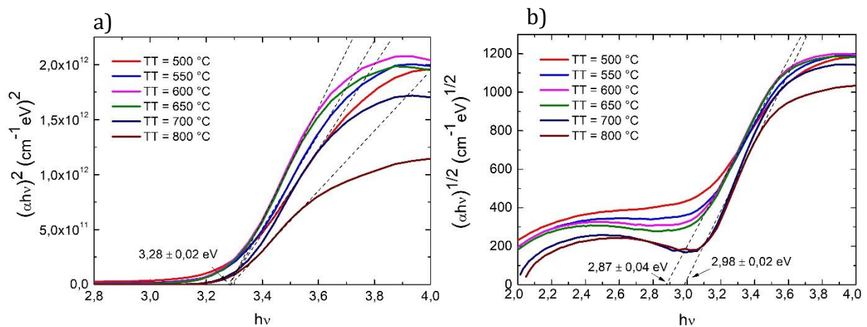
Figure 5-9 : Courbe représentant a) (\alpha h\nu)^2 et b) (\alpha h\nu)^{1/2} en fonction de h\nu pour les couches minces de \text{Cu}(\text{Cr,Fe})\text{O}_2:\text{Mg} d'épaisseur 100 nm traitées à différentes températures.
