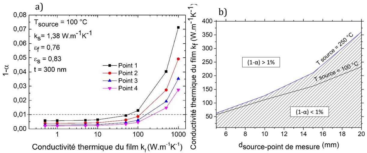
Figure 6-9 : a) Variation de (1-\alpha) en fonction de la conductivité thermique du film lorsque l'on applique 100\text{ °C} . b) Limite de la conductivité thermique du film en fonction de la distance entre la source et le point de mesure pour deux températures appliquées ( 100 et 250\text{ °C} ).
