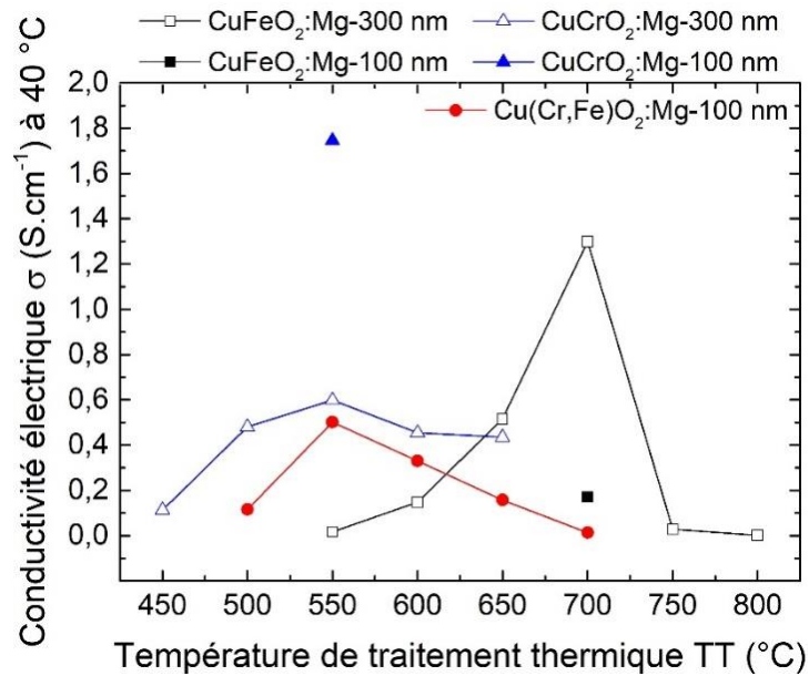
Figure 5-17 : Conductivité électrique à 40\text{ °C} des oxydes de lafossite étudiés en fonction de la température de traitement thermique.
