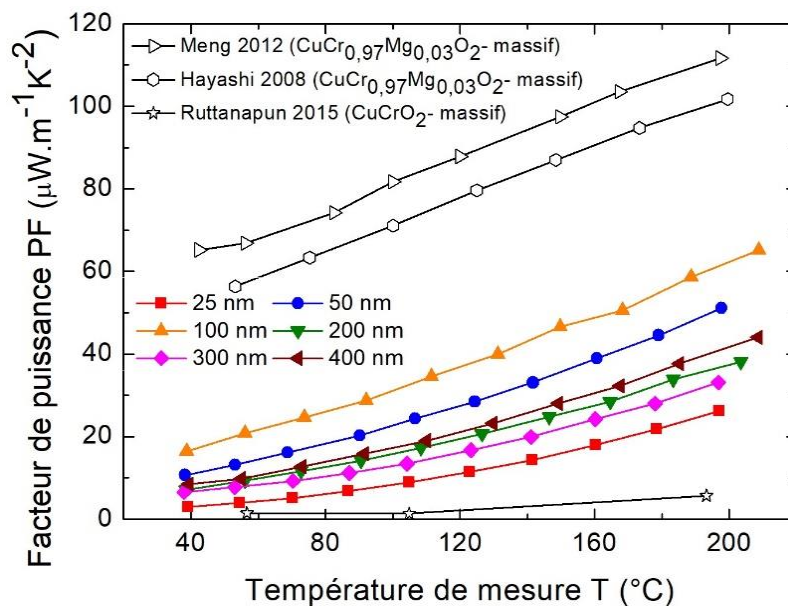
Figure 3-28 : Facteur de puissance des couches minces \text{CuCrO}_2\text{:Mg} recuites à 550 °C sous vide en fonction de la température de recuit en comparaison avec les données de la littérature.
