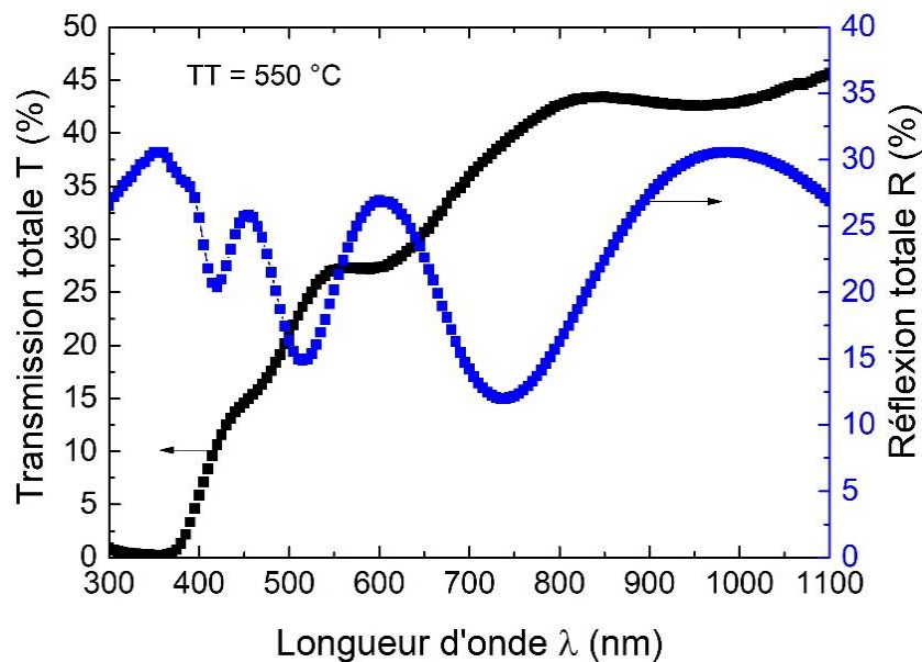
Figure 3-8 : Transmission totale et réflexion totale de la couche mince \text{CuCrO}_2:\text{Mg} recuite sous vide à 550\text{ °C} en fonction de la longueur d'onde.
