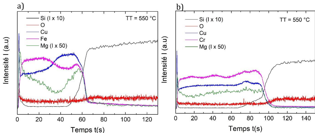
Figure 5-16 : Spectre d'émission lumineuse a) de la couche mince de \text{CuFeO}_2:\text{Mg} et b) \text{CuCrO}_2:\text{Mg} toutes les deux d'épaisseur 300 nm et traitées à 550^\circ\text{C} sous vide.
