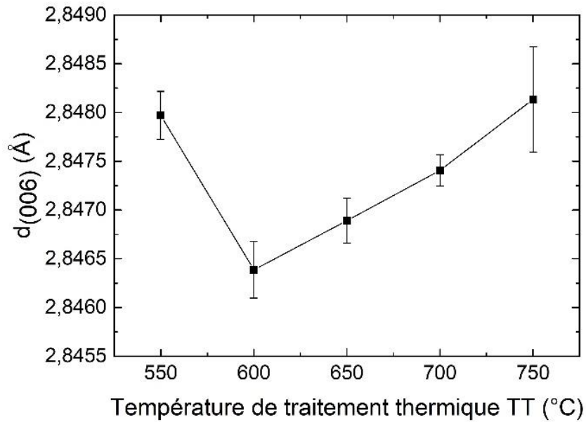
Figure 4-3 : Variation de la distance (006) en fonction de la température de traitement thermique.
