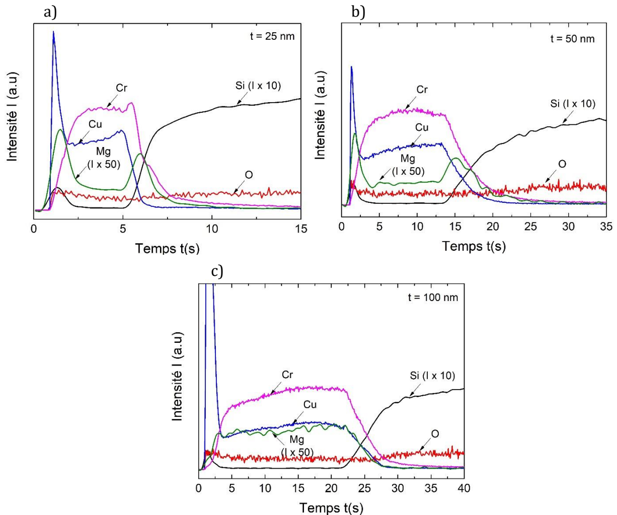
Figure 3-24 : Spectres d'émission lumineuse des couches minces \text{CuCrO}_2:\text{Mg} recuites à 550^\circ\text{C} d'épaisseur a) 25 nm, b) 50 nm et c) 100 nm.
