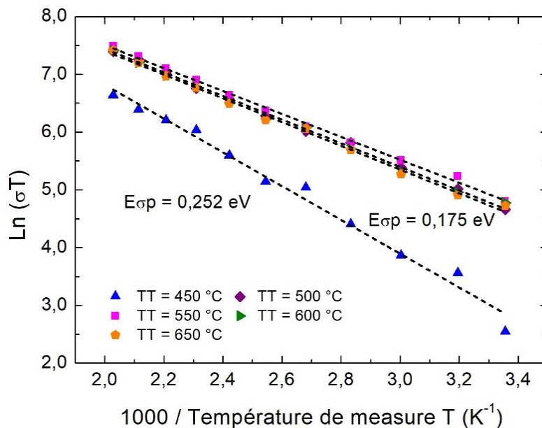
Figure 3-13 : \ln(\sigma T) des couches minces de CuCrO 2 :Mg recuites sous vide en fonction de 1000/T .
