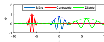
(c) Ondelettes de Morlet (partie réelle en trait plein et module en pointillés)
