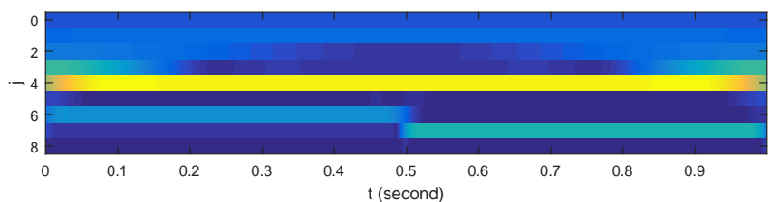
(f) Représentation temps-échelle avec les ondelettes de Morlet
