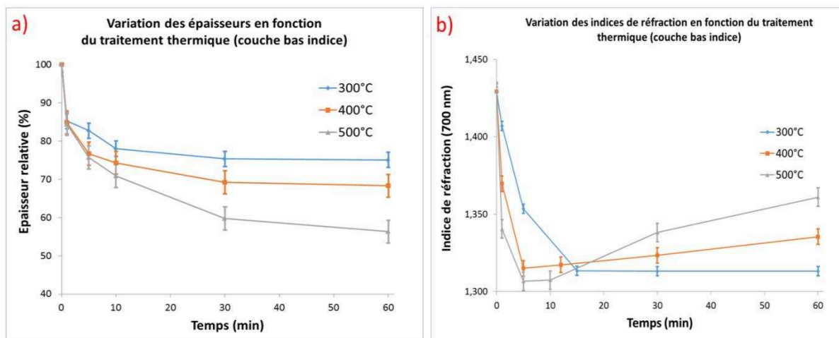
Annexe III.3 : Etude du traitement thermique (en temps et en température) sur la couche bas indice : a) variation des épaisseurs relatives ; b) variation des indices de réfraction. Les barres d'erreurs correspondent aux valeurs données par les écarts types correspondants aux 6 vitesses de retraits utilisées.
