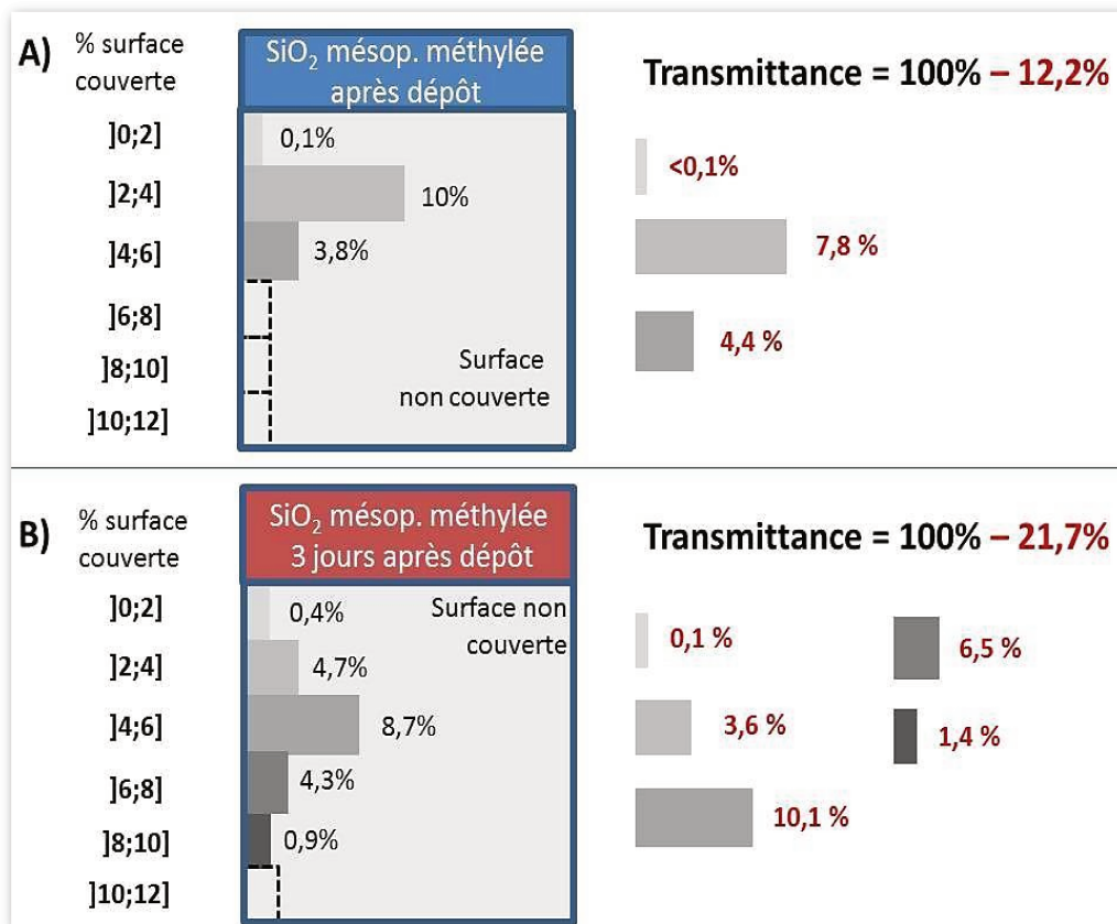
Figure V.37 : calculs de diffusion à t = 60 s pour une couche mince mésoporeuse de \text{SiO}_2 méthylée après dépôt (A) et 3 jours après dépôt (B). Les valeurs de surfaces couvertes par chaque type de gouttes sont indiquées sur la gauche. La perte de transmission par diffusion est présentée à droite avec la contribution de chaque famille de gouttes.
