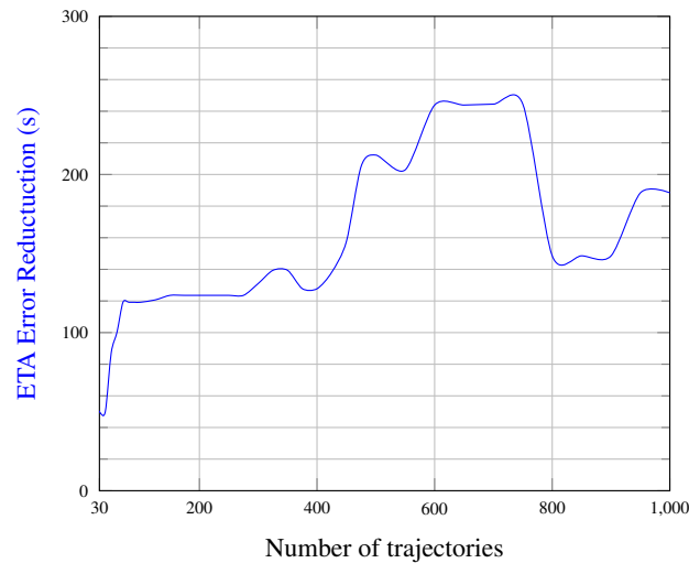
Figure 4.28 – \Delta ETA_{true/pred} - \Delta ETA_{true/up}
