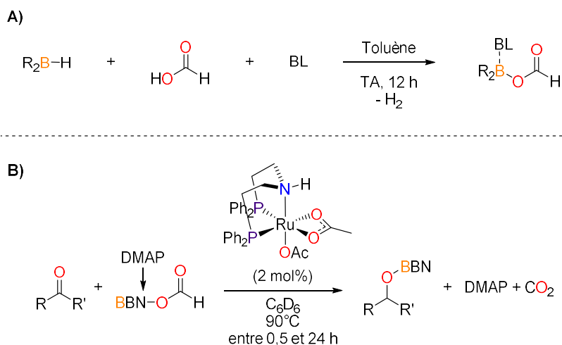
Figure IV-8 : A) Voie de synthèse d'un mono formiate de bore neutre. B) Hydroboration par transfert des aldéhydes et des cétones par un mono formiate de bore neutre, catalysée au ruthénium. BL = base de Lewis
