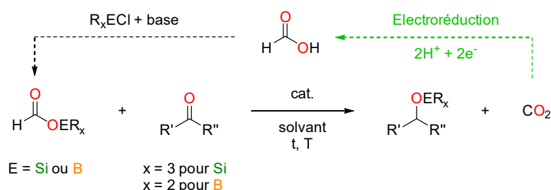
Figure IV-2 : Illustration de la recyclabilité du CO 2 pour l'utilisation des formiates de bore et de silicium.
