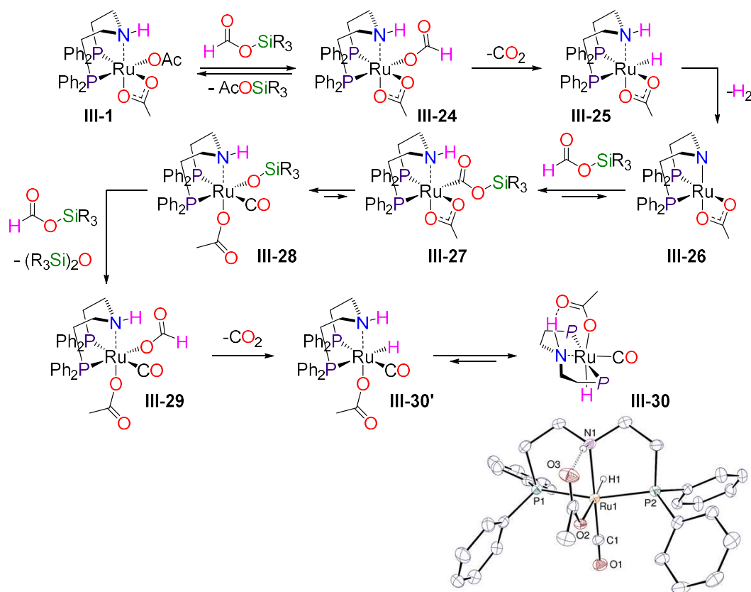
Figure II-54 : Equilibre thermodynamique entre [Ru(OAc) 2 (PN H P Ph )] ( III-1 ) et [Ru(H)(CO)(PN H P Ph )] ( III-30 )
