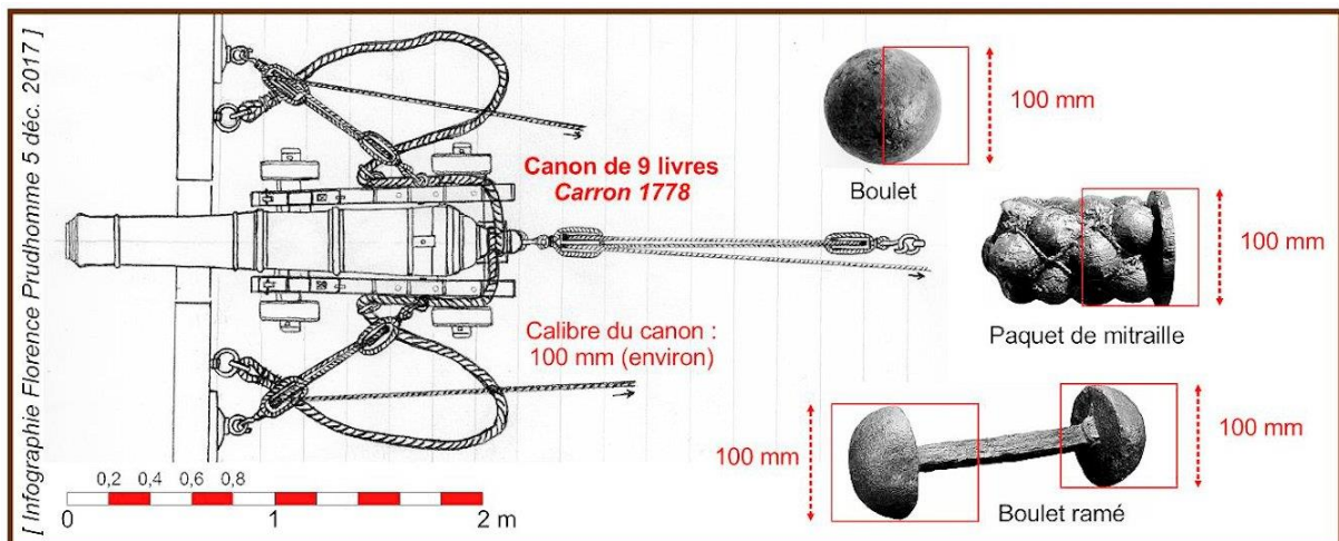
Fig. C2-009. Pièce de 9 livres et ses munitions.
