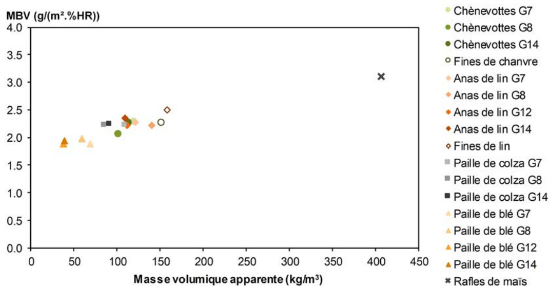
FIGURE 3.20 – Capacité tampon hygrique des granulats en fonction de leur masse volumique apparente.
