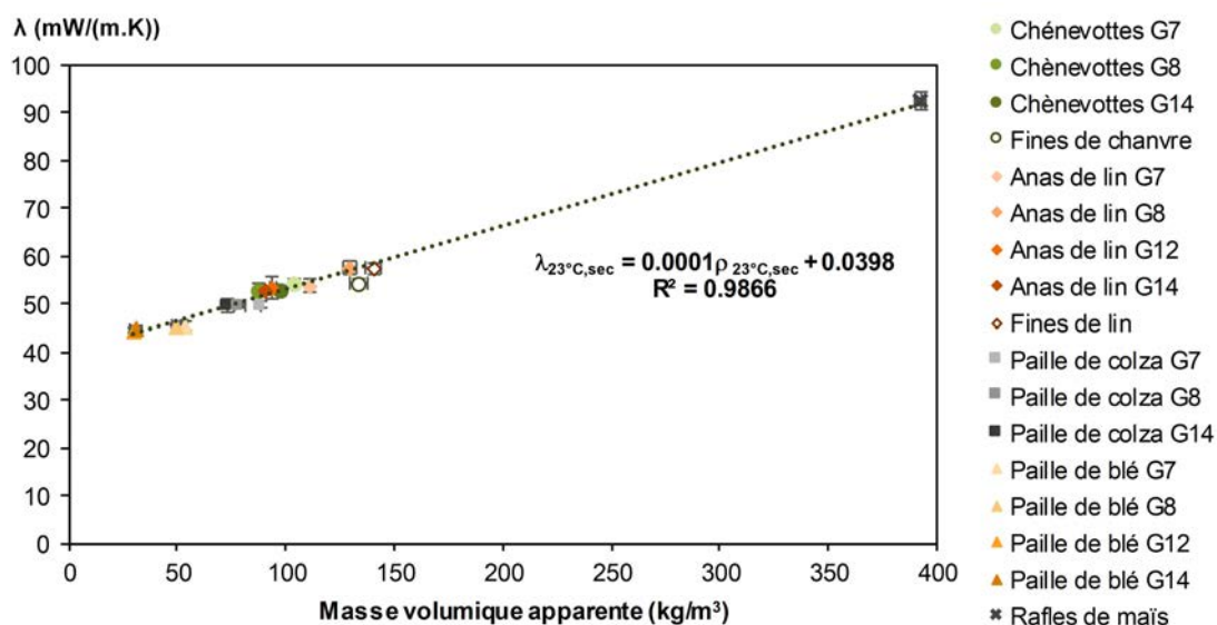
FIGURE 3.18 – Conductivité thermique des granulats en fonction de leur masse volumique apparente.
