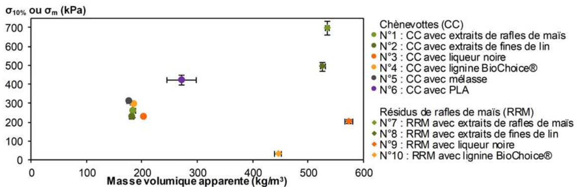
FIGURE 5.4 – Contrainte à 10 % de déformation ou contrainte maximale versus masse volumique apparente des composites à (23°C; 50 %HR).
