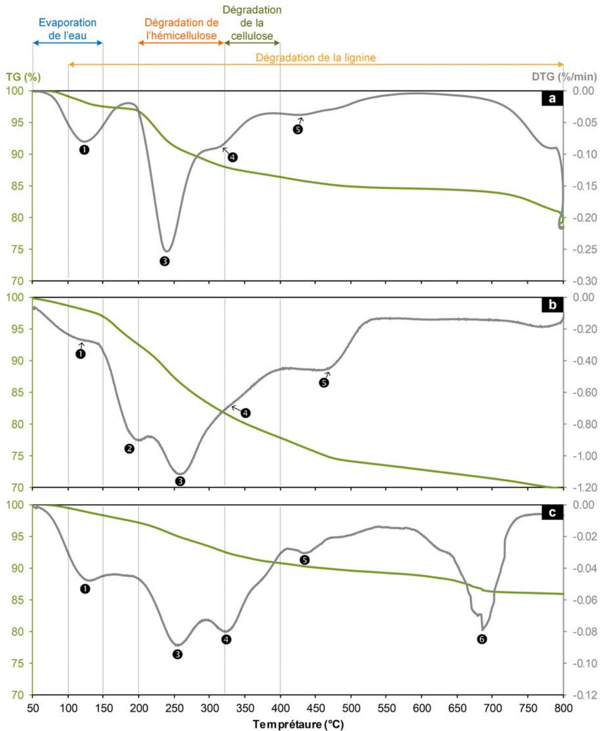
FIGURE 4.13 – Courbes TG (variation de masse) et DTG (dérivée de la variation de masse) des extraits issus : (a) des rafles de maïs avec une solution de soude à 2.5 %, (b) des rafles de maïs avec une solution de silicate de sodium à 5 % et (c) des fines de lin avec une solution de silicate de sodium à 5 %.
