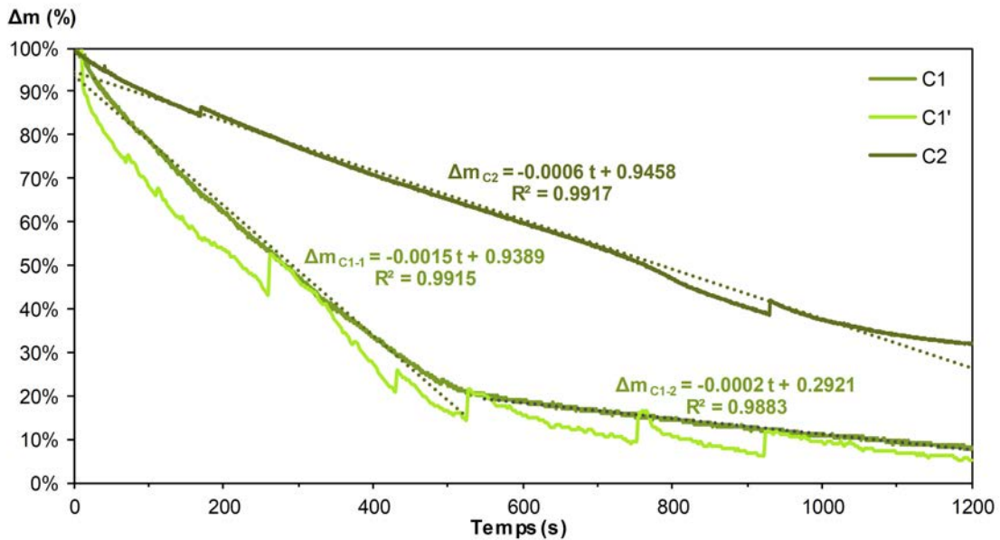
FIGURE 6.11 – Perte de masse des échantillons en fonction du temps lors du test avec le cône calorimètre.
