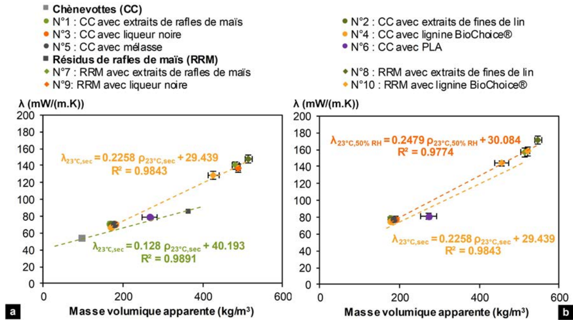
FIGURE 5.7 – Conductivité thermique des composites et des granulats versus leur masse volumique apparente à : (a) (23°C; point sec) et (b) (23°C; 50 %HR).
