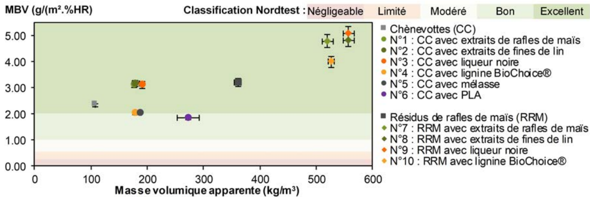
FIGURE 5.12 – Valeur MBV (g/(m 2 .%HR)) moyenne des composites fabriqués versus leur masse volumique apparente.
