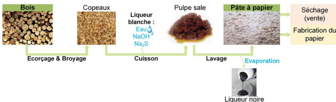
FIGURE 4.16 – Procédé de fabrication de la pâte à papier.
