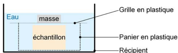
FIGURE 2.16 – Dispositif expérimental de l'essai d'immersion accidentelle.
