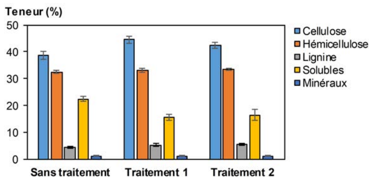
FIGURE 4.3 – Composition chimique de la paille de blé avant et après les traitements hydrothermiques : (1) infusion à 80°C et (2) infusion à 80°C puis cuisson à 180 °C.
