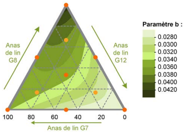
FIGURE 3.24 – Surface de réponse du paramètre b du modèle de Jones pour une pression de compression comprise entre 0.0637 et 0.2546 MPa en fonction de la distribution granulométrique des anas de lin.
