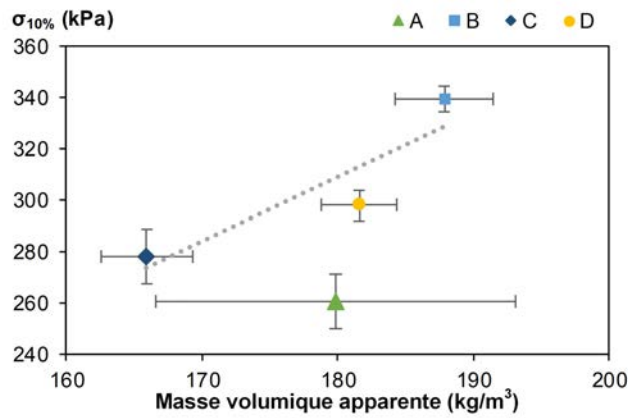
FIGURE 4.6 – Contrainte à 10 % de déformation versus la masse volumique apparente à (23°C; 50 %HR) des composites.
