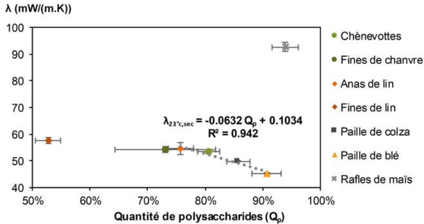
FIGURE 3.26 – Conductivité thermique en fonction de la quantité de polysaccharides (cellulose, hémicellulose et pectine) contenue dans les agro-ressources.
