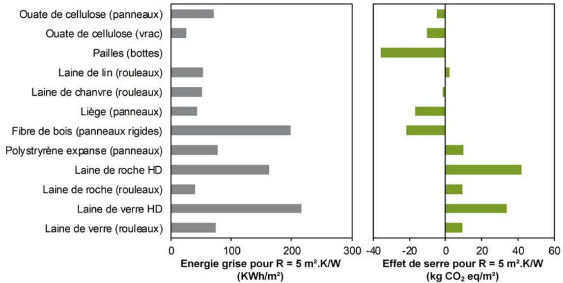
FIGURE 1.5 – Énergie grise et bilan de la production de CO 2 de différents isolants pour une résistance thermique R équivalente à 5 m 2 .K/W (TECHNIQUE DE L'INGÉNIEUR [2012]).
