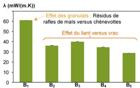
FIGURE 5.9 – Diagramme à barres pour la conductivité thermique au point sec (mW.(m.K)).
