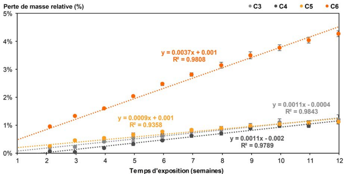
FIGURE 6.6 – Perte de masse des composites testés lors de l'essai de vieillissement.
