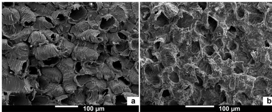
FIGURE 4.15 – Micrographies MEB des rafles de maïs avant et après l'extraction des solubles avec une solution de silicate de sodium à 5 %.
