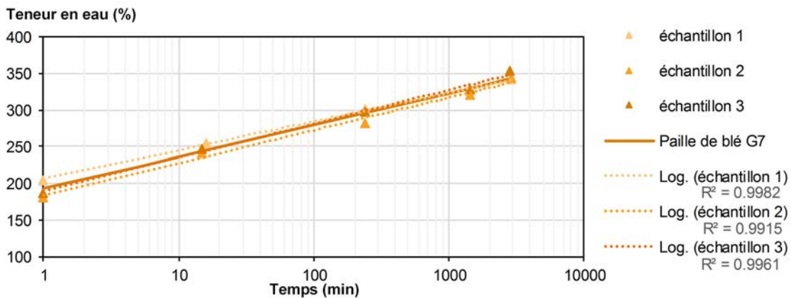
FIGURE 3.15 – Absorption d'eau de la paille de blé G7 - données expérimentales, courbes d'ajustement et courbe caractéristique.
