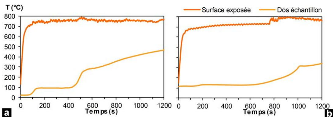
FIGURE 6.12 – Température en fonction du temps de la surface exposée au feu ainsi que du dos des échantillons : (a) C1 et (b) C2.
