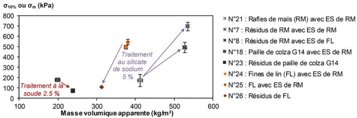
FIGURE 5.25 – Contrainte à 10 % de déformation ou contrainte maximale versus masse volumique apparente des composites à (23°C; 50 %HR).
