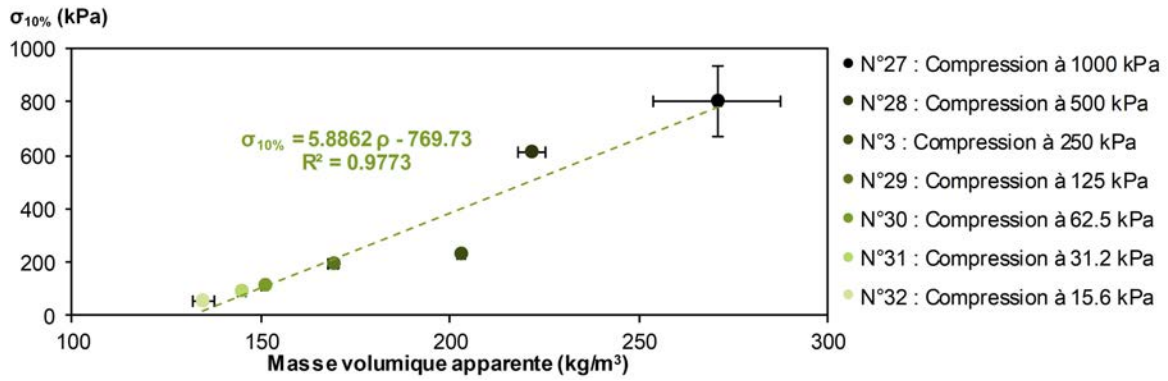
FIGURE 5.30 – Contrainte à 10 % de déformation des composites fabriqués versus leur masse volumique apparente.
