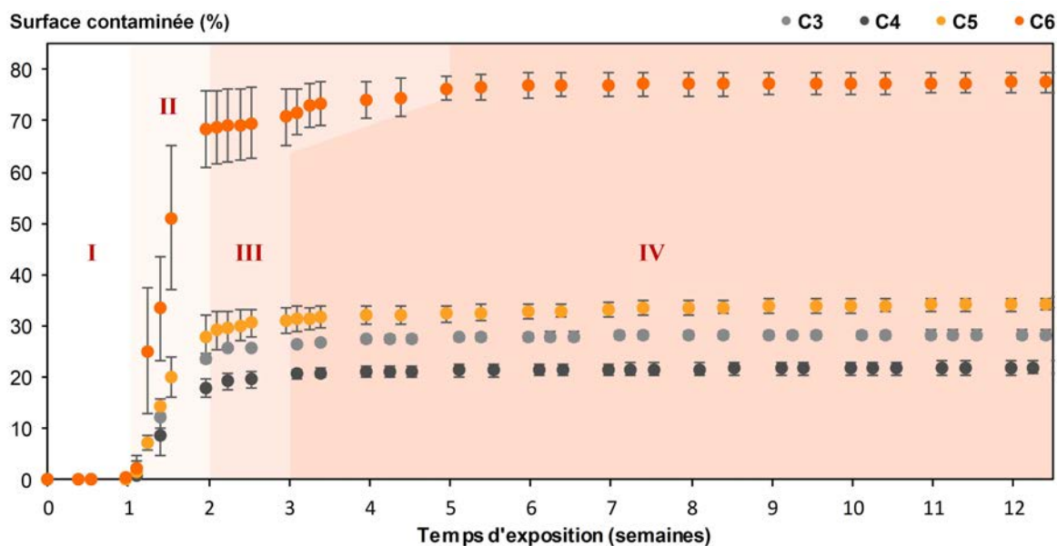
FIGURE 6.8 – Analyse d'images : évaluation de la surface contaminée de composites C3, C4, C5 et C6 exposés à 30°C et 90 % d'humidité relative pendant la période d'essai, corrélés aux phases de croissance fongique avec I : Phase de latence, II : Phase exponentielle, III : Phase de ralentissement et IV : Phase stationnaire.
