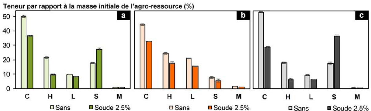
FIGURE 4.11 – Composition chimique des chènevottes (a), des anas de lin (b) et de la paille de colza (c) avant et après les extractions à la soude à 5% (C : Cellulose, H : Hémicellulose, L : Lignine, S : Solubles et M : Minéraux).
