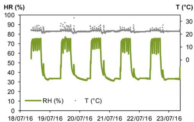
FIGURE 5.10 – Relevé de l'humidité relative et de la température dans l'enceinte climatique pendant le test MBV.
