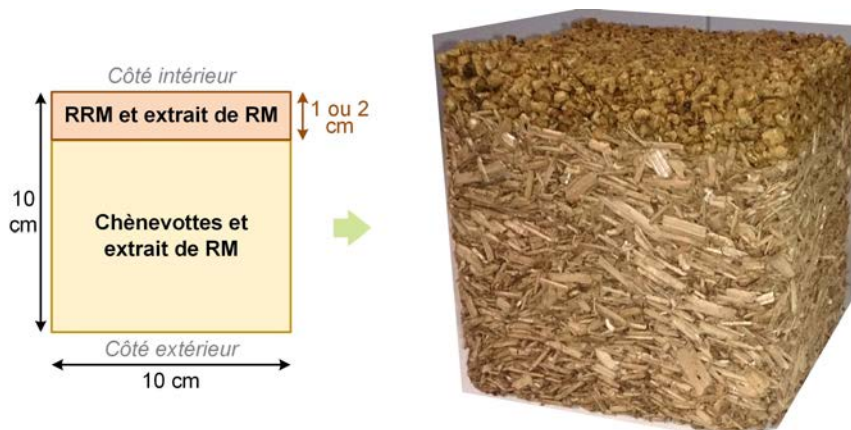
FIGURE 5.34 – Composite bi-couche lié avec de l'extrait de rafles de maïs (RM) et dont la première couche de 8 ou 9 cm, est composée de chènevottes et la deuxième de 1 ou 2 cm, est composée de résidus de rafles de maïs (RRM).
