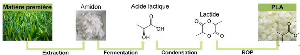
FIGURE 4.19 – Procédé de fabrication du PLA (ROP : Ring Opening Polymerization).
