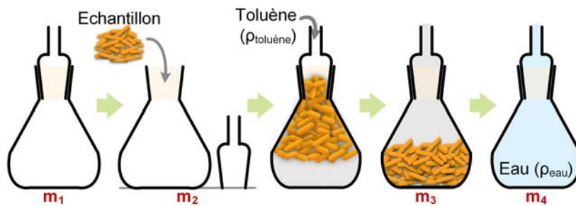
FIGURE 2.9 – Protocole de mesure de la masse volumique du squelette.
