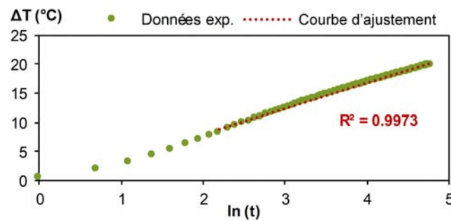
FIGURE 5.6 – Exemple d'augmentation de la température par rapport au logarithme népérien du temps.
