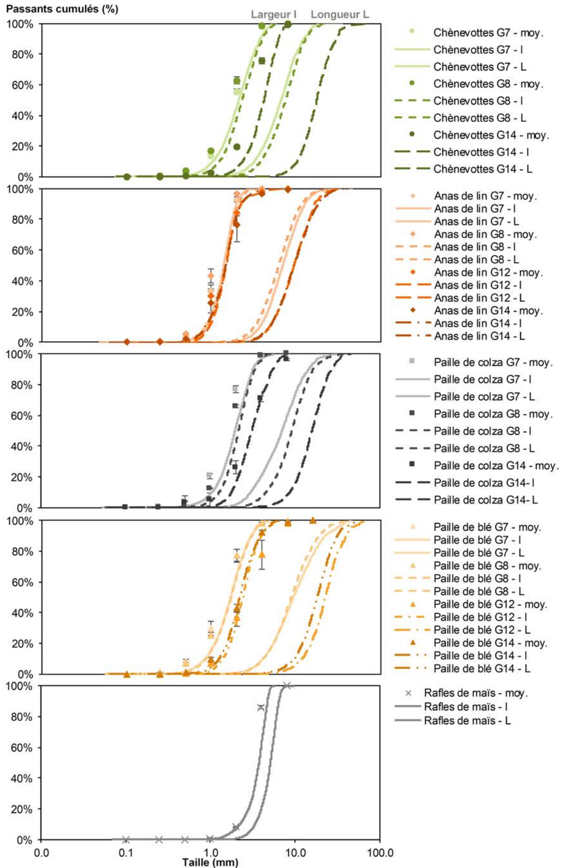
FIGURE 3.10 – Distribution granulométrique (PSD) des chènevottes, anas de lin, paille de colza, paille de blé et rafles de maïs - tamisage mécanique (moyenne et écart-type) et analyse d'image (l : largeur et L : longueur).
