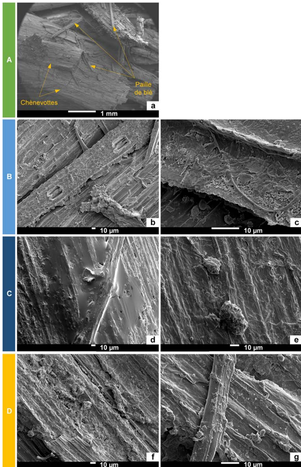
FIGURE 4.5 – Micrographies MEB de l'interface entre les chènevottes et le liant : (a) composite A, (b) et (c) composite B, (d) et (e) composite C ainsi que (f) et (g) composite D.
