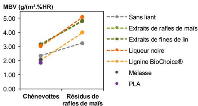
FIGURE 5.13 – Diagramme des interactions pour la valeur tampon hygrique (g/(m 2 .%HR)).
