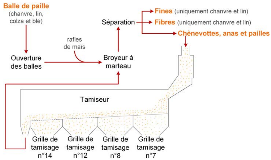
FIGURE 3.2 – Schéma du process de préparation des agro-ressources.
