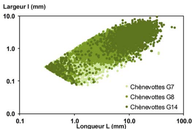
FIGURE 3.9 – Données brutes provenant de l'analyse d'images des chènevottes.
