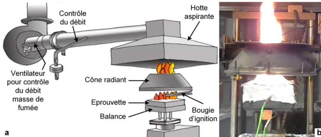
FIGURE 2.22 – (a) Schéma d'un cône calorimètre (MARQUIS et al [2009]) - (b) Cône calorimètre Atlas en fonctionnement.
