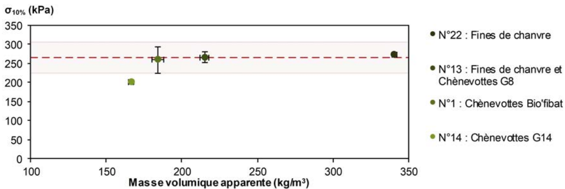
FIGURE 5.20 – Contrainte à 10 % de déformation ou contrainte maximale versus masse volumique apparente des composites à (23°C; 50 %HR).
