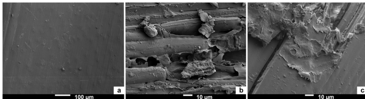
FIGURE 4.4 – Micrographies MEB de la surface de la paille de blé : (a) sans traitement, (b) et (c) après le traitement hydrothermique 2.
