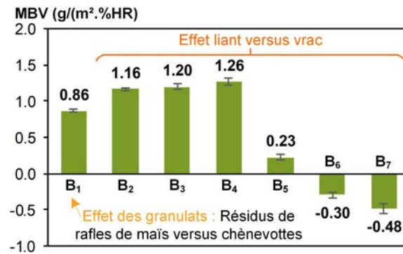
FIGURE 5.14 – Diagramme à barres pour la valeur tampon hygrique ( \text{g}/(\text{m}^2.\%HR) ).
