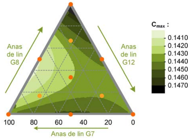
FIGURE 3.22 – Surface de réponse de la compacité maximale ( C_{max} ) des anas de lin en fonction de leur distribution granulométrique.
