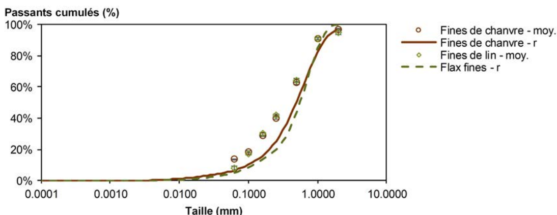
FIGURE 3.12 – PSD des fines - tamisage mécanique (moyenne et écart-type) et granulométrie à diffraction laser (r : rayon).
