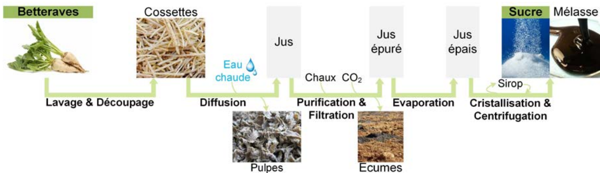
FIGURE 4.18 – Procédé de fabrication du sucre.
