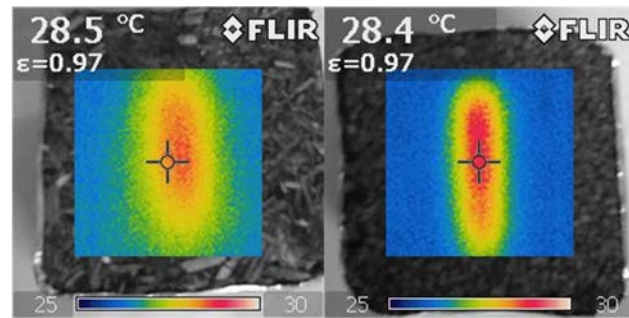
FIGURE 5.5 – Photos de thermographie infrarouge des échantillons n°5 (à gauche, chènevottes collées avec de la mélasse) et n°8 (à droite, résidus de rafles de maïs collés avec de l'extrait de fines de lin) immédiatement après la mesure de la conductivité thermique.
