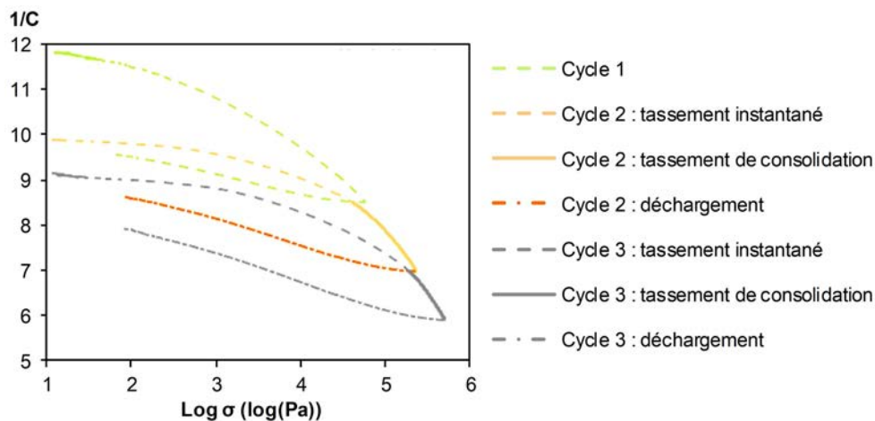
FIGURE 3.21 – Division des courbes de tassement pour l'identification des modèles pour un mélange entièrement constitué d'anas de lin G7.
