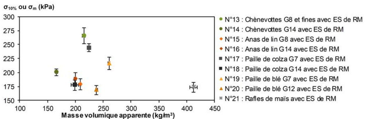
FIGURE 5.16 – Contrainte à 10 % de déformation ou contrainte maximale versus masse volumique apparente des composites à (23°C; 50 %HR) (ES de RM : Extrait de rafles de maïs).
