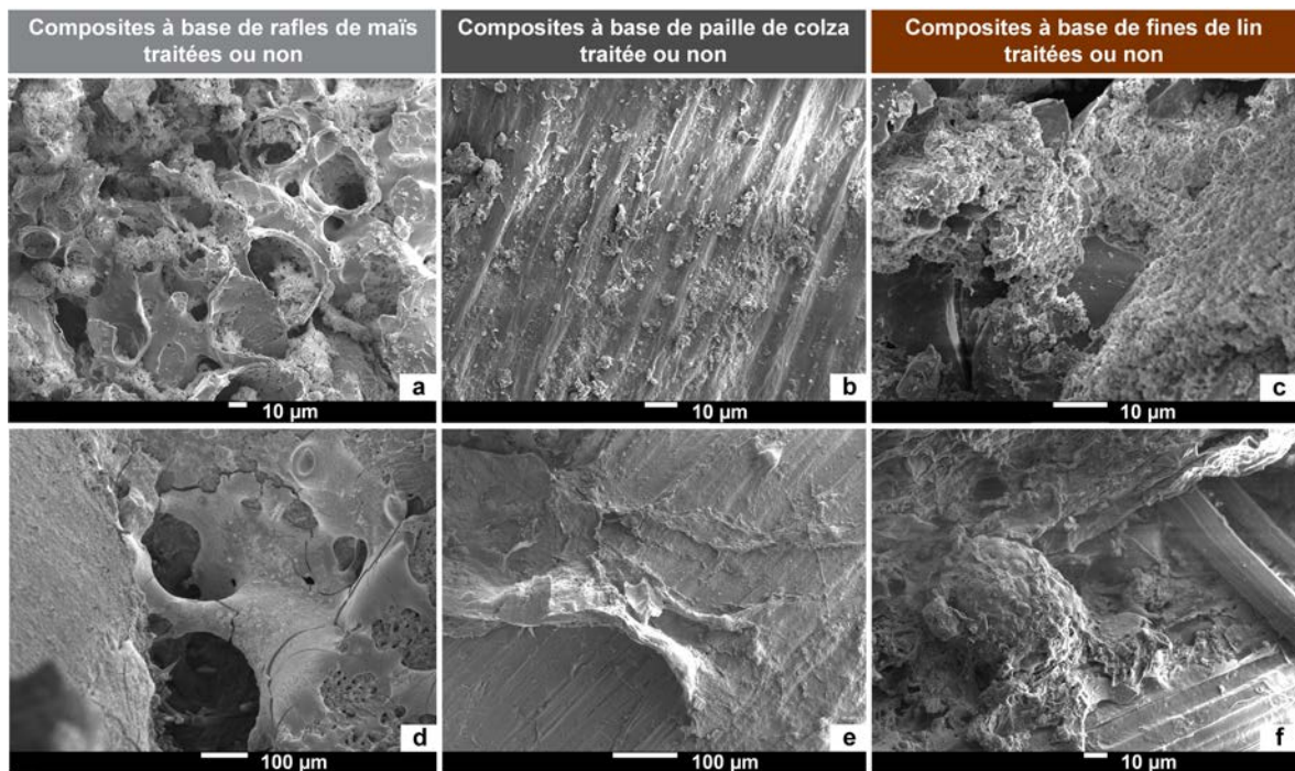
FIGURE 5.24 – Micrographies MEB des composites avec et sans traitement : (a) composite à base de rafles de maïs et d'extrait de rafles de maïs, (b) composite à base de paille de colza et d'extrait de rafles de maïs, (c) composite à base de fines de lin et d'extrait de rafles de maïs, (d) composite à base de résidus de rafles de maïs et d'extrait de rafles de maïs (e) composite à base de résidus de paille de colza et (f) composite à base de résidus de fines de lin.
