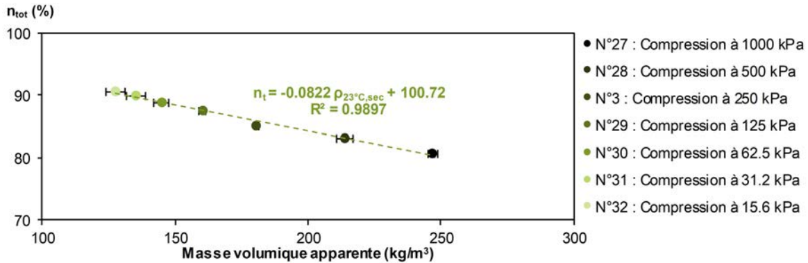
FIGURE 5.29 – Porosité totale des composites fabriqués versus leur masse volumique apparente à (23°C; point sec).
