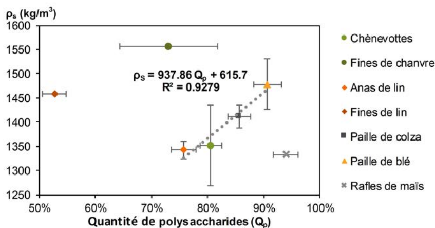
FIGURE 3.25 – Masse volumique du squelette en fonction de la quantité de polysaccharides (cellulose, hémicellulose et pectine) contenue dans les agro-ressources.
