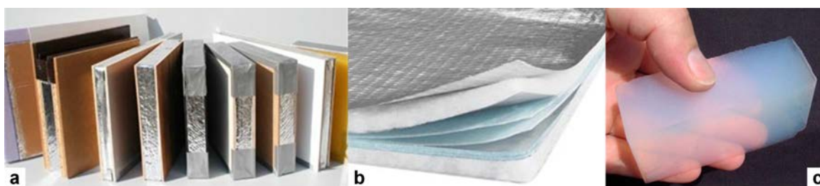
FIGURE 1.10 – Isolants nouvelle génération : (a) Panneaux sous vide, (b) Panneau réfléchissant et (c) Aérogel.
