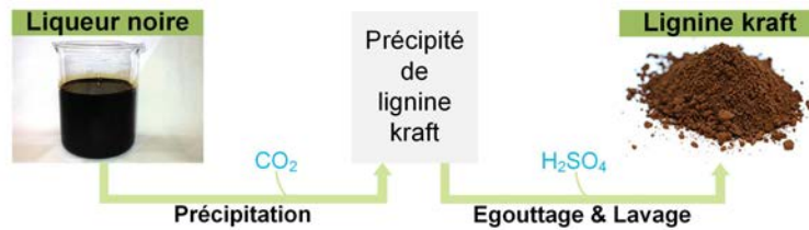
FIGURE 4.17 – Procédé de fabrication de la lignine kraft à partir de la liqueur noire.
