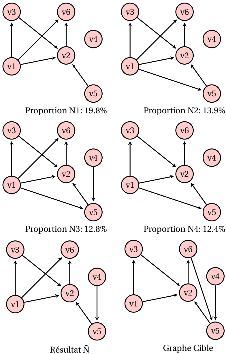
FIGURE 4.10 – Principaux graphes obtenus par la méthode. Nous notons la proportion obtenue dans l'échantillon final des principaux graphes. La référence est donnée par le dernier graphe. Le graphe "Résultat" est le graphe moyen, puis seuillé.
