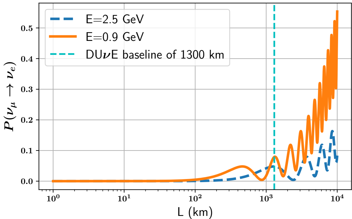
FIGURE 1.3 – P(\nu_\mu \rightarrow \nu_e) en fonction de L pour un neutrino de 0,9 GeV et 2,5 GeV. La ligne verticale représente la ligne de base de \text{DU}\nu\text{E} . Le faisceau de neutrino envoyé aura des énergies allant de 0,5 GeV et 5 GeV, incluant donc les deux premiers maxima locaux de probabilité.
