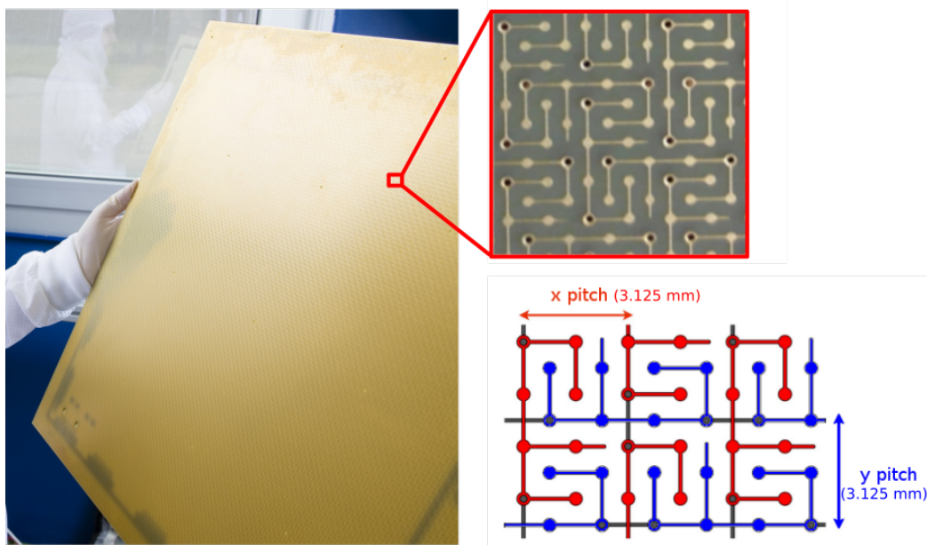
FIGURE 3.15 – Photo et schéma d’une anode de 50 \times 50 \text{ cm}^2 . Le design vient des études du prototype de 3 L[11, 5] et permet un partage égal de la charge entre les deux vues tout en minimisant la capacitance.
