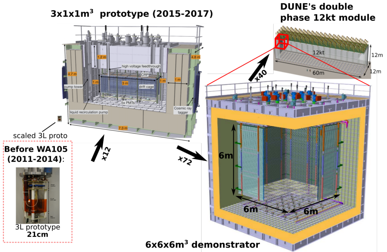
FIGURE 3.2 – WA105 et sa place dans le développement de la technologie DArTPC.
