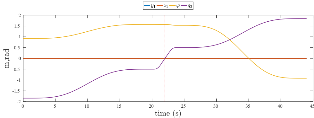
FIGURE 5.8 – Trajectoire pour la traversée de la singularité pour les coordonnées \mathbf{q}_p . La barre verticale rouge indique la traversée de la singularité.
