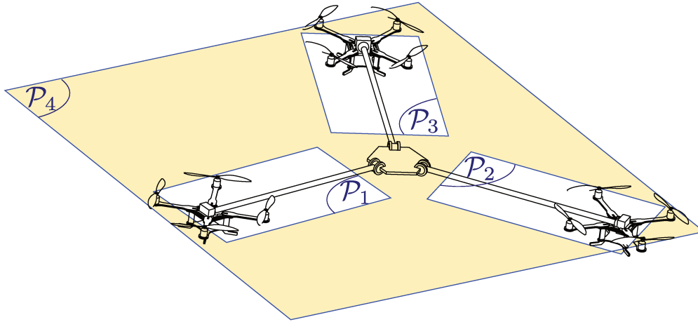
FIGURE 3.4 – Exemple d’une configuration singulière pour le robot parallèle volant à trois drones. \mathcal{P}_1 , \mathcal{P}_2 , \mathcal{P}_3 et \mathcal{P}_4 sont coplanaires.
