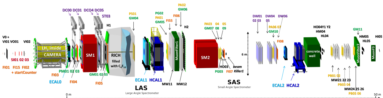
Figure 81: Schéma de principe de l'expérience COMPASS pour 2016 et 2017.
