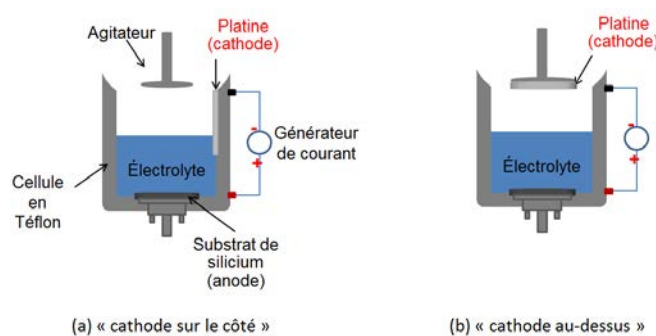
FIGURE 4.6 – Schéma de la cellule d'anodisation électrochimique en configuration (a) "cathode sur le côté" et "cathode au-dessus".
