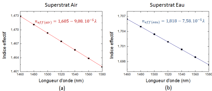
FIGURE 4.30 – Indices effectifs de guide d’onde Superstrat/50/80/Si de dimensions 2 \mu\text{m} \times 1,5 \mu\text{m} pour les superstrats : air et eau désionisée.
