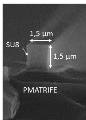
FIGURE 3.19 – Image MEB de la vue en coupe d'un guide d'onde ridge Air/SU8/PMATRIFE/Si.
