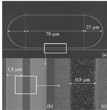
FIGURE 4.25 – Images MEB du micro-résonateur en forme d’hippodrome : vues de dessus à différents grossissements : (a) L’ensemble du micro-résonateur de rayon égal à 25 \mu\text{m} et de longueur de couplage égale à 70 \mu\text{m} , (b) et (c) la zone de couplage.
