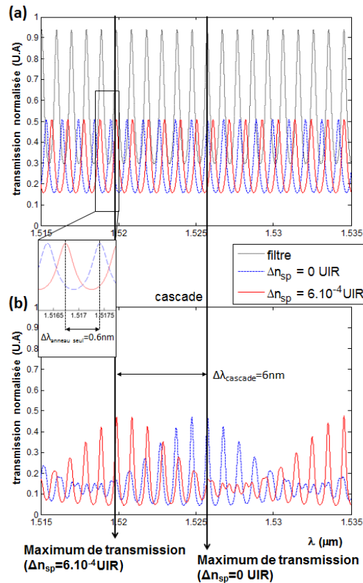
FIGURE 1.16 – Principe de l'effet Vernier : (a) Transmissions normalisées pour les micro-résonateurs de référence et de détection et (b) Transmissions normalisées du système cascade. Un décalage est représenté pour une valeur arbitraire de \Delta n_{sp} .
