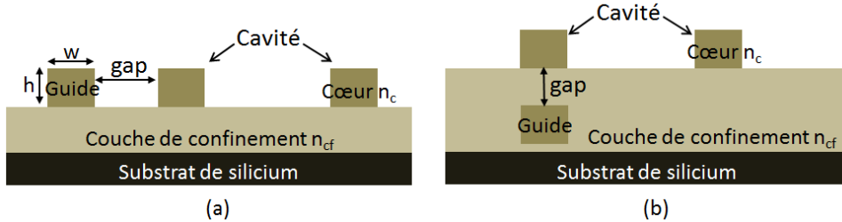
FIGURE 1.12 – Différents types de couplage : (a) Couplage horizontal; (b) Couplage vertical pour un micro-résonateur couplé à un seul guide.
