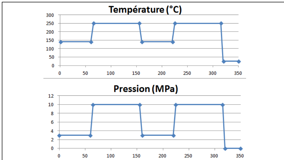
Figure 4.3 : Profils de sollicitation lors du report de l'assemblage onduleur triphasé vertical-3D.
