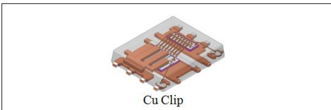
Figure 1.10 : Assemblage par clip brasé Cu. [44]
