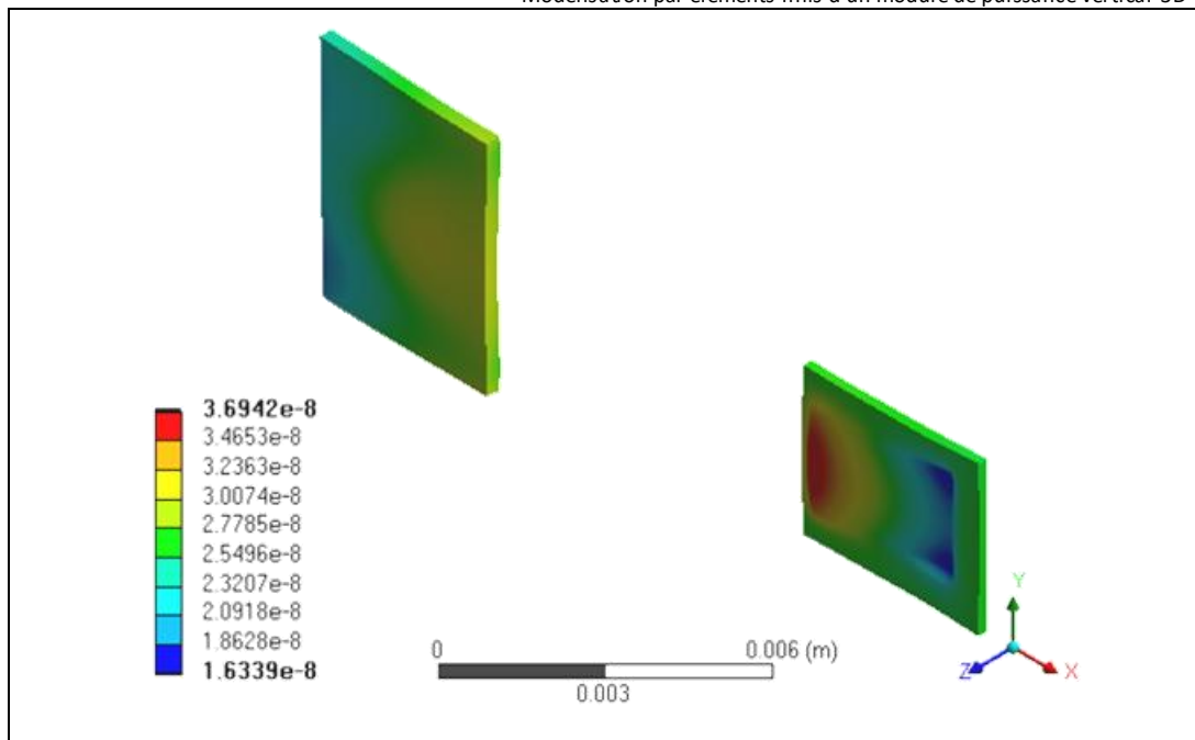
Figure 4.4 : Cartographie des déformations totales dans les puces de l'assemblage onduleur triphasé vertical-3D après report.
