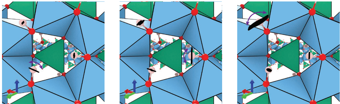
(a) Bending A . 114 – 121 meV avec s = 5 .
