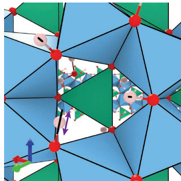
(d) Stretching A . 457 – 461 meV avec s = 20 .
