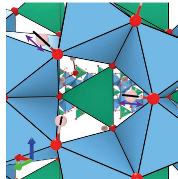
(e) Stretching B and C . 465 – 470 meV avec s = 20 .
