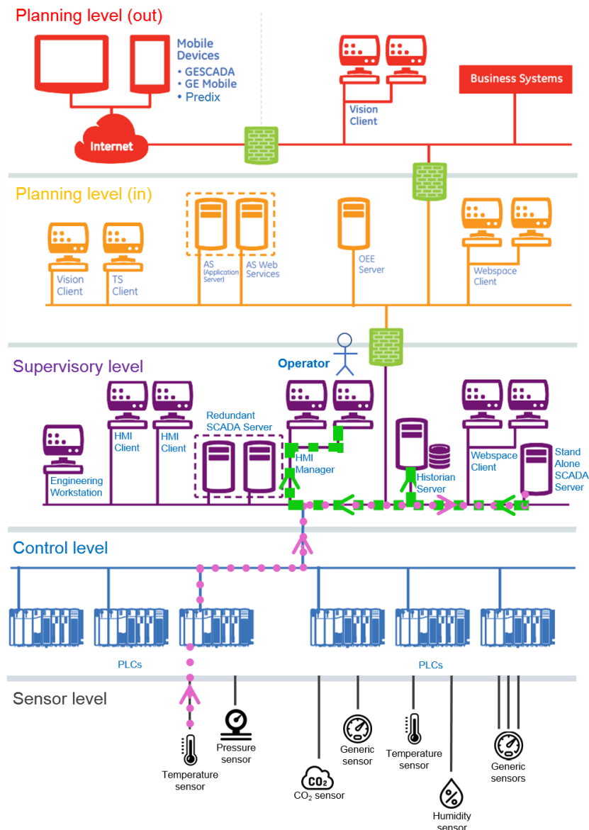
Figure 2 : Architecture type d'un système moderne de contrôle et de supervision (source GE)
