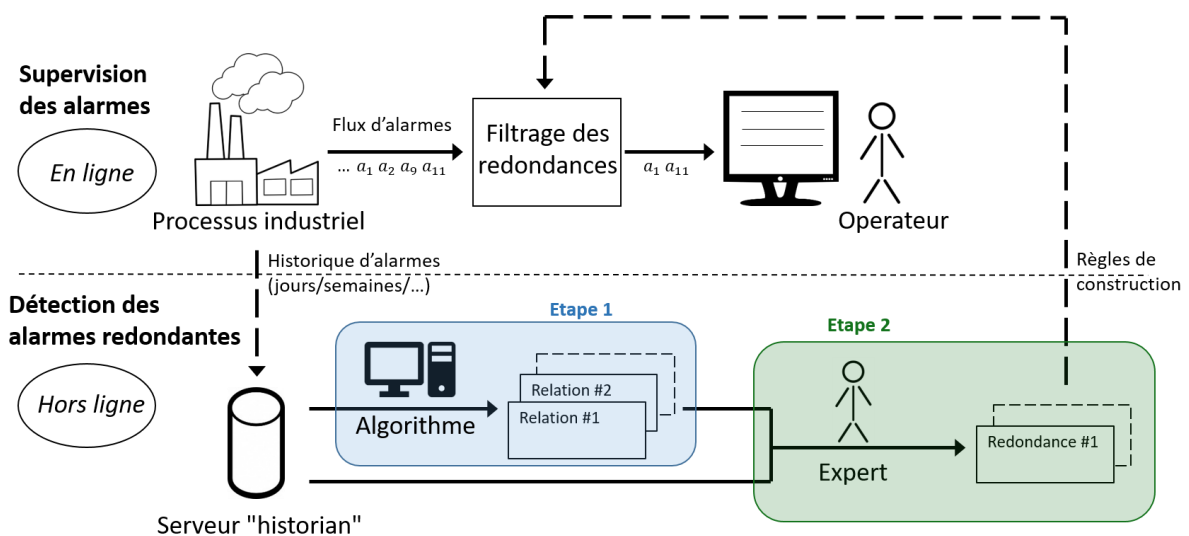
Figure 10 : Schéma détaillant l'approche proposée
