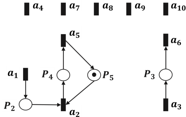
Figure 37 : Réseau de Petri identifié dans l'exemple de la chaudière
