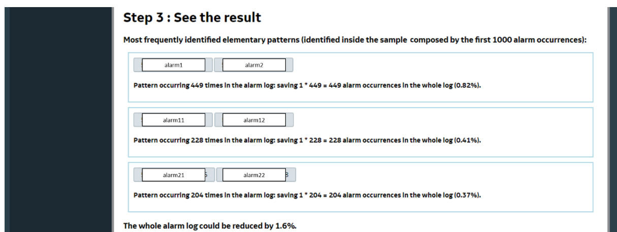
Figure 32 : Résultats de la recherche limitée de séquences fréquentes
