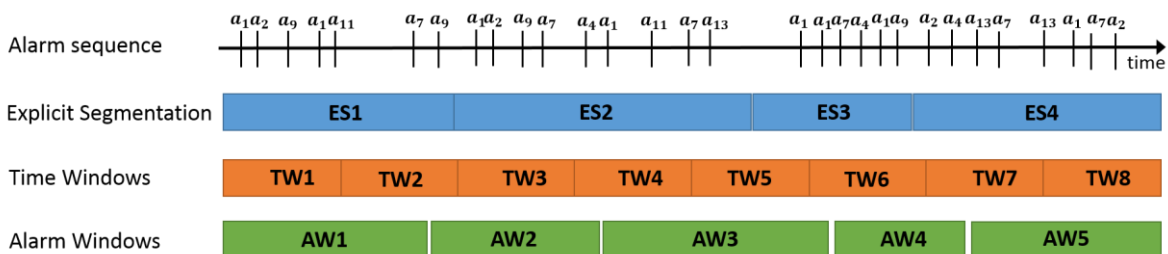
Figure 14 : Approches classiques pour fenêtrer une séquence (inspiré par (Krishnan, et al., 2014))
