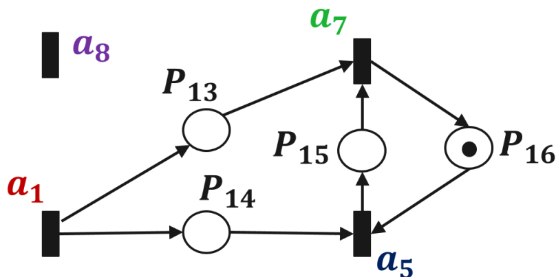
Figure 23 : Représentation complète des relations entre alarmes
