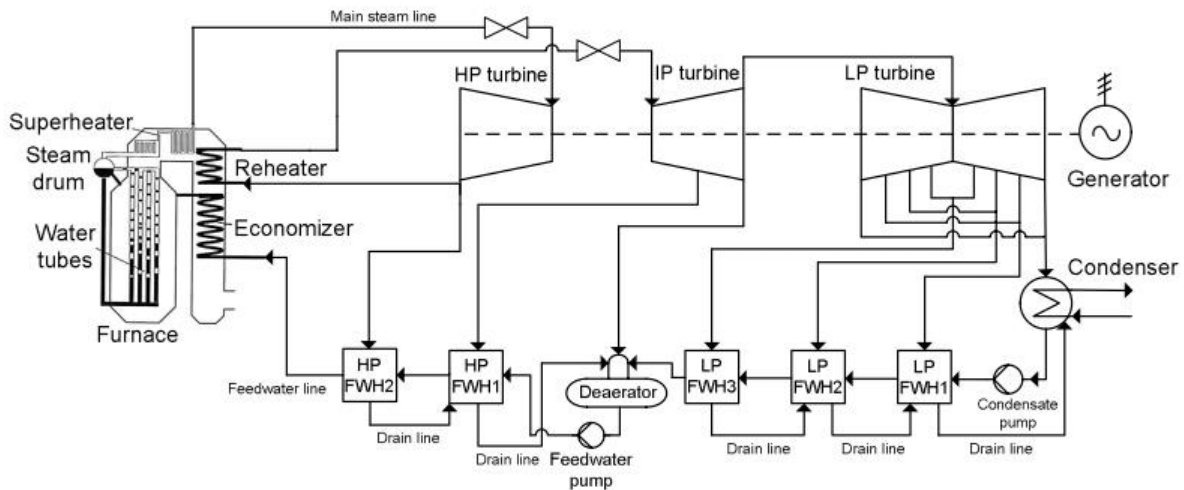
Figure 17 : Schéma représentant un système de production d'énergie (Mikkonen, et al., 2016)
