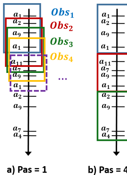
Figure 15 : Exemples de fenêtrage avec une fenêtre de longueur 4
