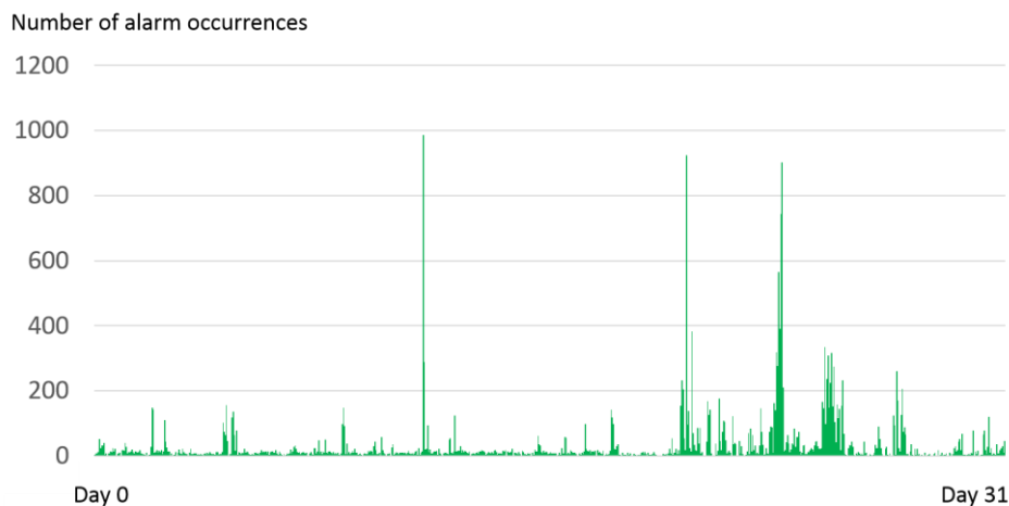
Figure 26 : Evolution du nombre d'occurrences d'alarmes durant le mois
