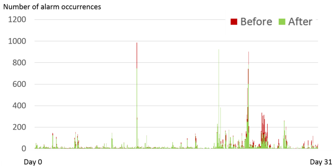
Figure 27 : Evolution du nombre d'occurrences d'alarmes durant le mois avant et après la réduction des séquences fréquentes
