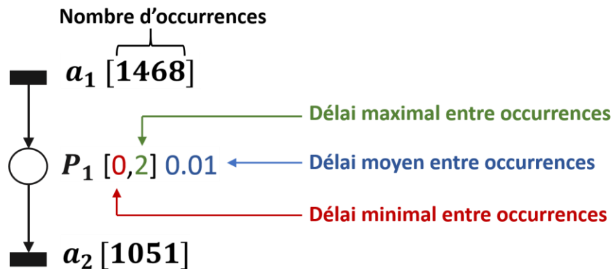
Figure 38 : Fragment avec informations utiles à l'expertise
