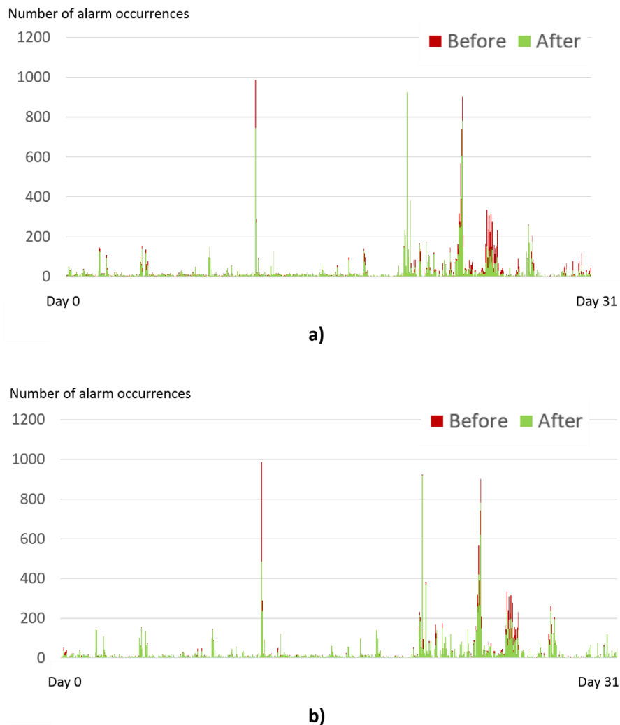
Figure 36 : Mise en parallèle des résultats des méthodes par recherche a) d'adjacences fréquentes et b) de précédences systématiques
