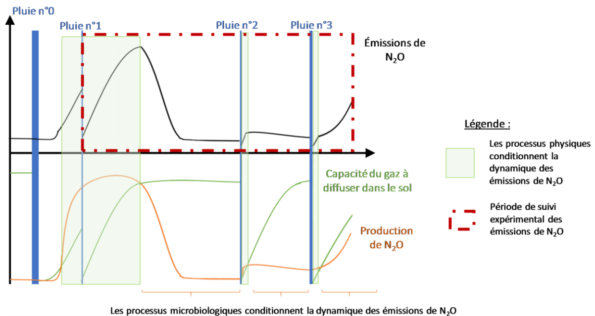
Figure 2-13 : Rôle des processus microbiologiques et physiques dans la dynamique des émissions de N 2 O : schéma explicatif de l'hypothèse proposée pour expliquer les observations lors du suivi expérimental.
