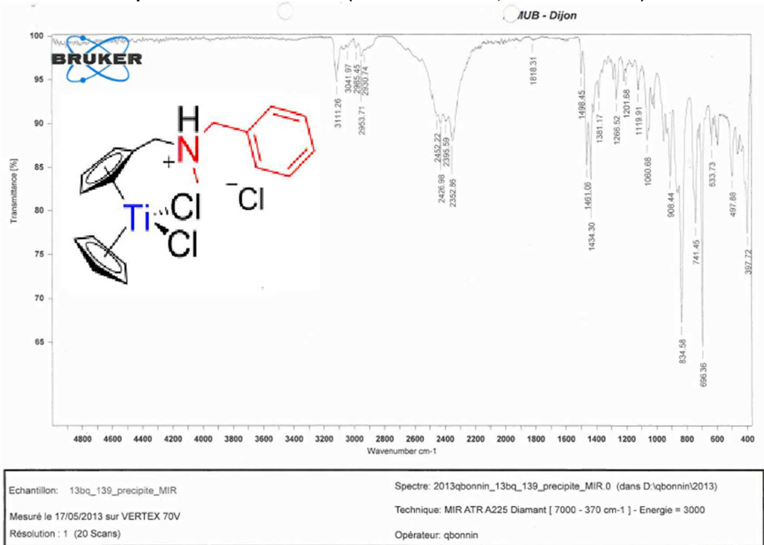
Spectrum 0-82: MIR of 14
