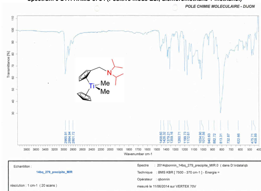
Spectrum 0-242: MIR of 34
