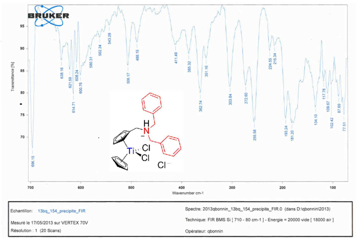
Spectrum 0-99: FIR of 16
