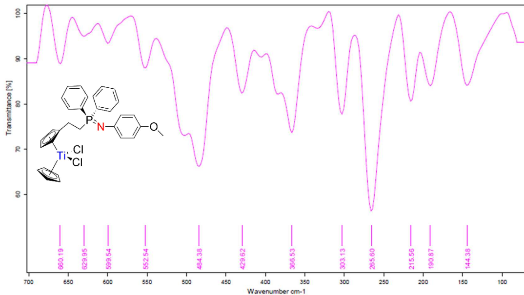
Spectrum 0-474: MIR of 57
