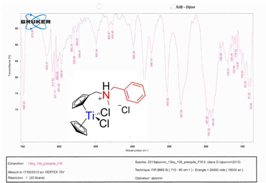
Spectrum 0-83: FIR of 14
