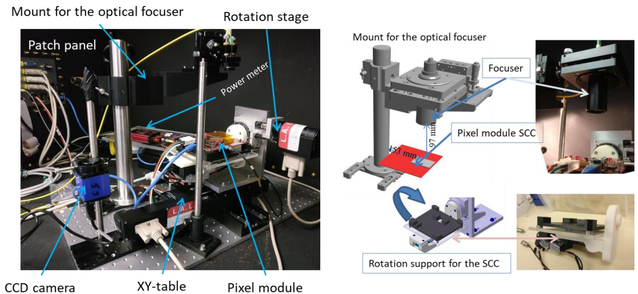
Figure 7 – a) Photo en salle blanche du banc de test laser. La carte SCC avec le module pixel, attachée au dispositif de rotation et l'ensemble monté sur la table de translation X-Y. Le portique à colonne maintient la focale. La caméra CCD bleue est fixée au même niveau que le module pixel pour la caractérisation faisceau. b) Embase et support du système de focalisation optique. La carte SCC et la distance du module à la lentille et au portique sont montrées. Embase et dispositif de maintien, en impression 3D plastique, de la carte SCC avec module pixel et scintillateur PMT.
