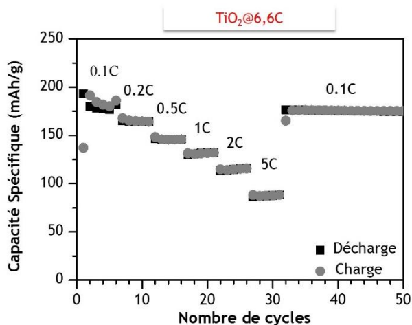
Figure A10 Capacité en puissance d'électrode à base de \text{TiO}_2@6,6\text{C} – capacité spécifique en fonction du nombre de cycles
