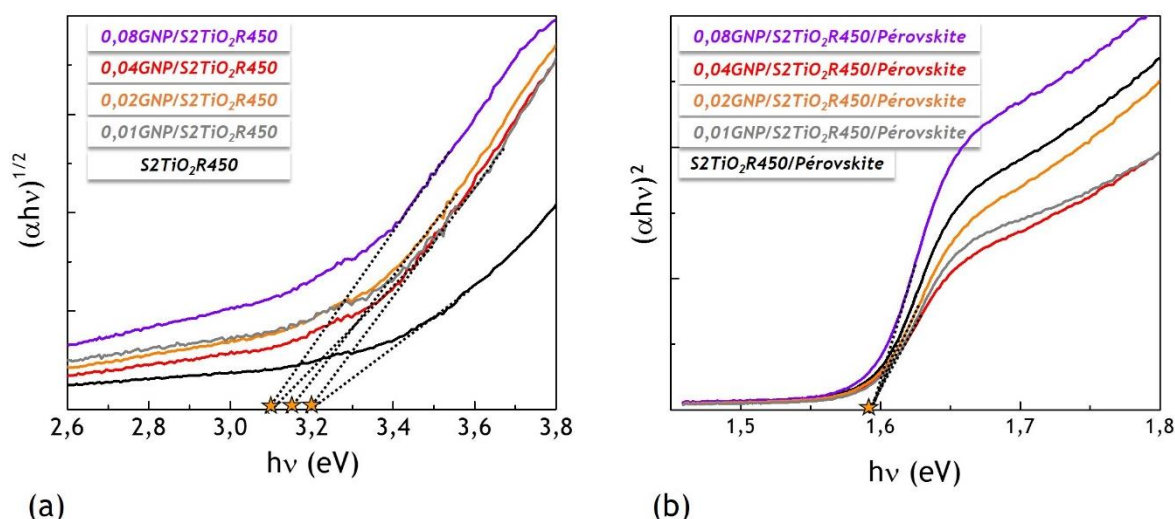
Figure IV-6 (a) « Tauc's plot » de l'absorption du TiO_2 pour la détermination du gap optique des couches mésoporeuses à base de TiO_2 et TiO_2 /graphène ( TiO_2 de référence S2TiO_2R450 et TiO_2 /GNP ( 0,01 - à 0,08GNP/S2TiO_2R450 )) (b) « Tauc's plot » pour la détermination du gap optique de la pérovskite déposée sur les couches à base de TiO_2 de référence S2TiO_2R450 et TiO_2 /GNP ( 0,01 - à 0,08GNP/S2TiO_2R450 )
